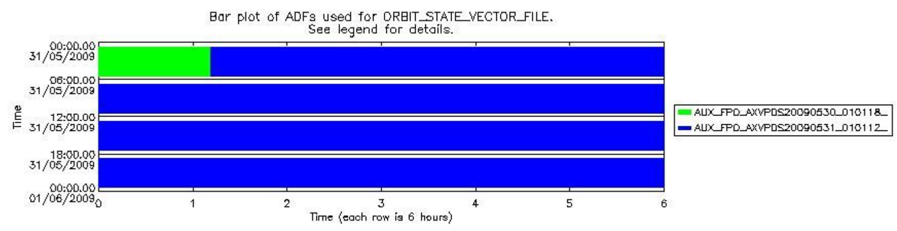
sciamachy_daily_report_level0_KSPT_L0_4303_N_20090531_8.PNG
