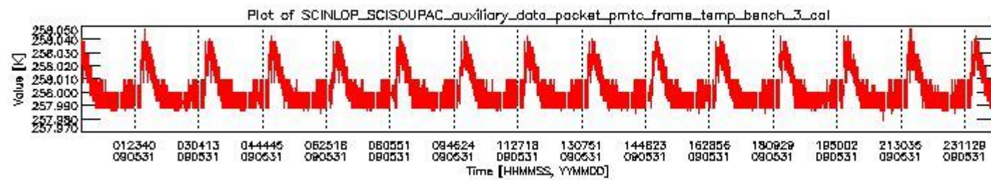
sciamachy_daily_report_level0_KSPT_L0_4303_N_20090531_2.PNG
