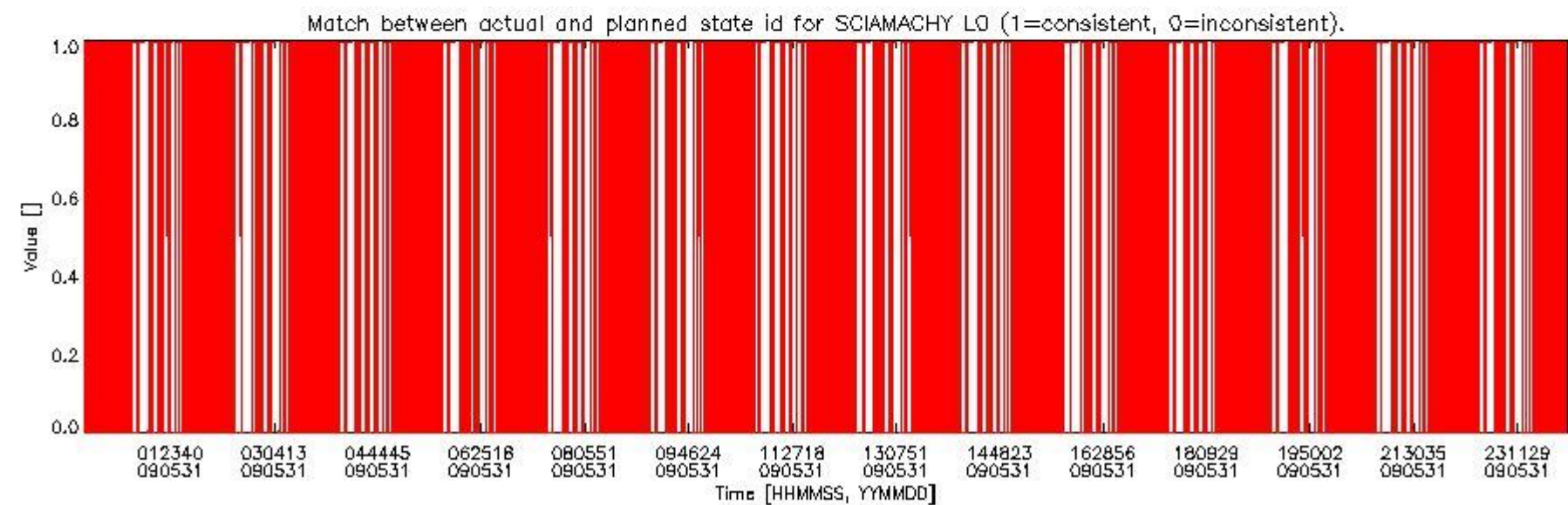
sciamachy_daily_report_level0_KSPT_L0_4303_N_20090531_5.PNG
