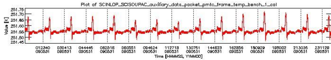
sciamachy_daily_report_level0_KSPT_L0_4303_N_20090531_0.PNG
