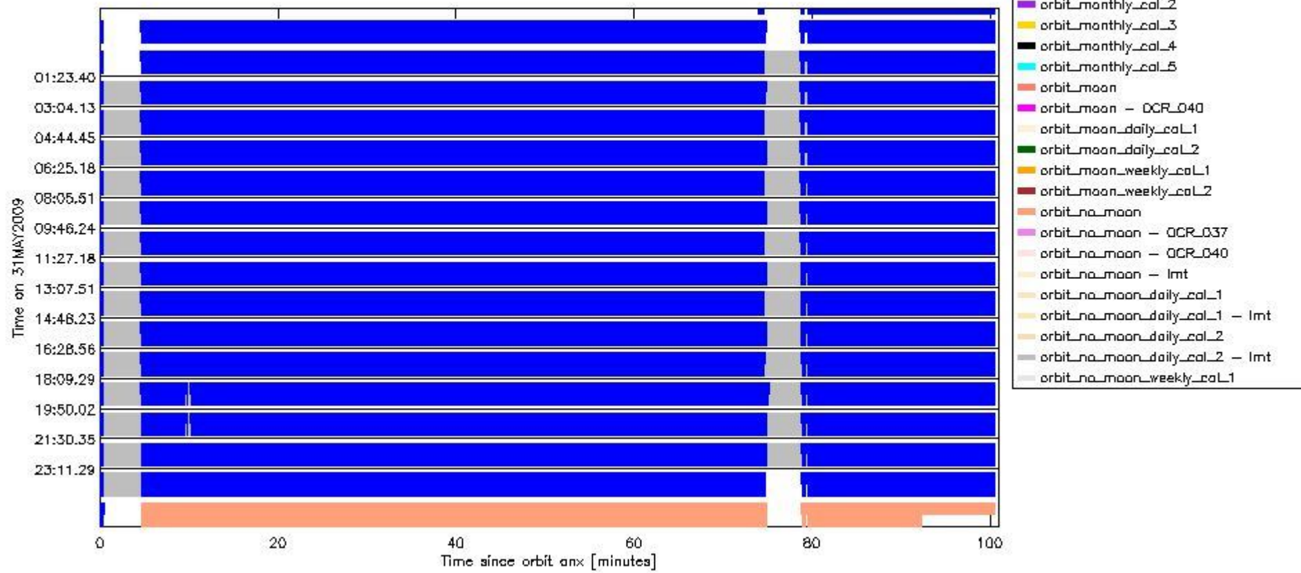
sciamachy_daily_report_level0_KSPT_L0_4303_N_20090531_6.PNG
