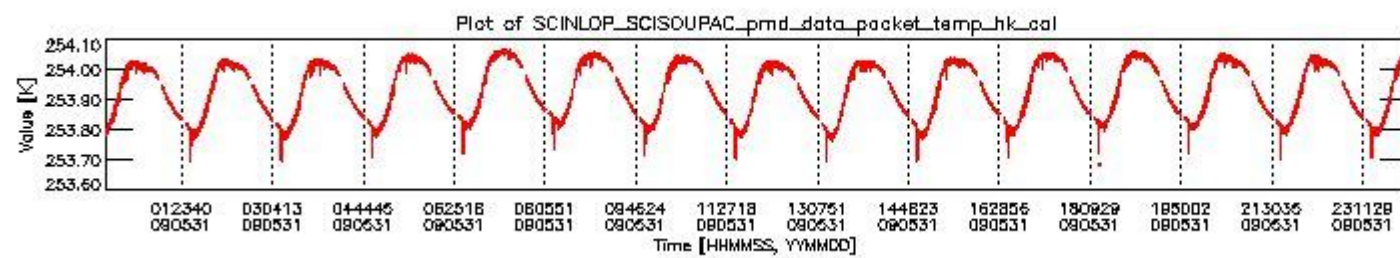
sciamachy_daily_report_level0_KSPT_L0_4303_N_20090531_3.PNG
