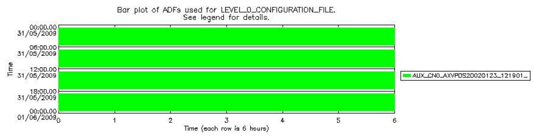
sciamachy_daily_report_level0_KSPT_L0_4303_N_20090531_7.PNG
