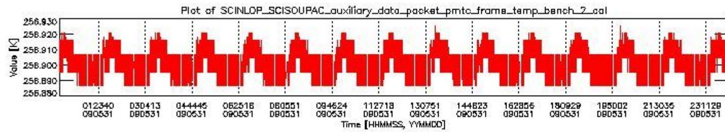
sciamachy_daily_report_level0_KSPT_L0_4303_N_20090531_1.PNG
