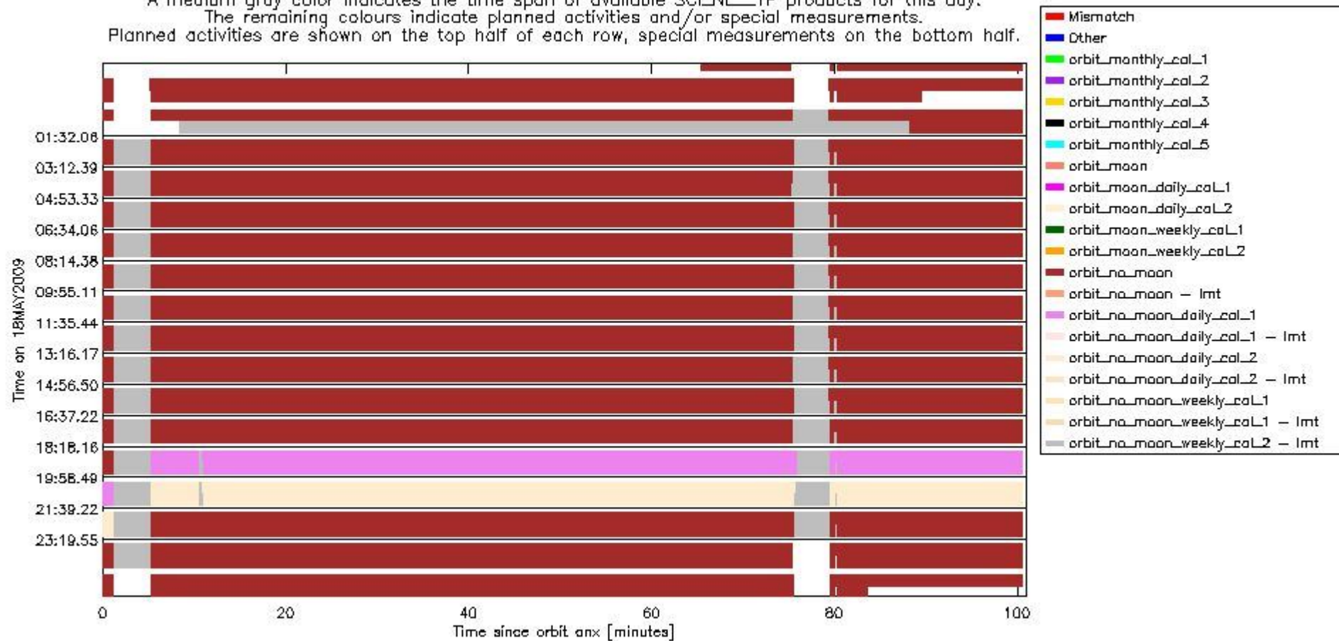
sciamachy_daily_report_level0_KSPT_L0_4303_N_20090518_6.PNG
