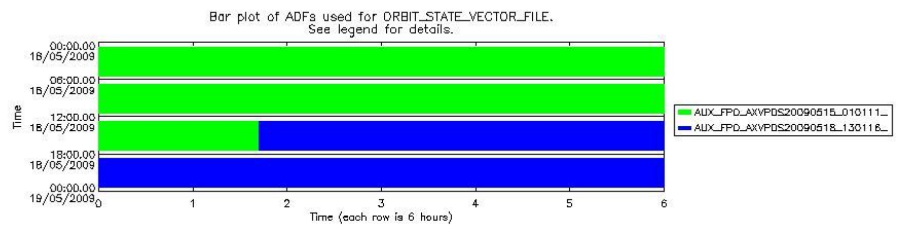
sciamachy_daily_report_level0_KSPT_L0_4303_N_20090518_8.PNG
