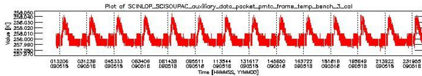
sciamachy_daily_report_level0_KSPT_L0_4303_N_20090518_2.PNG
