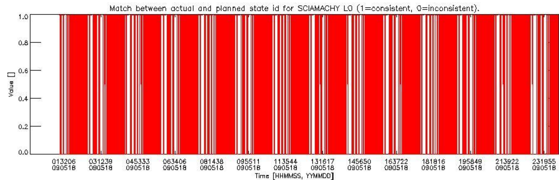
sciamachy_daily_report_level0_KSPT_L0_4303_N_20090518_5.PNG
