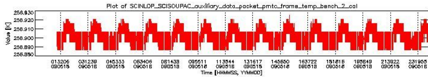
sciamachy_daily_report_level0_KSPT_L0_4303_N_20090518_1.PNG
