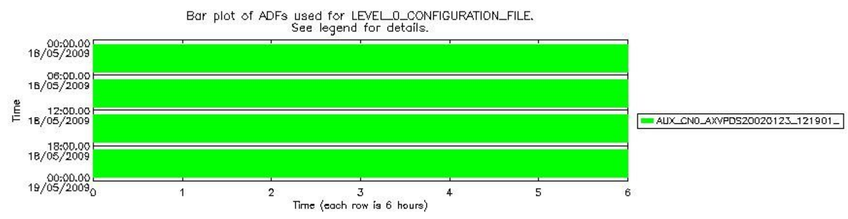
sciamachy_daily_report_level0_KSPT_L0_4303_N_20090518_7.PNG
