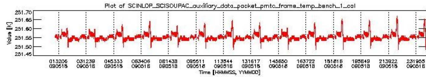
sciamachy_daily_report_level0_KSPT_L0_4303_N_20090518_0.PNG
