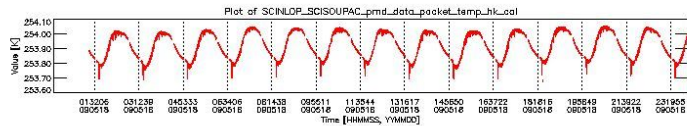
sciamachy_daily_report_level0_KSPT_L0_4303_N_20090518_3.PNG
