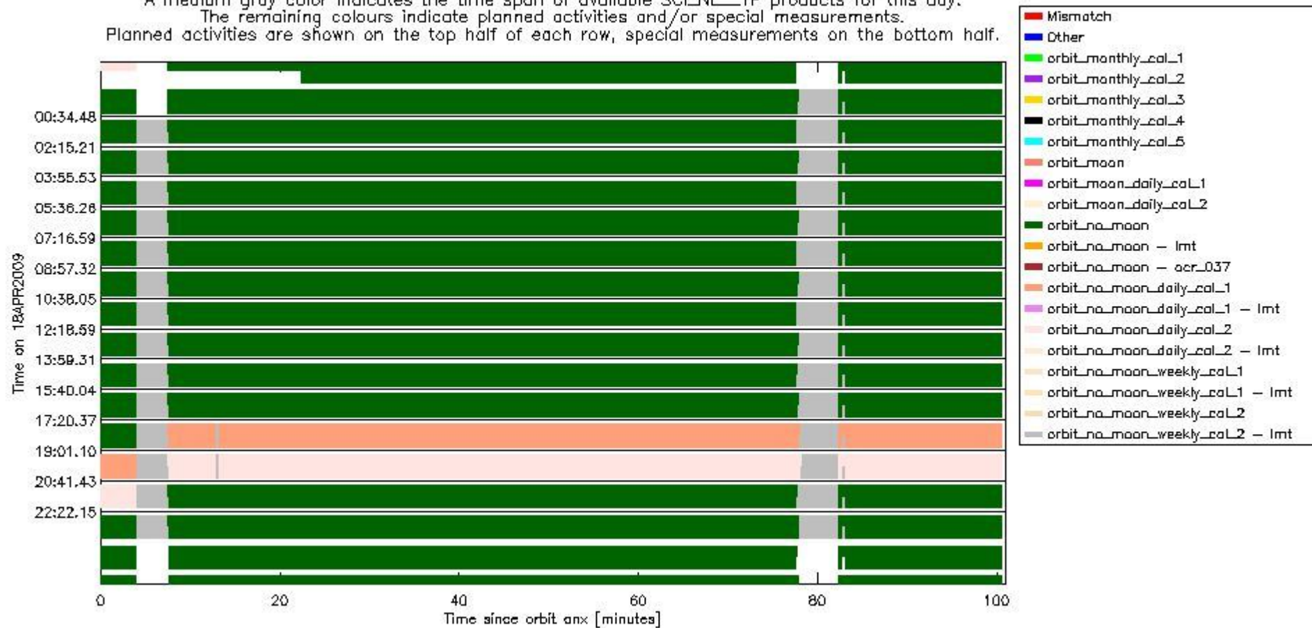
sciamachy_daily_report_level0_KSPT_L0_4303_N_20090418_6.PNG
