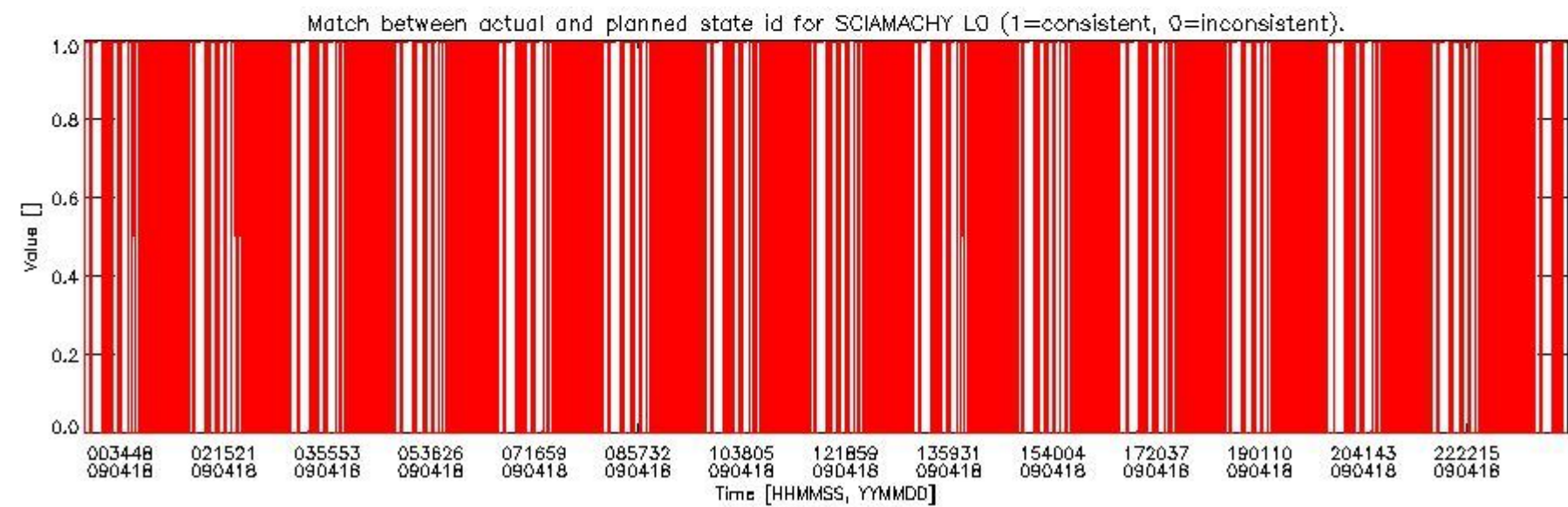
sciamachy_daily_report_level0_KSPT_L0_4303_N_20090418_5.PNG
