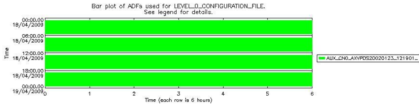
sciamachy_daily_report_level0_KSPT_L0_4303_N_20090418_7.PNG
