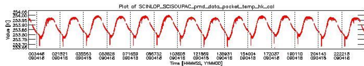
sciamachy_daily_report_level0_KSPT_L0_4303_N_20090418_3.PNG
