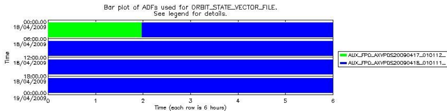
sciamachy_daily_report_level0_KSPT_L0_4303_N_20090418_8.PNG
