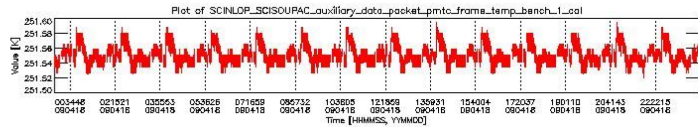
sciamachy_daily_report_level0_KSPT_L0_4303_N_20090418_0.PNG
