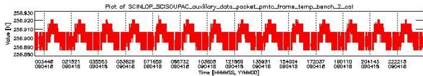
sciamachy_daily_report_level0_KSPT_L0_4303_N_20090418_1.PNG
