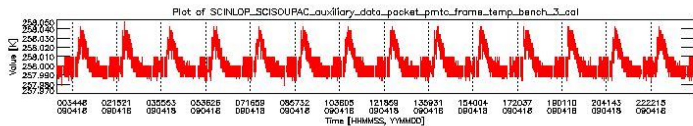
sciamachy_daily_report_level0_KSPT_L0_4303_N_20090418_2.PNG
