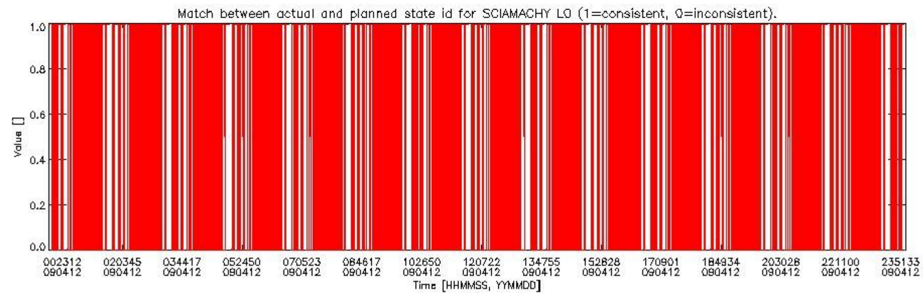
sciamachy_daily_report_level0_KSPT_L0_4303_N_20090412_5.PNG
