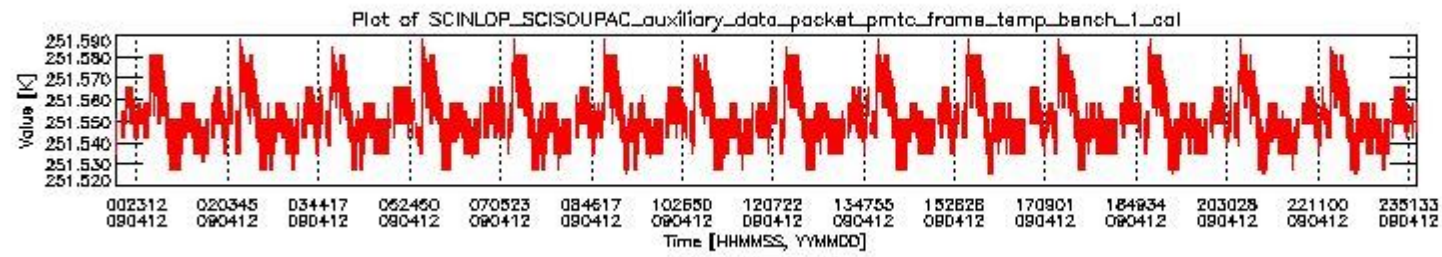
sciamachy_daily_report_level0_KSPT_L0_4303_N_20090412_0.PNG
