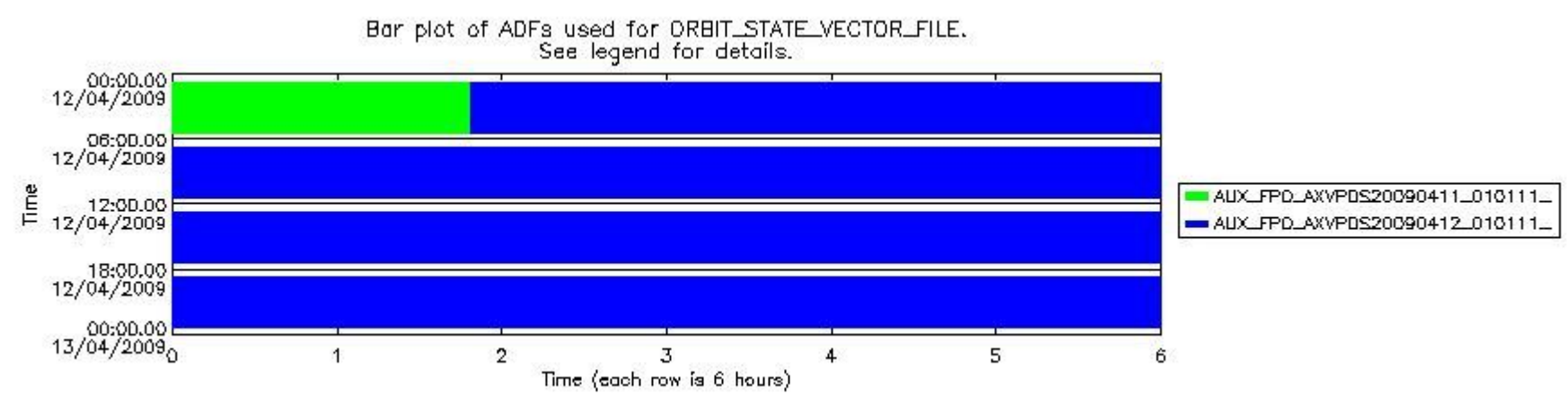
sciamachy_daily_report_level0_KSPT_L0_4303_N_20090412_8.PNG
