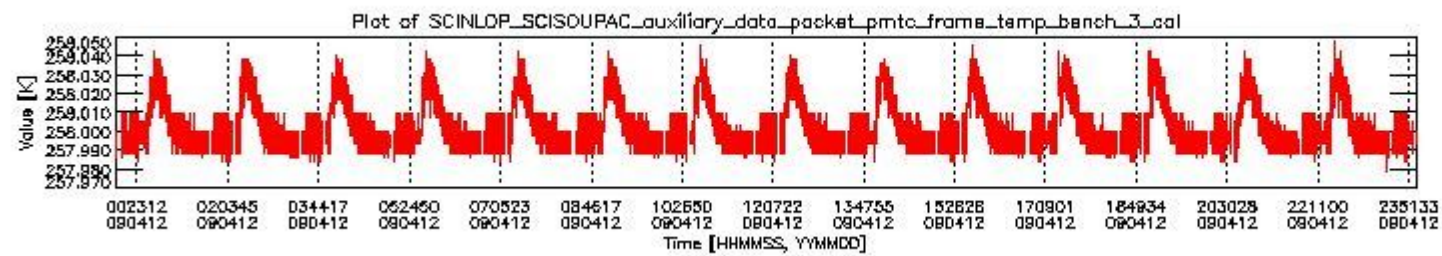
sciamachy_daily_report_level0_KSPT_L0_4303_N_20090412_2.PNG
