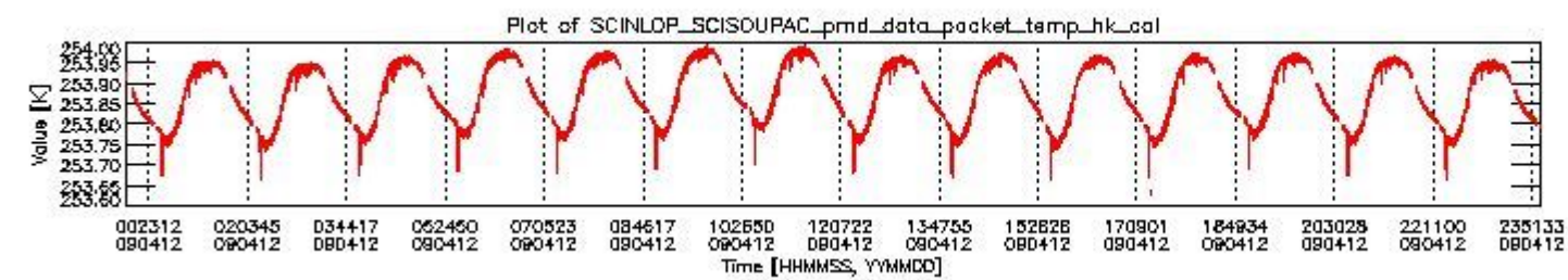
sciamachy_daily_report_level0_KSPT_L0_4303_N_20090412_3.PNG
