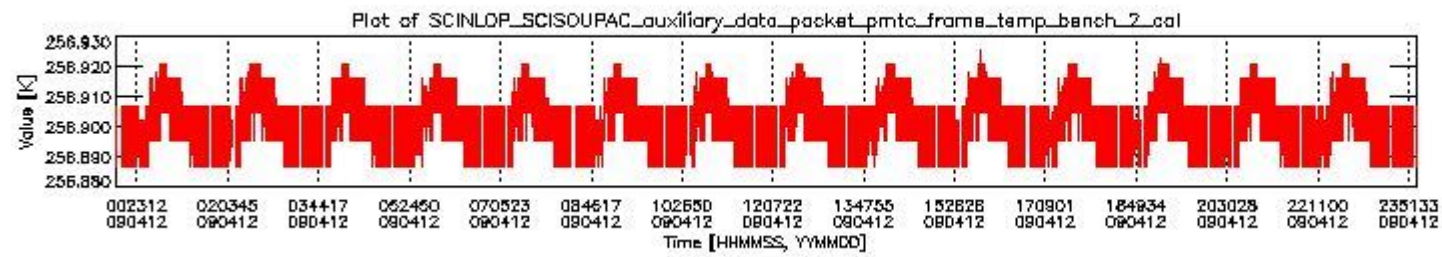
sciamachy_daily_report_level0_KSPT_L0_4303_N_20090412_1.PNG
