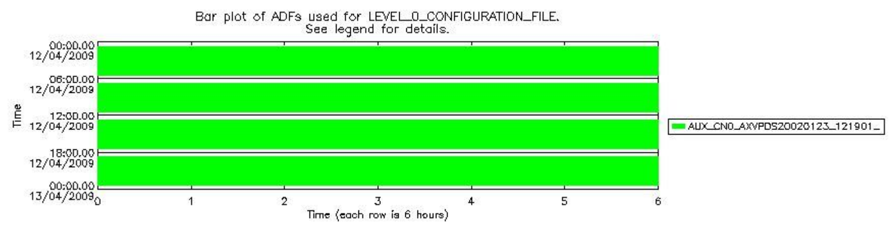
sciamachy_daily_report_level0_KSPT_L0_4303_N_20090412_7.PNG
