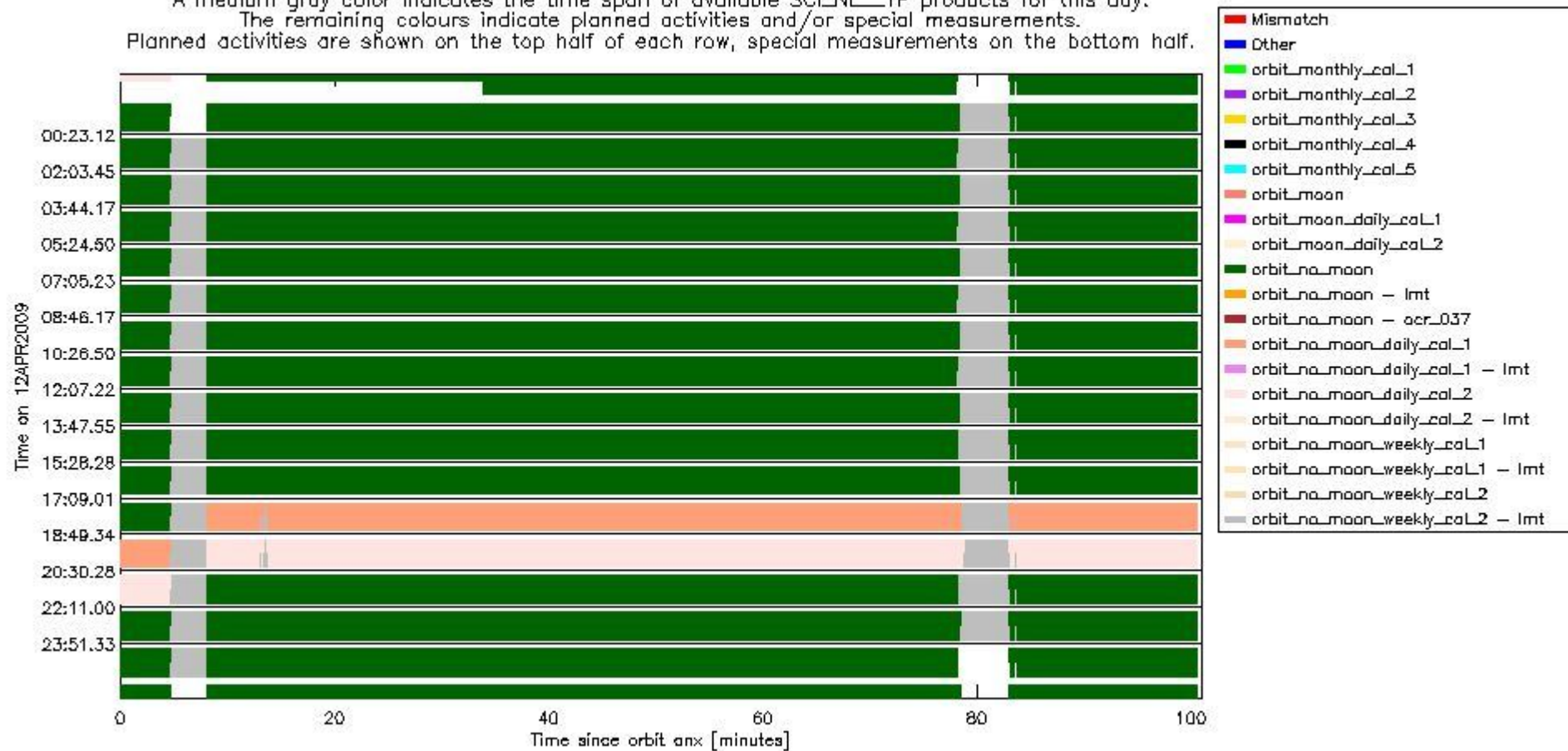
sciamachy_daily_report_level0_KSPT_L0_4303_N_20090412_6.PNG
