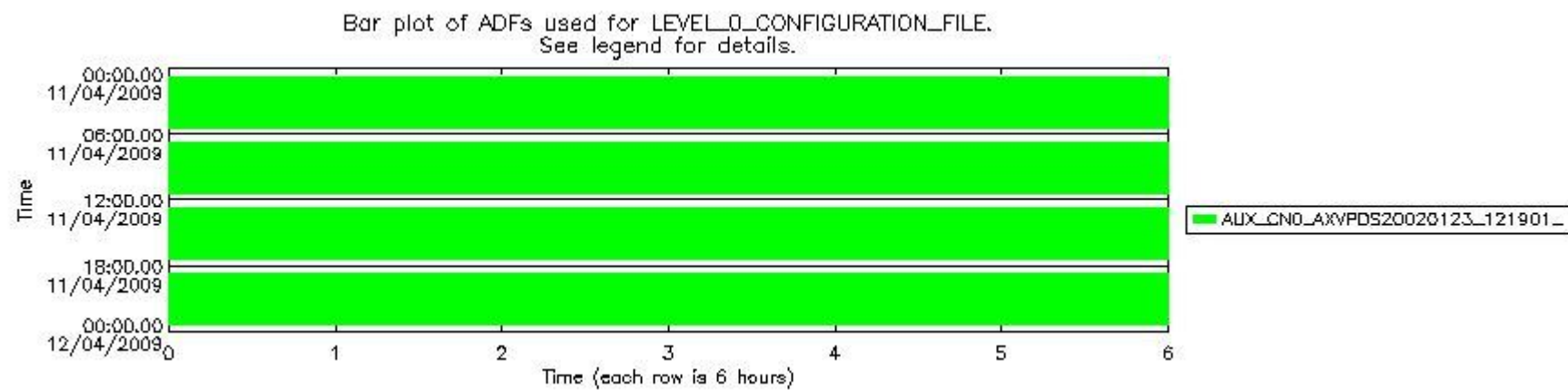
sciamachy_daily_report_level0_KSPT_L0_4303_N_20090411_7.PNG
