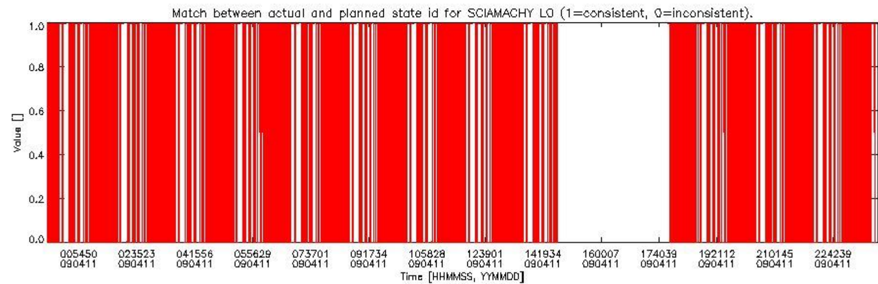
sciamachy_daily_report_level0_KSPT_L0_4303_N_20090411_5.PNG
