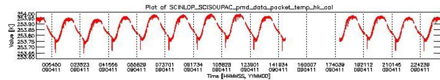
sciamachy_daily_report_level0_KSPT_L0_4303_N_20090411_3.PNG
