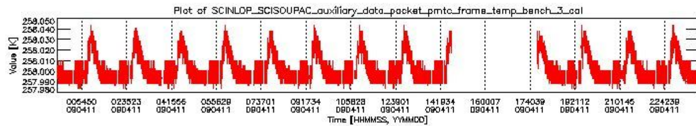
sciamachy_daily_report_level0_KSPT_L0_4303_N_20090411_2.PNG
