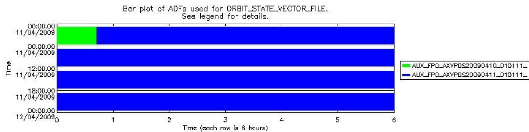
sciamachy_daily_report_level0_KSPT_L0_4303_N_20090411_8.PNG
