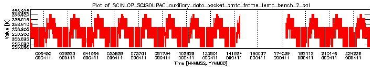
sciamachy_daily_report_level0_KSPT_L0_4303_N_20090411_1.PNG
