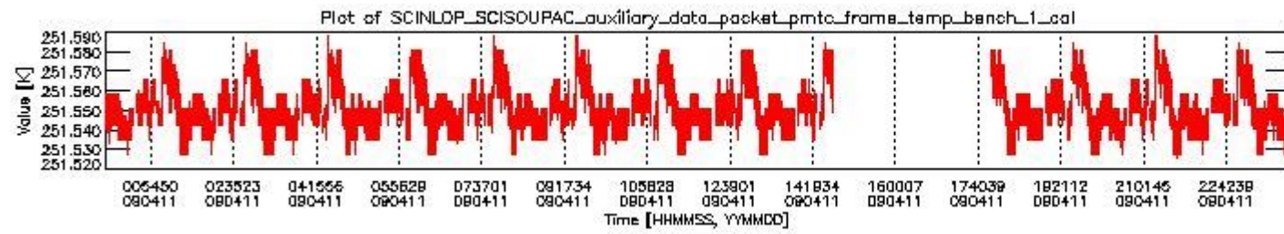
sciamachy_daily_report_level0_KSPT_L0_4303_N_20090411_0.PNG
