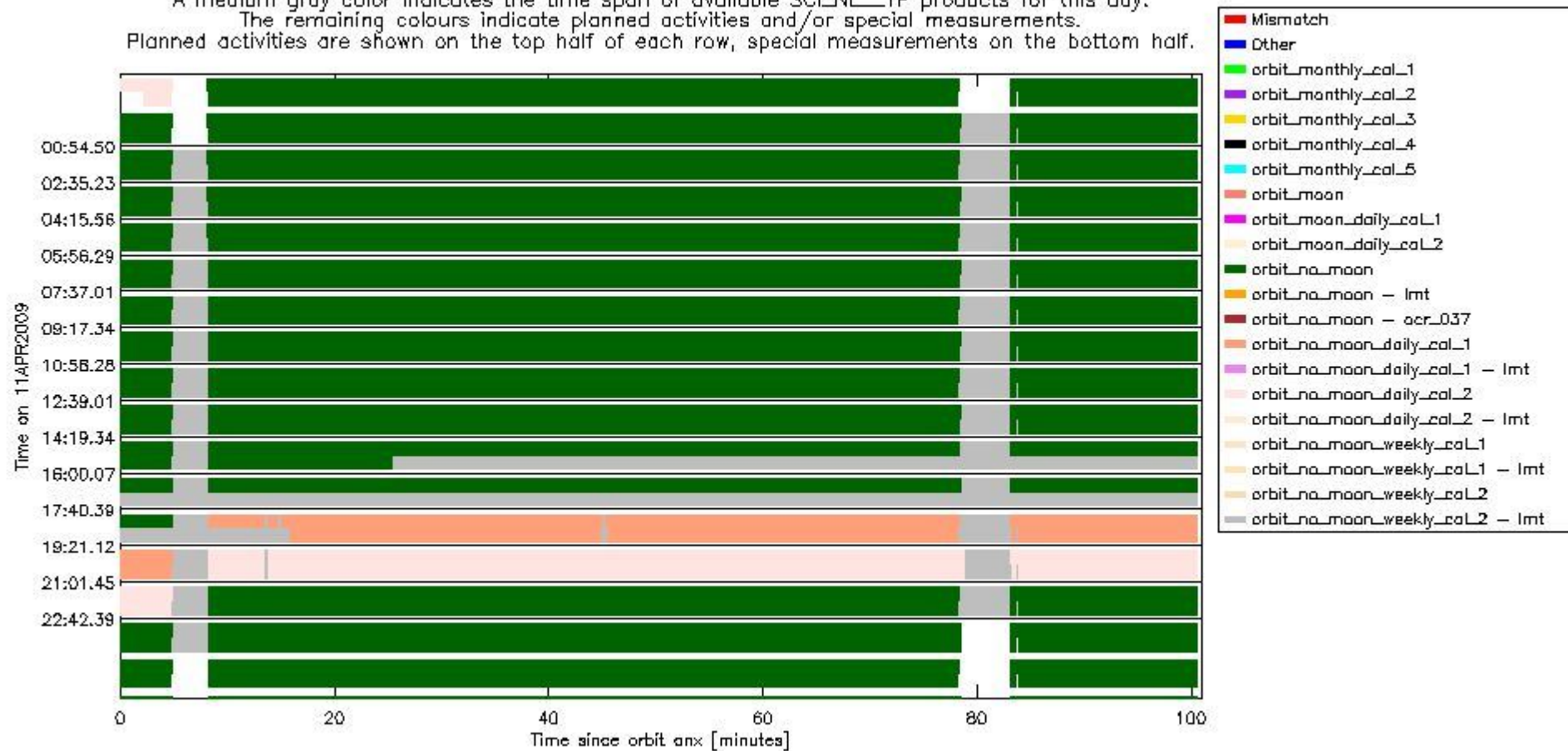
sciamachy_daily_report_level0_KSPT_L0_4303_N_20090411_6.PNG
