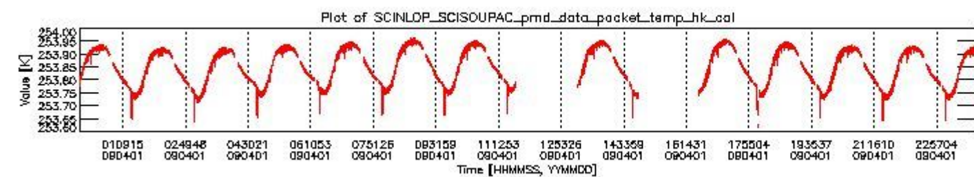
sciamachy_daily_report_level0_KSPT_L0_4303_N_20090401_3.PNG
