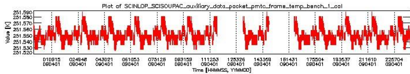
sciamachy_daily_report_level0_KSPT_L0_4303_N_20090401_0.PNG
