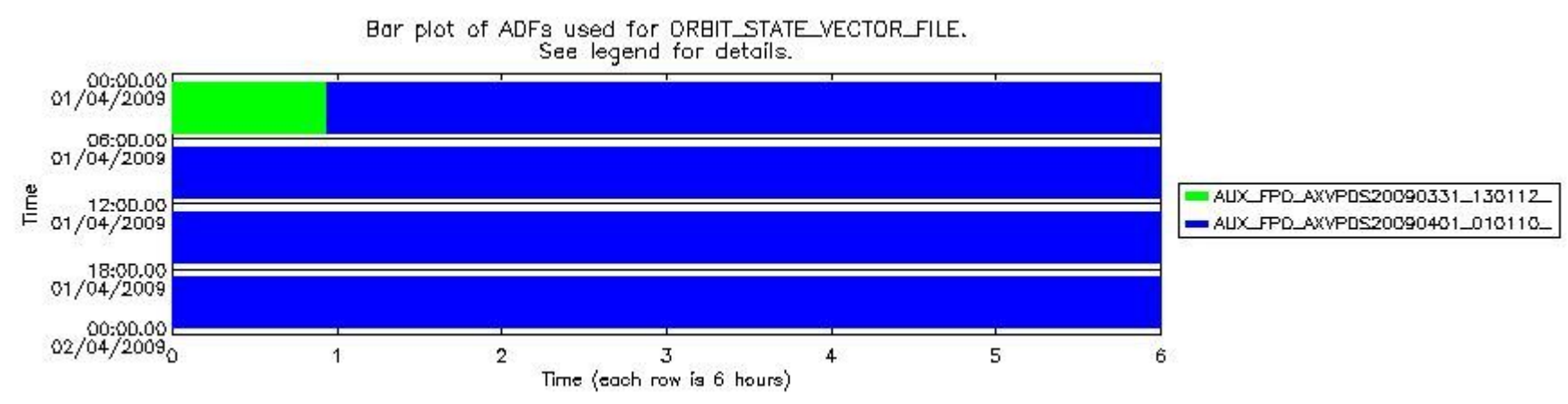
sciamachy_daily_report_level0_KSPT_L0_4303_N_20090401_8.PNG
