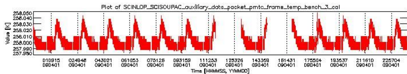
sciamachy_daily_report_level0_KSPT_L0_4303_N_20090401_2.PNG
