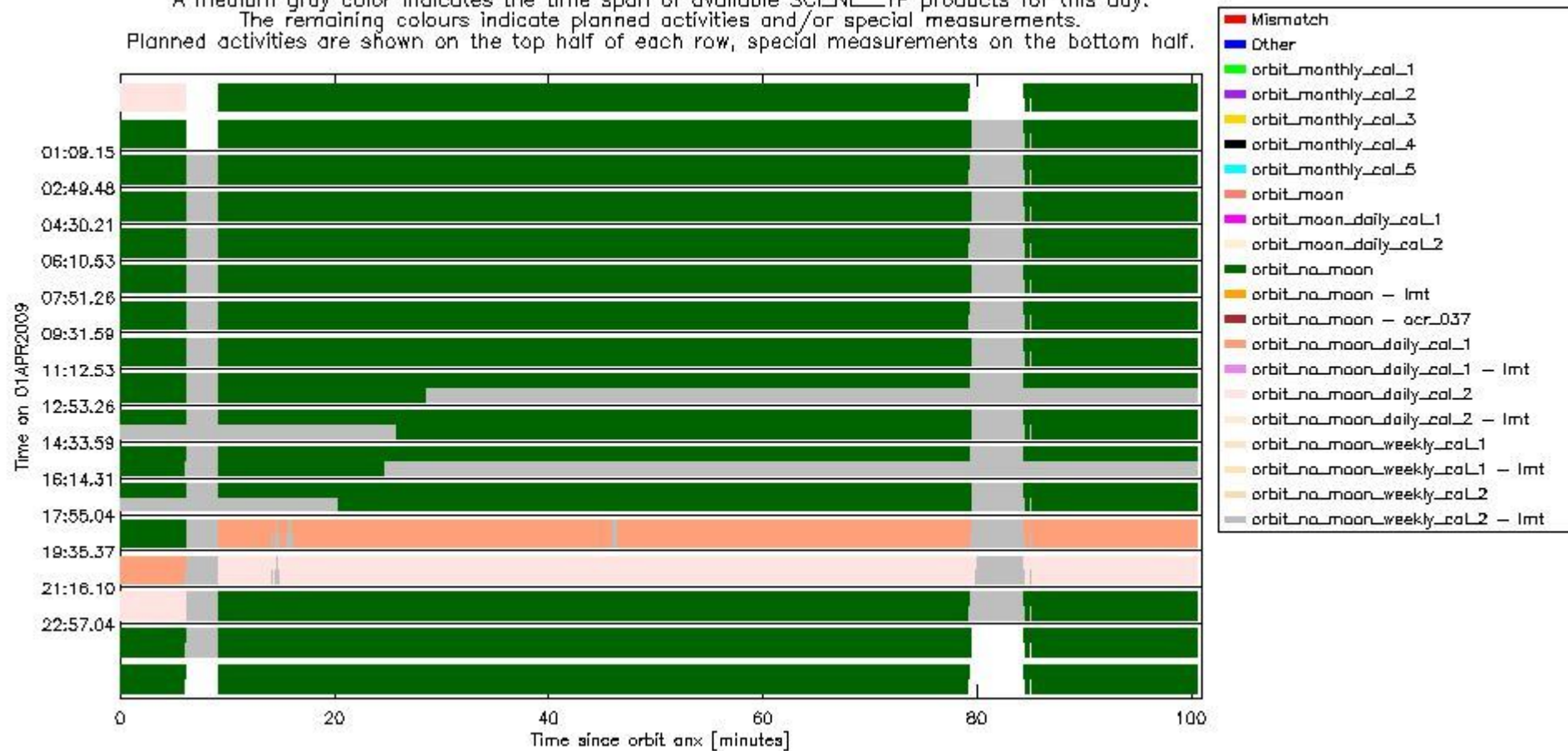
sciamachy_daily_report_level0_KSPT_L0_4303_N_20090401_6.PNG
