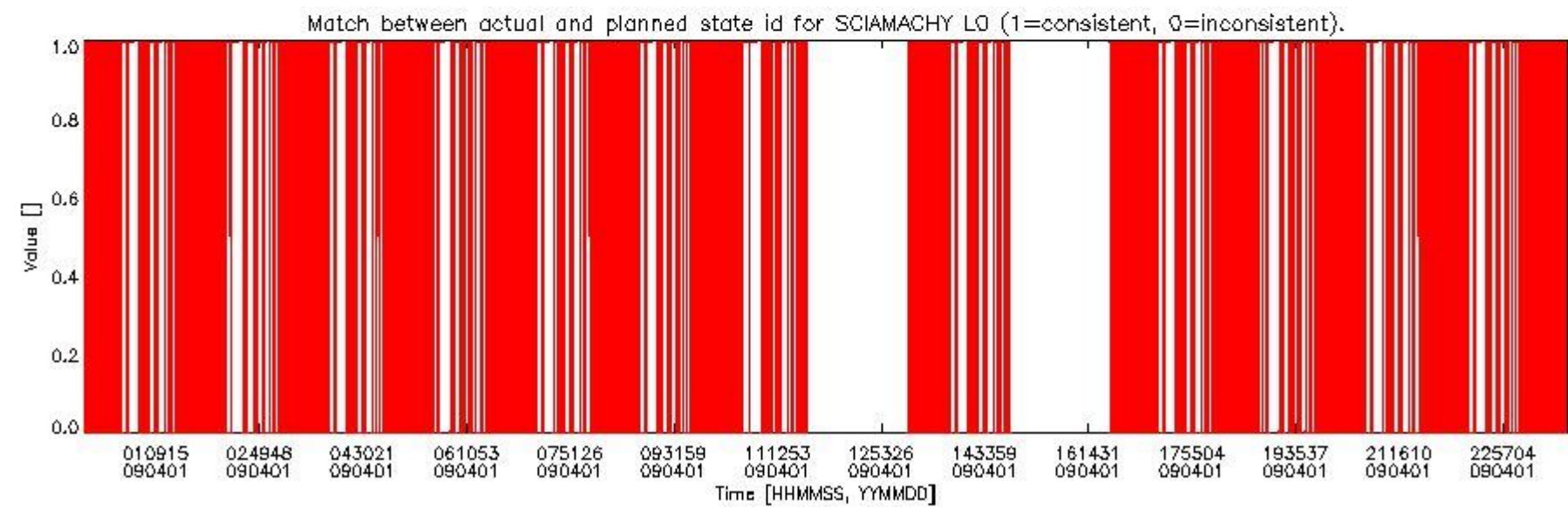
sciamachy_daily_report_level0_KSPT_L0_4303_N_20090401_5.PNG
