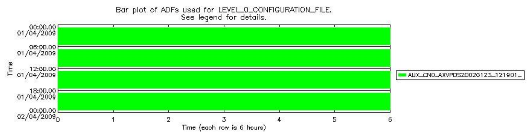
sciamachy_daily_report_level0_KSPT_L0_4303_N_20090401_7.PNG
