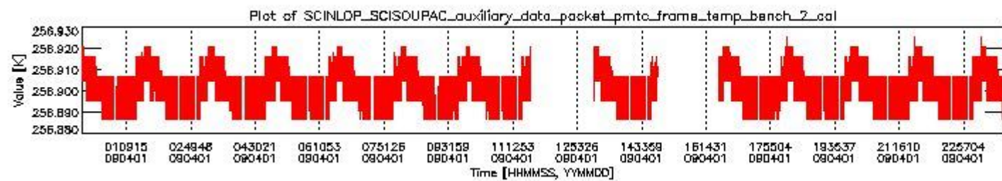
sciamachy_daily_report_level0_KSPT_L0_4303_N_20090401_1.PNG
