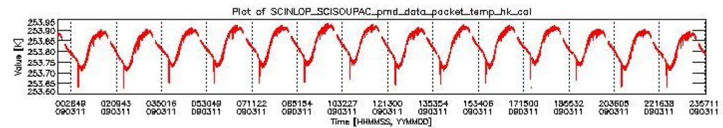
sciamachy_daily_report_level0_KSPT_L0_4303_N_20090311_3.PNG
