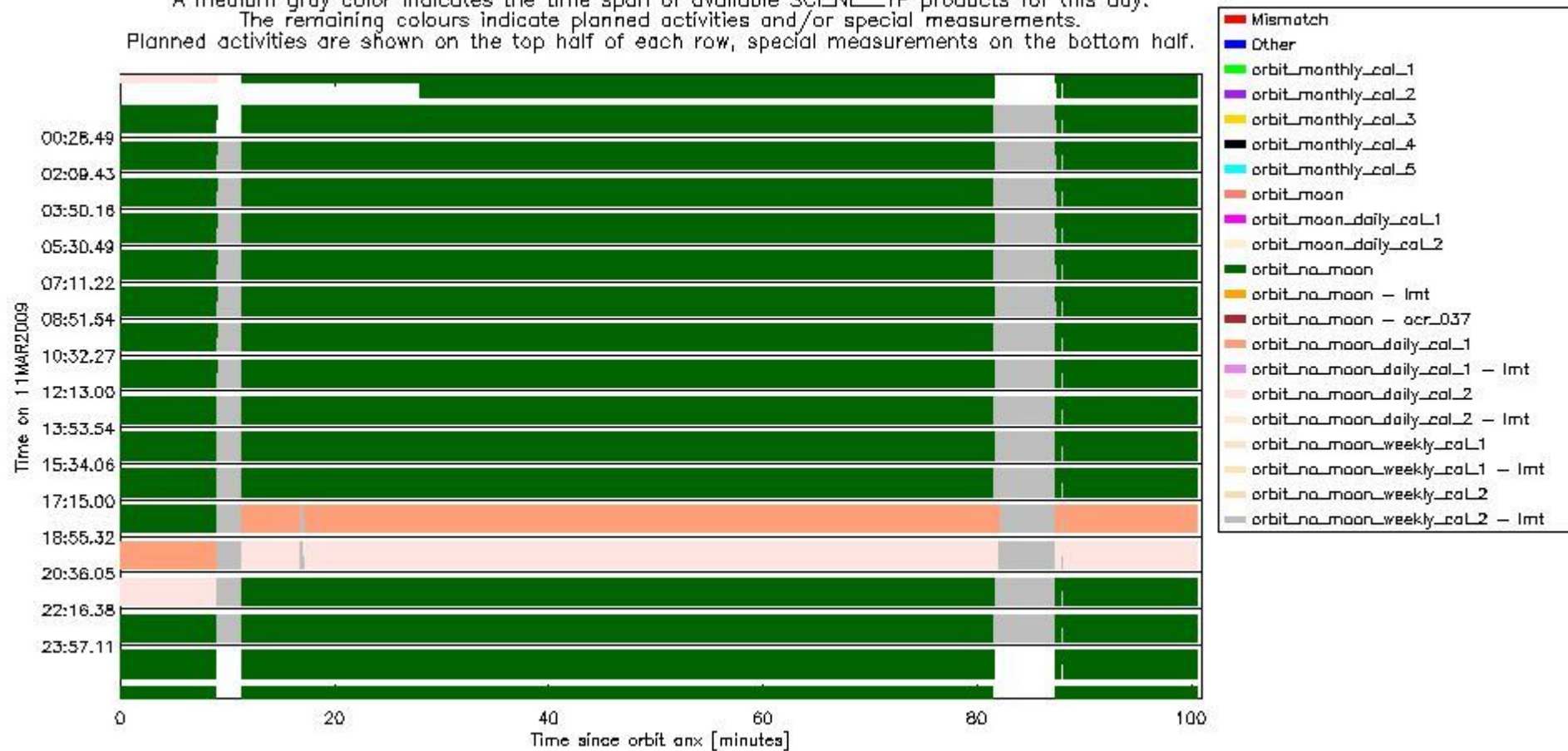
sciamachy_daily_report_level0_KSPT_L0_4303_N_20090311_6.PNG
