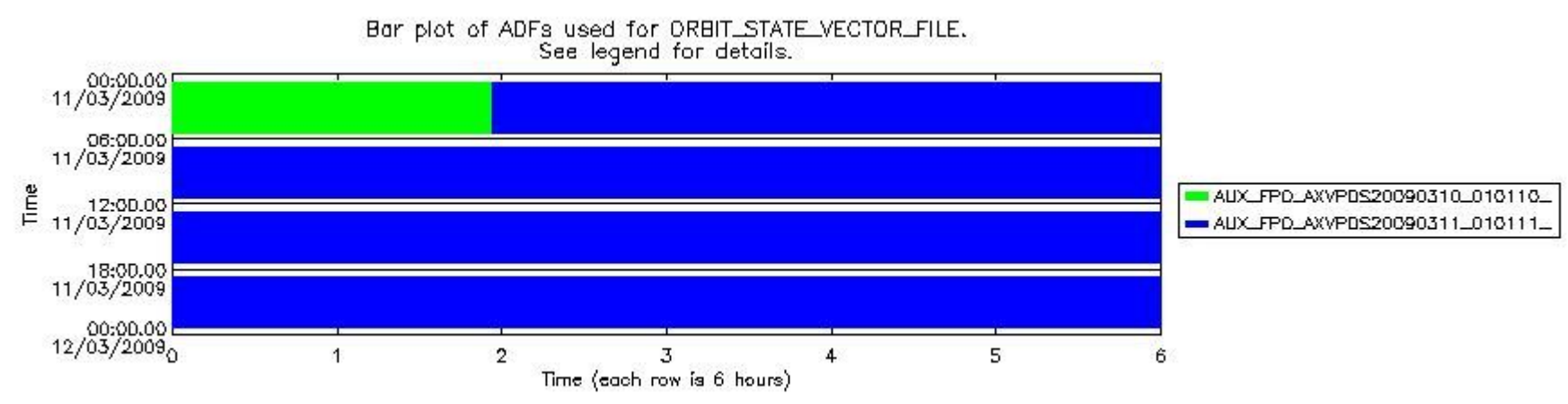
sciamachy_daily_report_level0_KSPT_L0_4303_N_20090311_8.PNG
