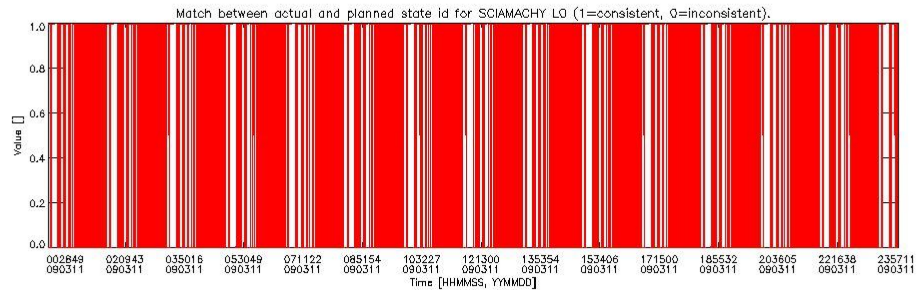
sciamachy_daily_report_level0_KSPT_L0_4303_N_20090311_5.PNG
