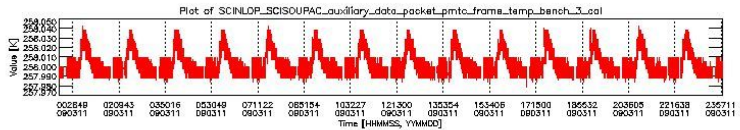
sciamachy_daily_report_level0_KSPT_L0_4303_N_20090311_2.PNG
