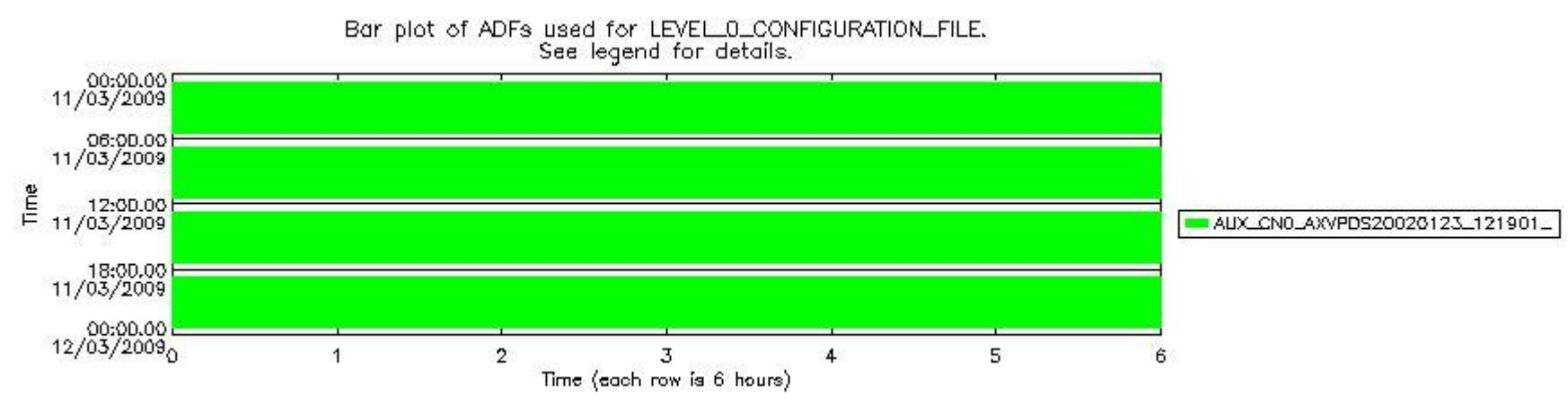
sciamachy_daily_report_level0_KSPT_L0_4303_N_20090311_7.PNG
