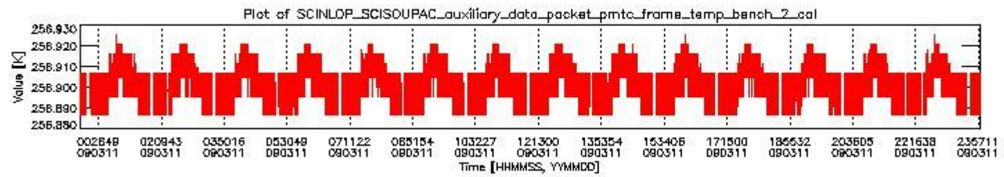
sciamachy_daily_report_level0_KSPT_L0_4303_N_20090311_1.PNG
