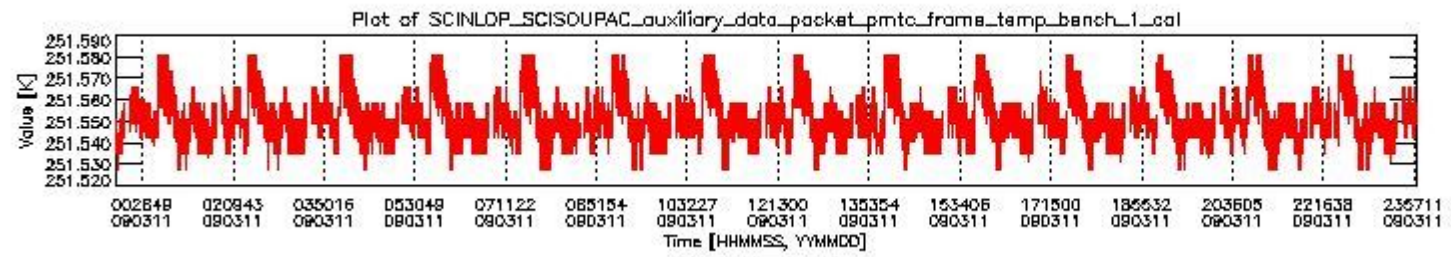
sciamachy_daily_report_level0_KSPT_L0_4303_N_20090311_0.PNG
