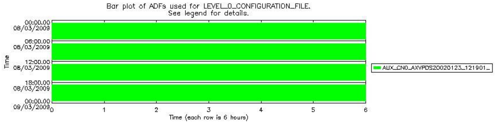
sciamachy_daily_report_level0_KSPT_L0_4303_N_20090308_7.PNG
