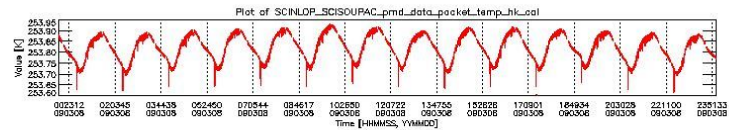
sciamachy_daily_report_level0_KSPT_L0_4303_N_20090308_3.PNG
