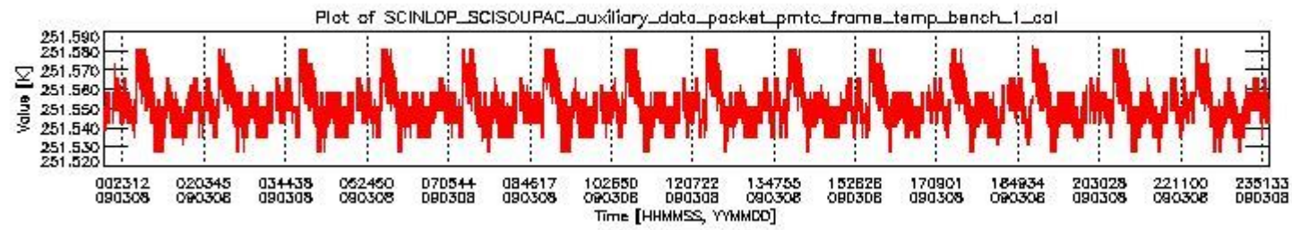
sciamachy_daily_report_level0_KSPT_L0_4303_N_20090308_0.PNG
