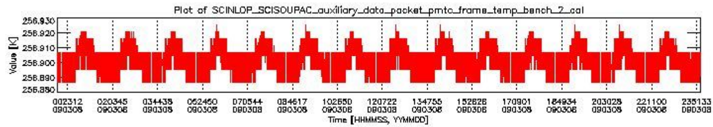
sciamachy_daily_report_level0_KSPT_L0_4303_N_20090308_1.PNG
