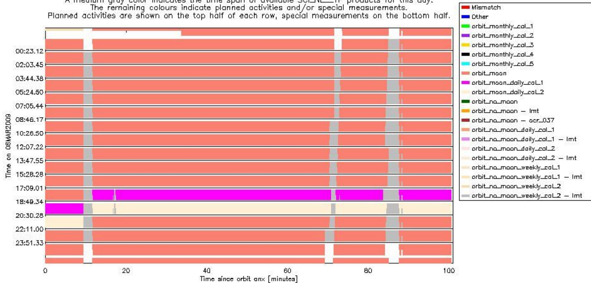
sciamachy_daily_report_level0_KSPT_L0_4303_N_20090308_6.PNG
