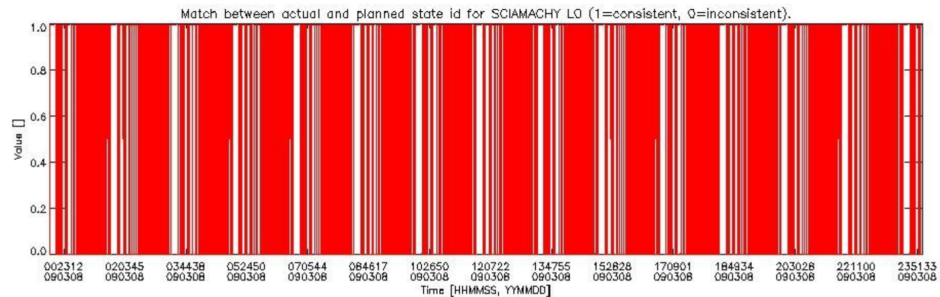
sciamachy_daily_report_level0_KSPT_L0_4303_N_20090308_5.PNG
