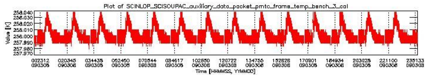
sciamachy_daily_report_level0_KSPT_L0_4303_N_20090308_2.PNG
