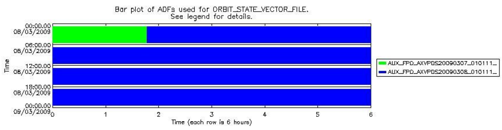
sciamachy_daily_report_level0_KSPT_L0_4303_N_20090308_8.PNG
