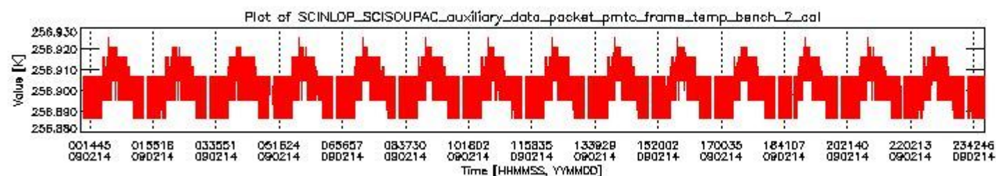
sciamachy_daily_report_level0_KSPT_L0_4303_N_20090214_1.PNG
