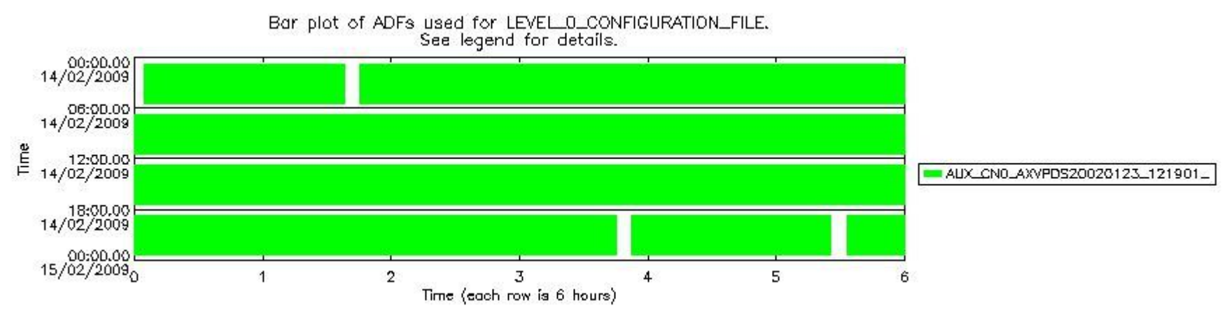
sciamachy_daily_report_level0_KSPT_L0_4303_N_20090214_7.PNG
