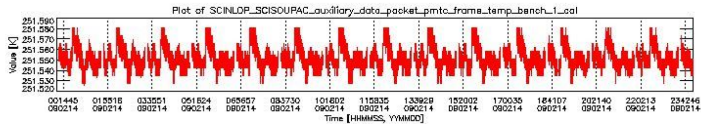
sciamachy_daily_report_level0_KSPT_L0_4303_N_20090214_0.PNG
