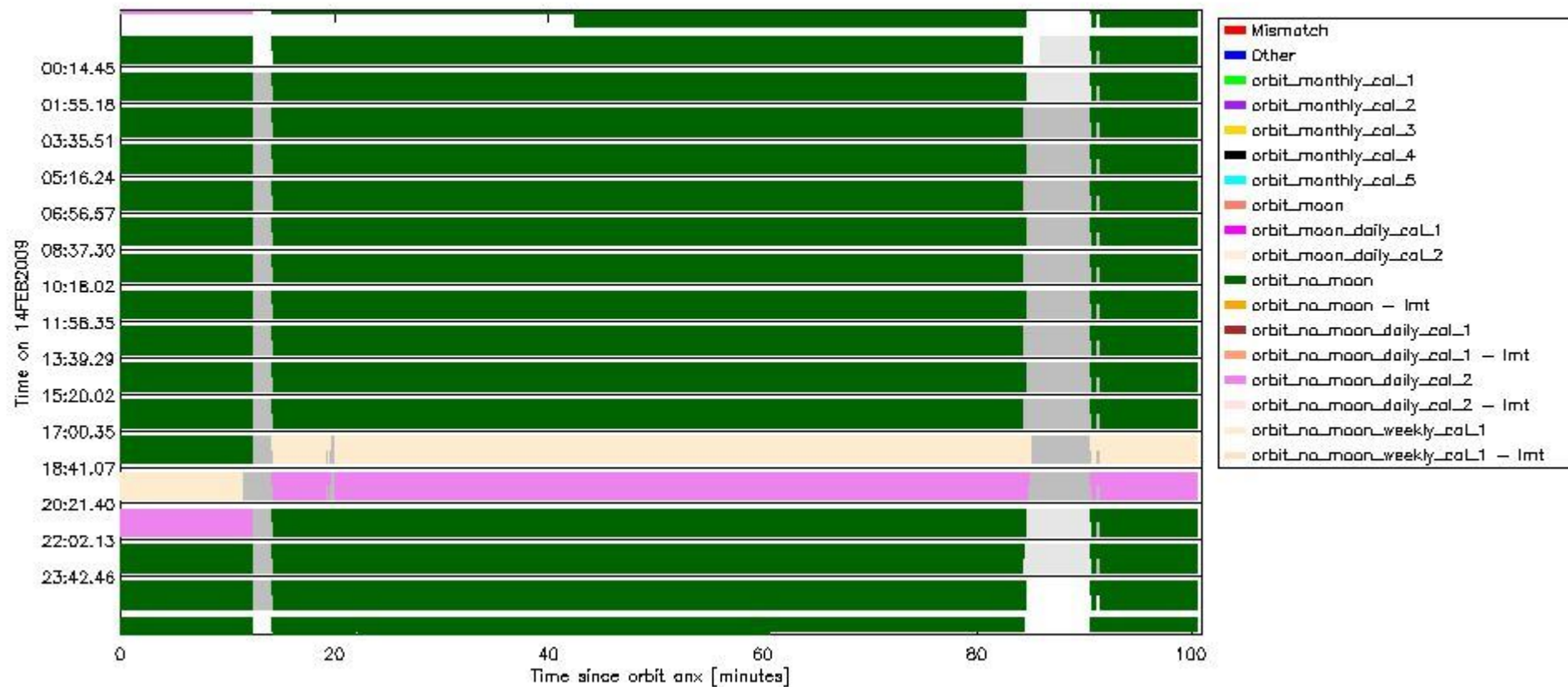
sciamachy_daily_report_level0_KSPT_L0_4303_N_20090214_6.PNG
