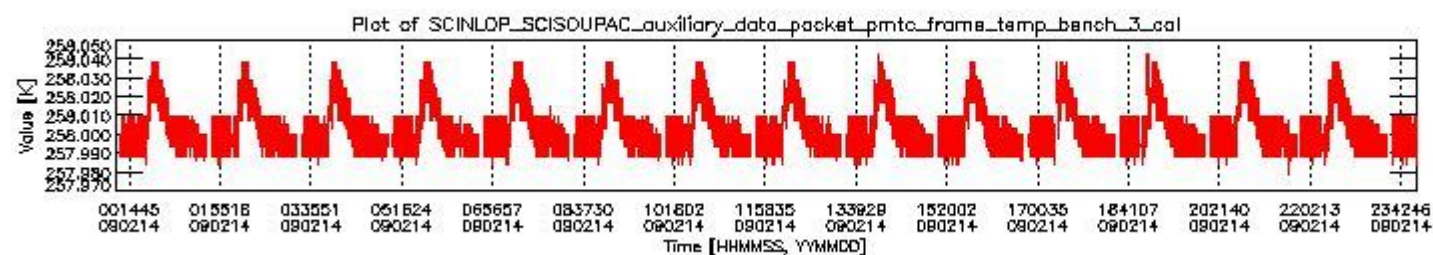
sciamachy_daily_report_level0_KSPT_L0_4303_N_20090214_2.PNG
