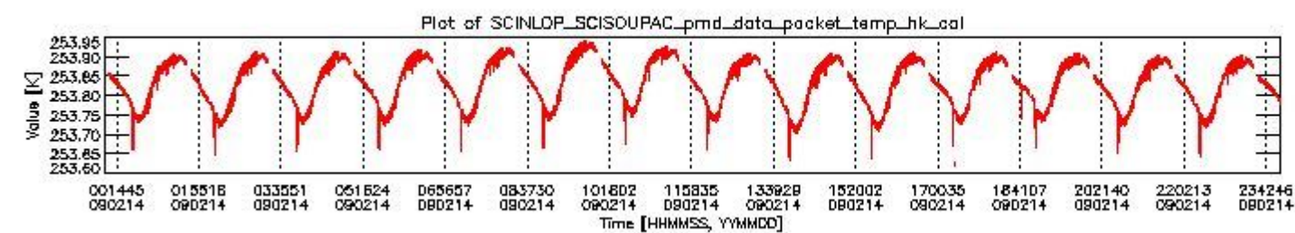
sciamachy_daily_report_level0_KSPT_L0_4303_N_20090214_3.PNG
