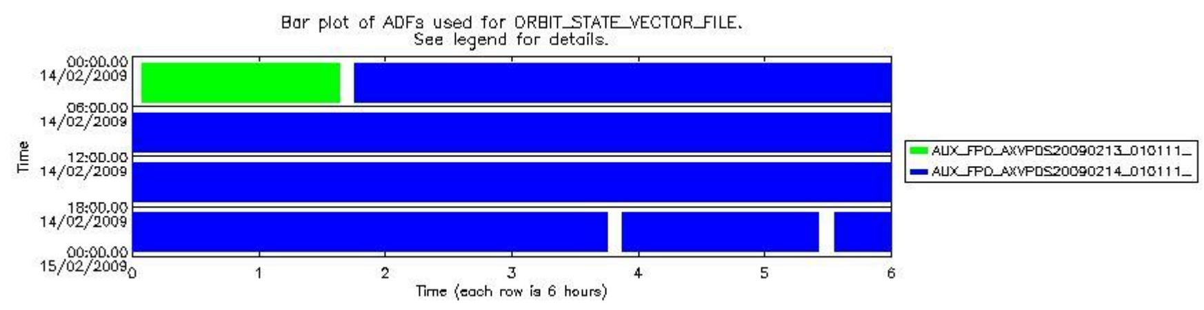
sciamachy_daily_report_level0_KSPT_L0_4303_N_20090214_8.PNG
