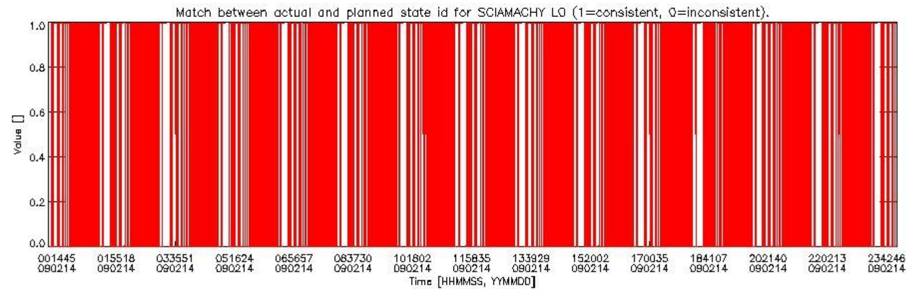
sciamachy_daily_report_level0_KSPT_L0_4303_N_20090214_5.PNG
