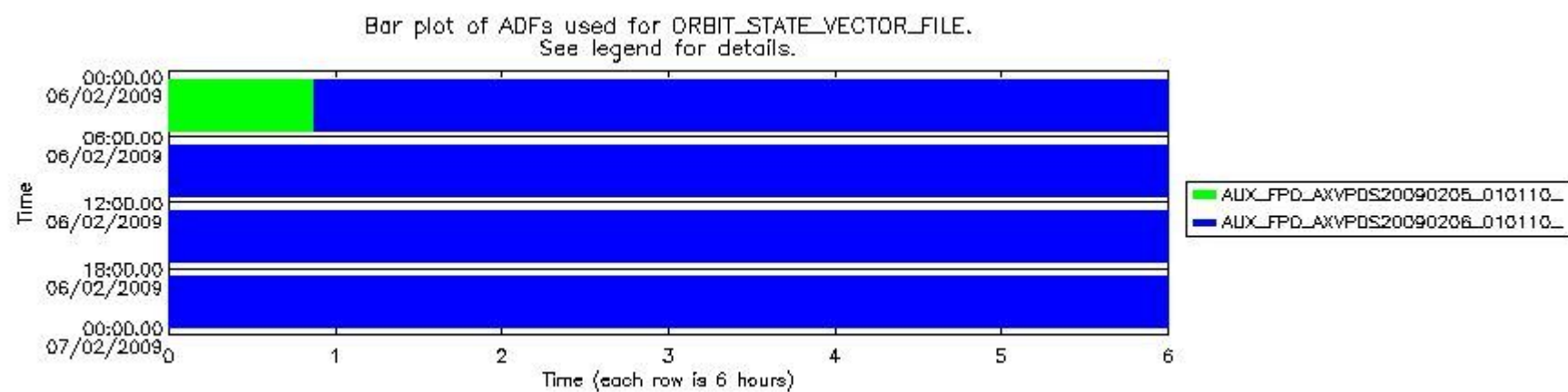
sciamachy_daily_report_level0_KSPT_L0_4303_N_20090206_8.PNG
