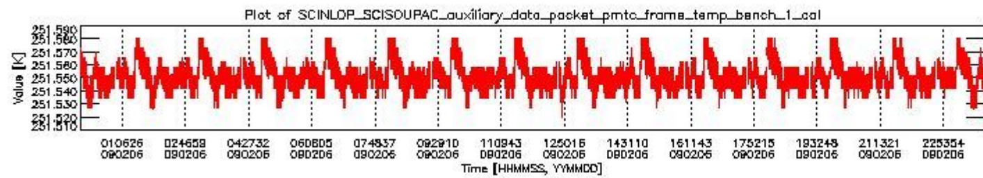
sciamachy_daily_report_level0_KSPT_L0_4303_N_20090206_0.PNG
