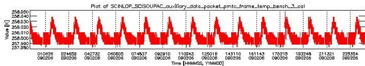
sciamachy_daily_report_level0_KSPT_L0_4303_N_20090206_2.PNG
