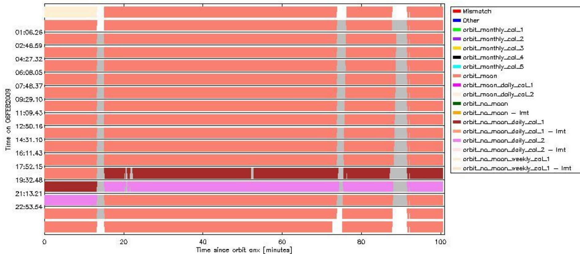
sciamachy_daily_report_level0_KSPT_L0_4303_N_20090206_6.PNG
