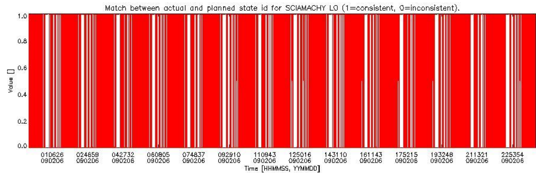
sciamachy_daily_report_level0_KSPT_L0_4303_N_20090206_5.PNG
