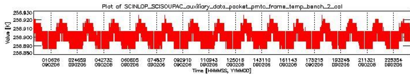
sciamachy_daily_report_level0_KSPT_L0_4303_N_20090206_1.PNG
