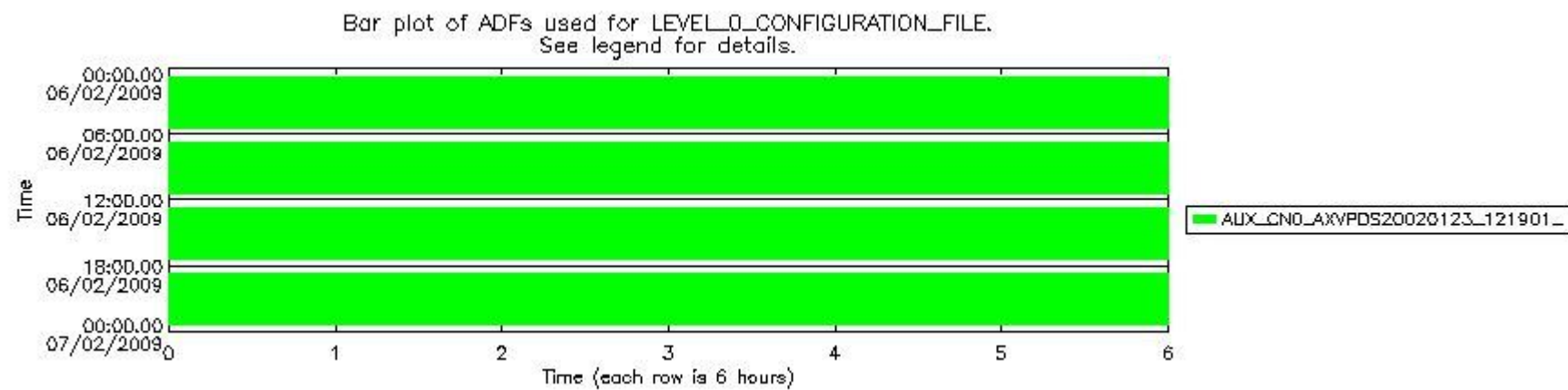
sciamachy_daily_report_level0_KSPT_L0_4303_N_20090206_7.PNG
