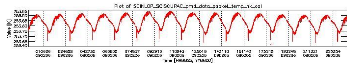
sciamachy_daily_report_level0_KSPT_L0_4303_N_20090206_3.PNG
