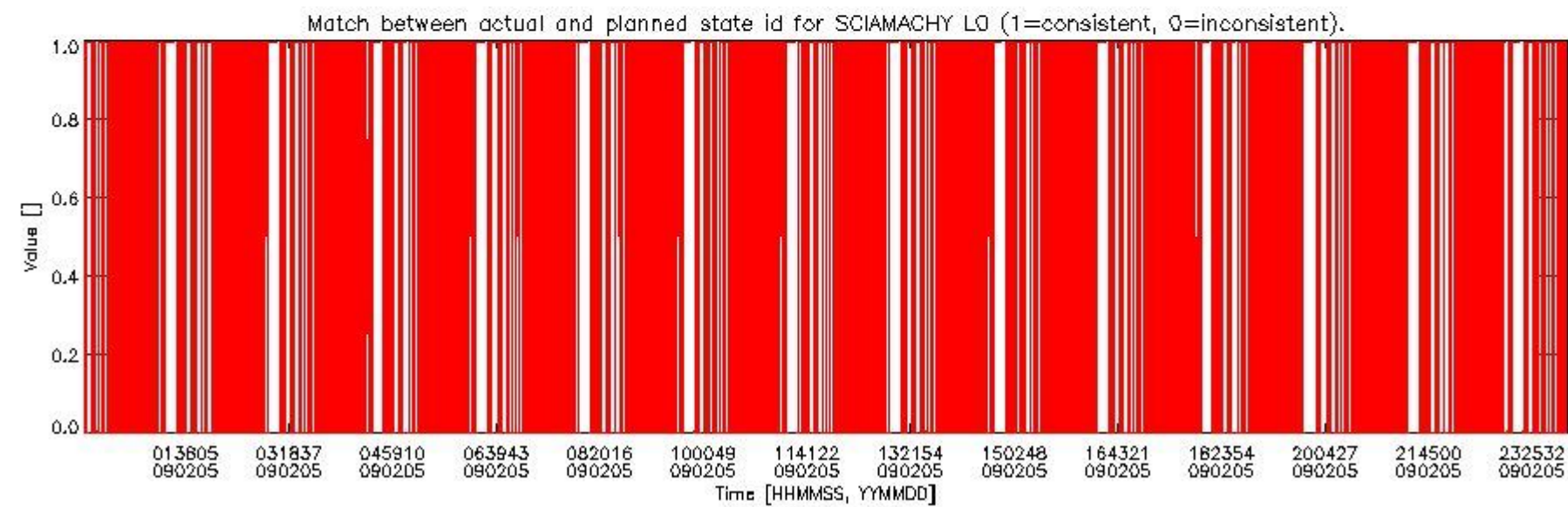
sciamachy_daily_report_level0_KSPT_L0_4303_N_20090205_5.PNG
