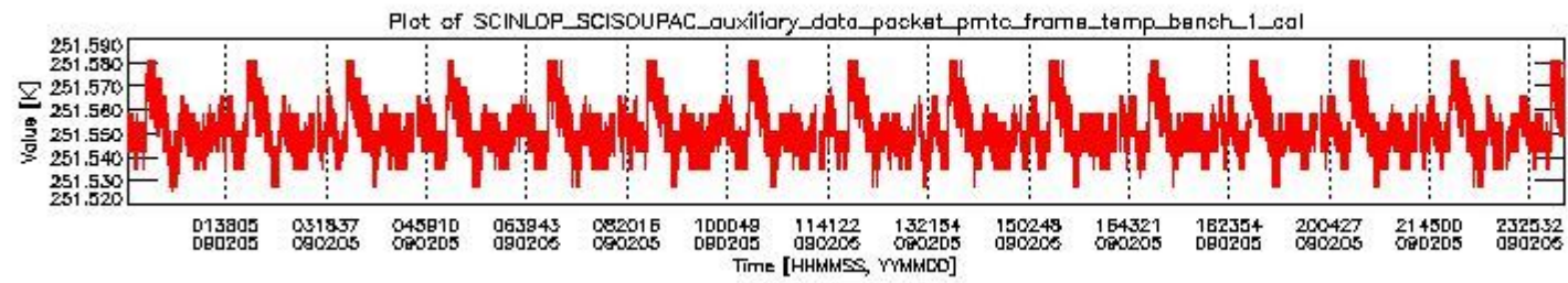
sciamachy_daily_report_level0_KSPT_L0_4303_N_20090205_0.PNG
