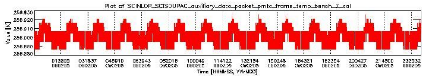
sciamachy_daily_report_level0_KSPT_L0_4303_N_20090205_1.PNG
