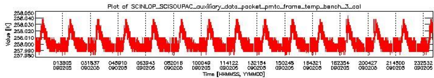
sciamachy_daily_report_level0_KSPT_L0_4303_N_20090205_2.PNG
