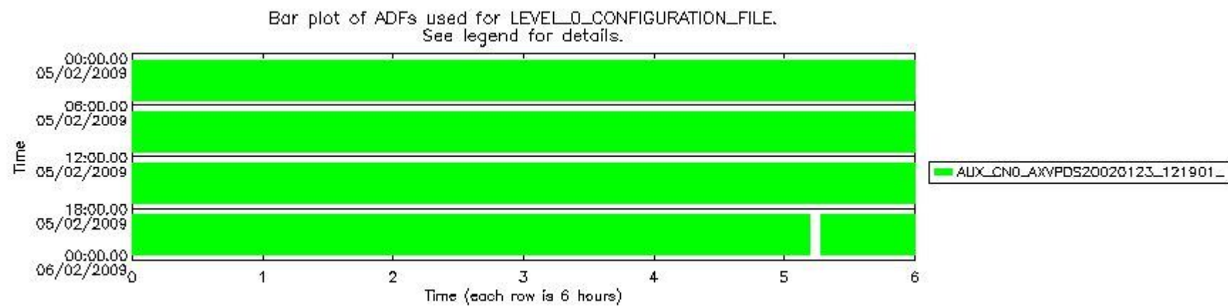
sciamachy_daily_report_level0_KSPT_L0_4303_N_20090205_7.PNG
