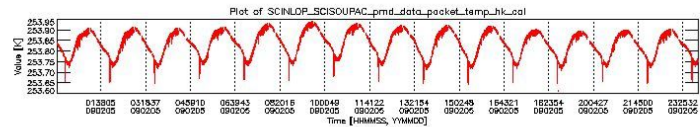
sciamachy_daily_report_level0_KSPT_L0_4303_N_20090205_3.PNG
