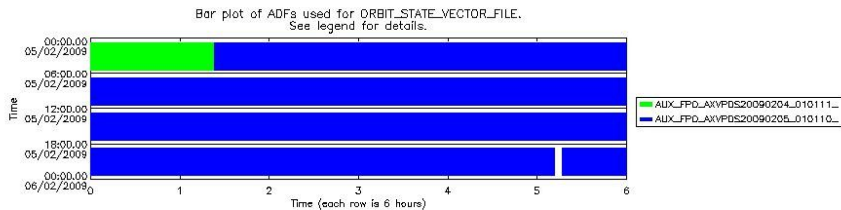
sciamachy_daily_report_level0_KSPT_L0_4303_N_20090205_8.PNG
