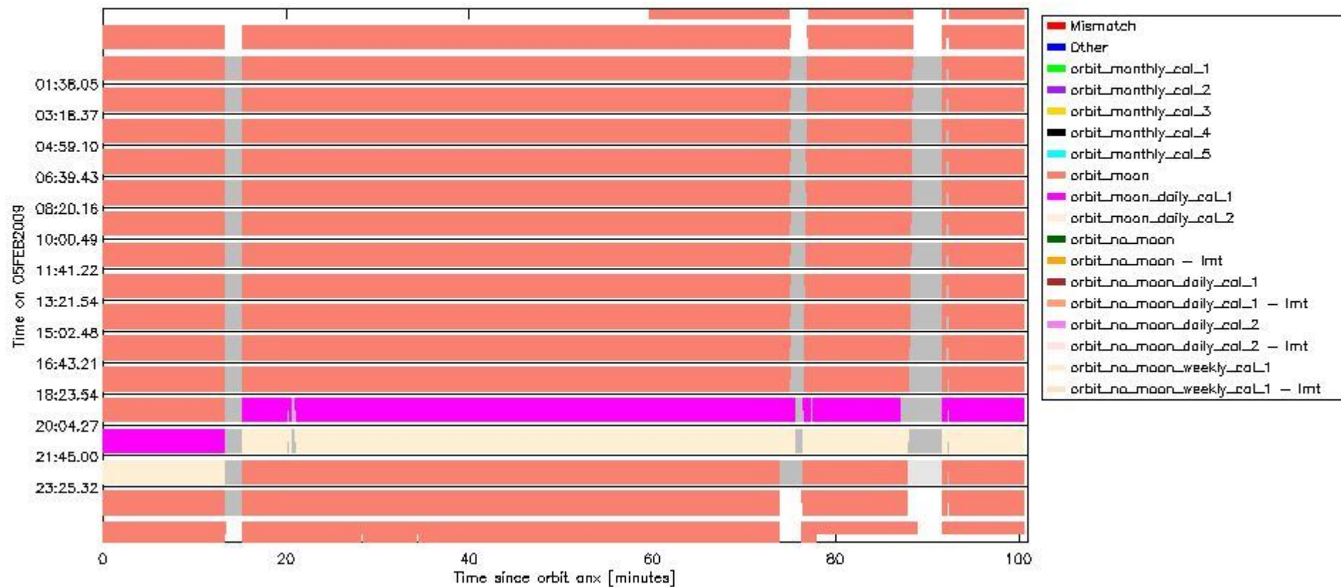
sciamachy_daily_report_level0_KSPT_L0_4303_N_20090205_6.PNG
