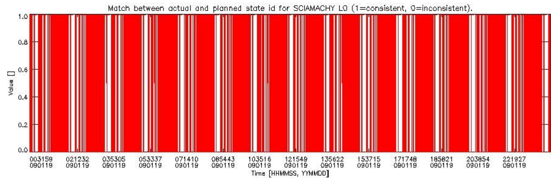
sciamachy_daily_report_level0_KSPT_L0_4303_N_20090119_5.PNG
