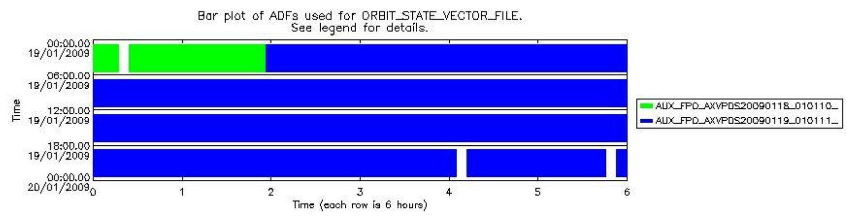
sciamachy_daily_report_level0_KSPT_L0_4303_N_20090119_8.PNG
