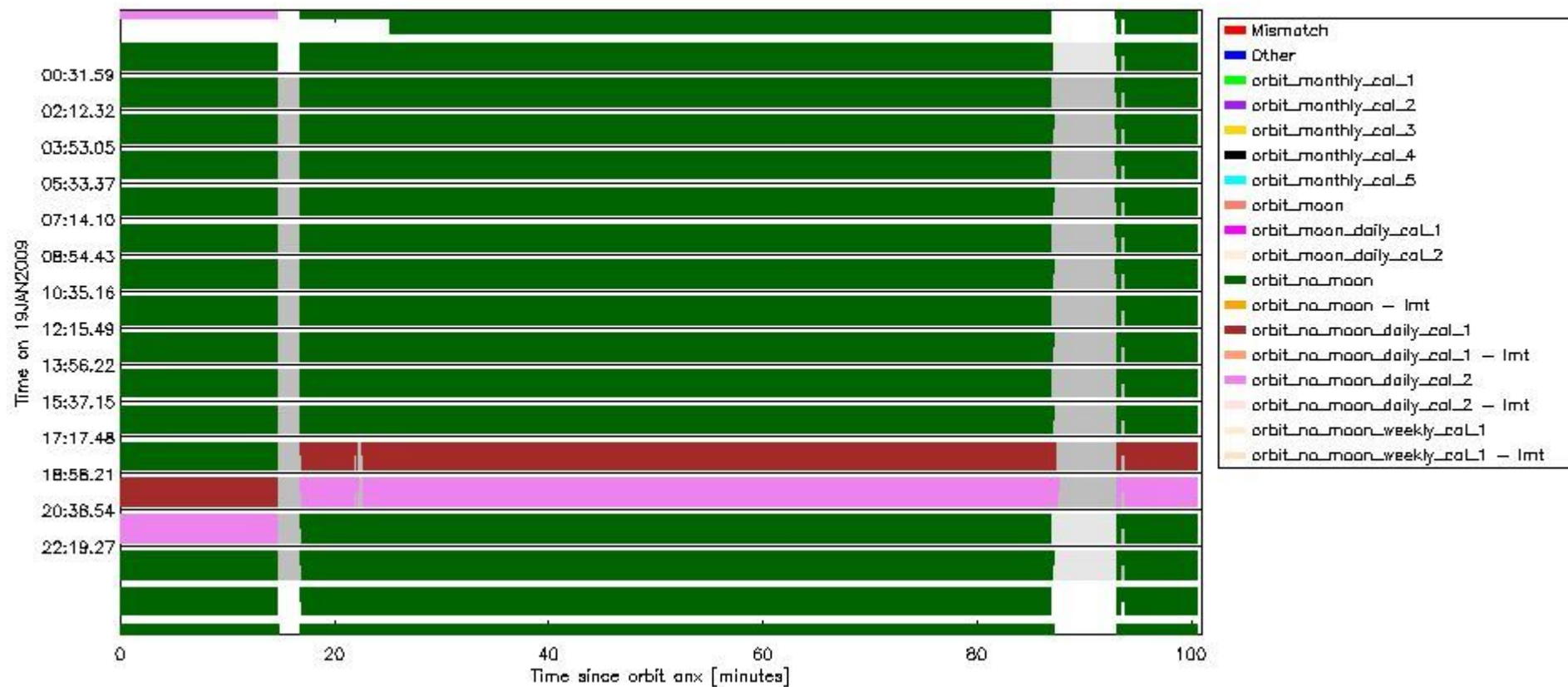
sciamachy_daily_report_level0_KSPT_L0_4303_N_20090119_6.PNG
