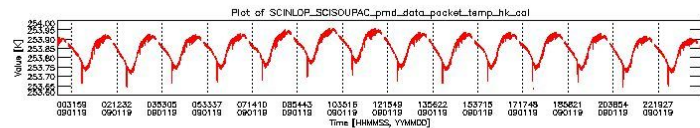
sciamachy_daily_report_level0_KSPT_L0_4303_N_20090119_3.PNG
