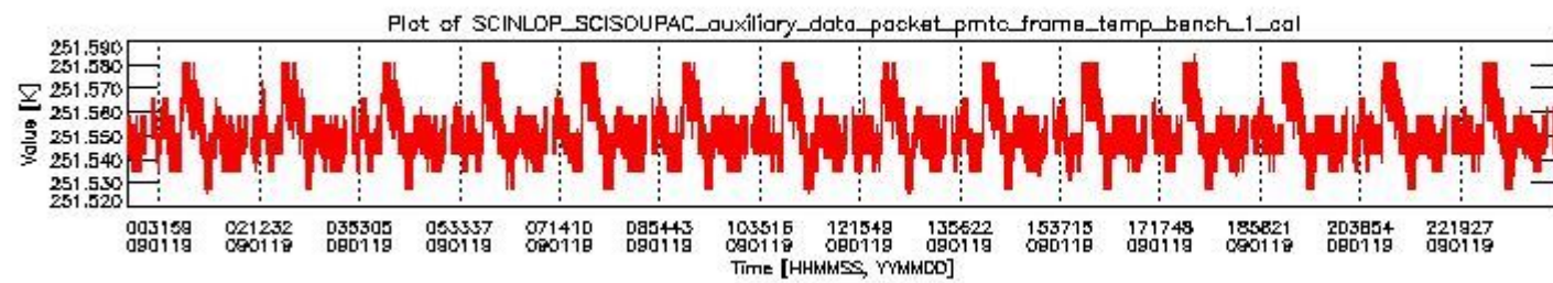
sciamachy_daily_report_level0_KSPT_L0_4303_N_20090119_0.PNG
