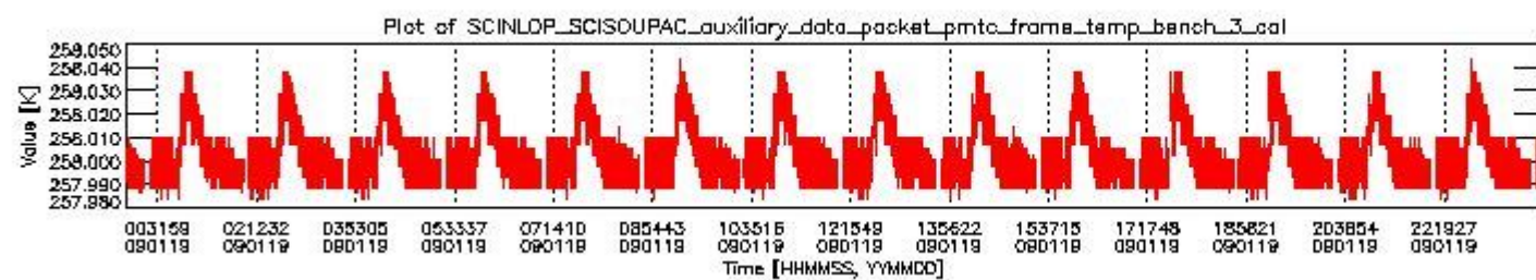
sciamachy_daily_report_level0_KSPT_L0_4303_N_20090119_2.PNG
