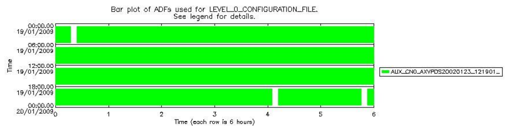
sciamachy_daily_report_level0_KSPT_L0_4303_N_20090119_7.PNG
