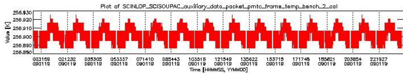
sciamachy_daily_report_level0_KSPT_L0_4303_N_20090119_1.PNG
