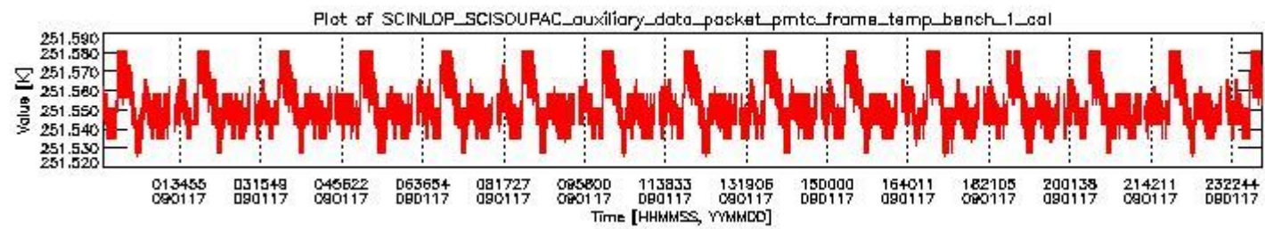
sciamachy_daily_report_level0_KSPT_L0_4303_N_20090117_0.PNG
