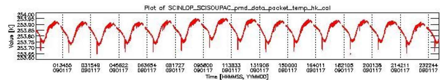
sciamachy_daily_report_level0_KSPT_L0_4303_N_20090117_3.PNG
