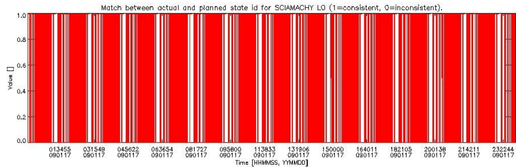
sciamachy_daily_report_level0_KSPT_L0_4303_N_20090117_5.PNG
