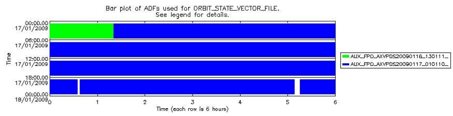
sciamachy_daily_report_level0_KSPT_L0_4303_N_20090117_8.PNG
