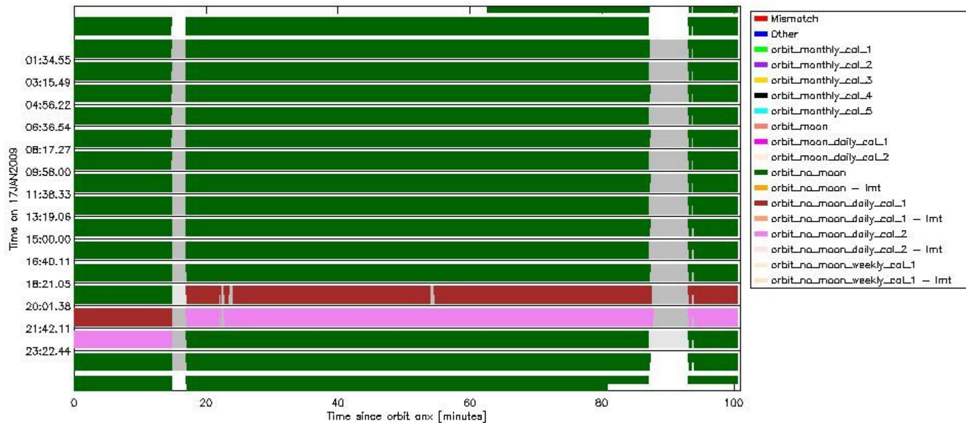
sciamachy_daily_report_level0_KSPT_L0_4303_N_20090117_6.PNG
