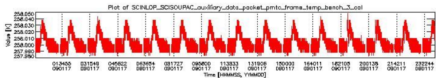
sciamachy_daily_report_level0_KSPT_L0_4303_N_20090117_2.PNG
