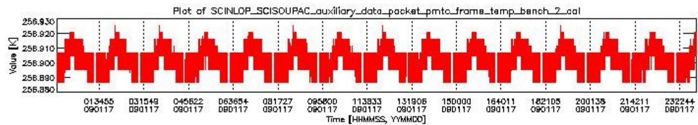
sciamachy_daily_report_level0_KSPT_L0_4303_N_20090117_1.PNG
