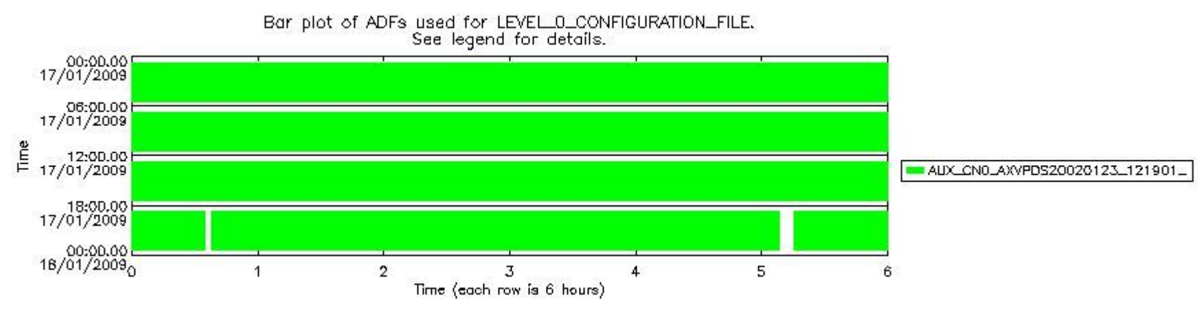
sciamachy_daily_report_level0_KSPT_L0_4303_N_20090117_7.PNG
