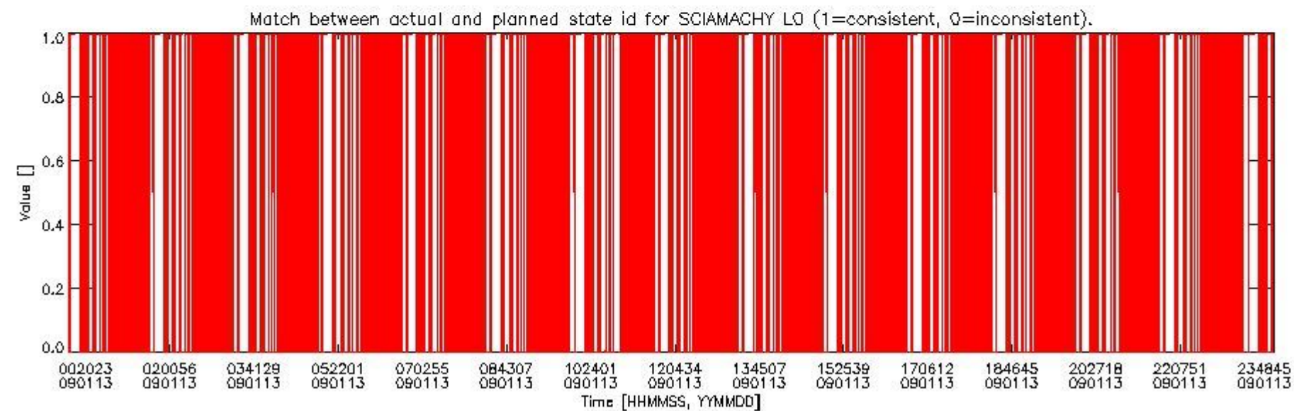
sciamachy_daily_report_level0_KSPT_L0_4303_N_20090113_5.PNG
