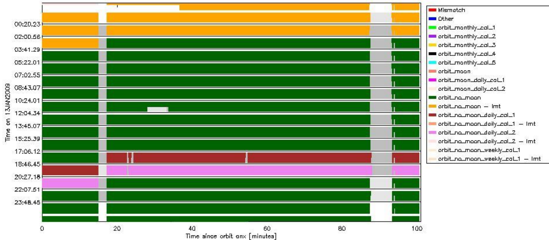
sciamachy_daily_report_level0_KSPT_L0_4303_N_20090113_6.PNG
