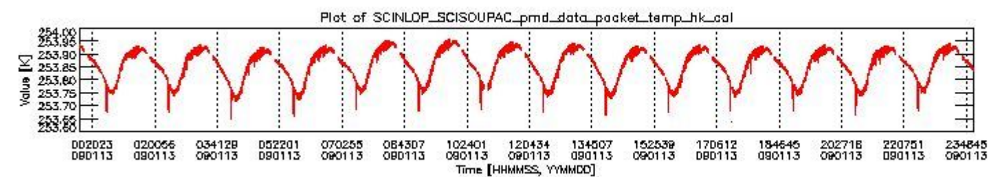
sciamachy_daily_report_level0_KSPT_L0_4303_N_20090113_3.PNG
