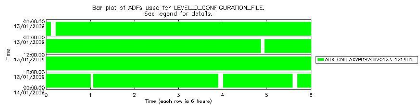
sciamachy_daily_report_level0_KSPT_L0_4303_N_20090113_7.PNG
