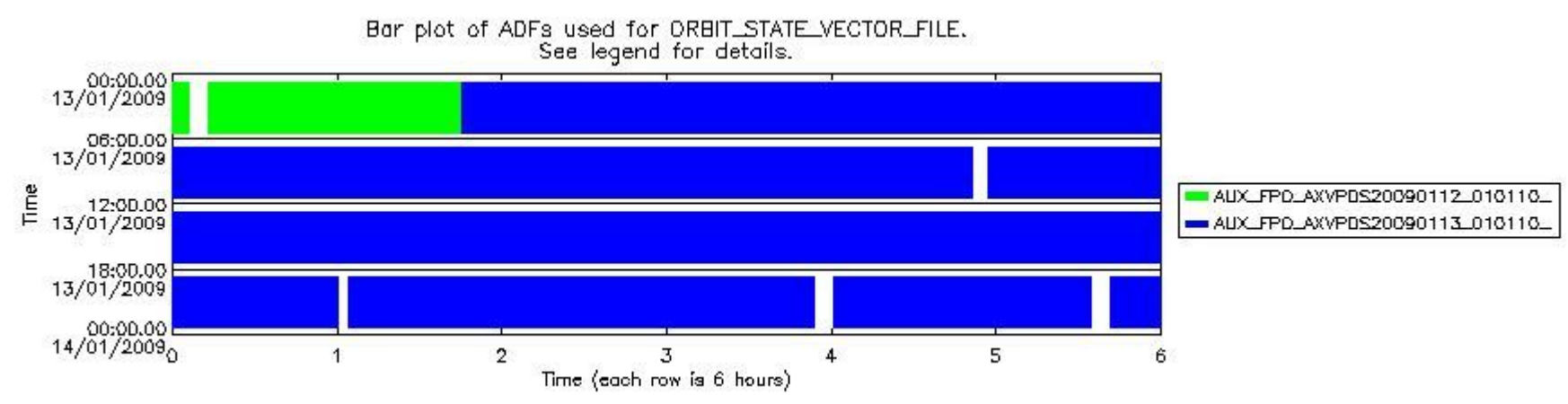
sciamachy_daily_report_level0_KSPT_L0_4303_N_20090113_8.PNG
