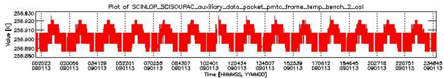
sciamachy_daily_report_level0_KSPT_L0_4303_N_20090113_1.PNG
