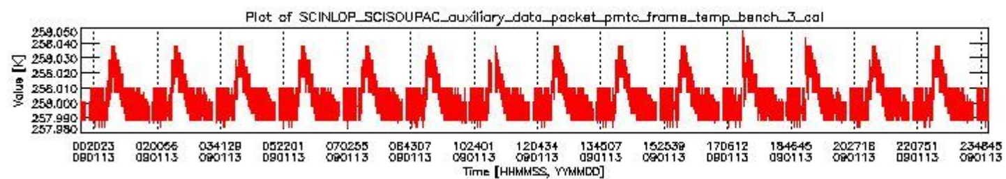
sciamachy_daily_report_level0_KSPT_L0_4303_N_20090113_2.PNG
