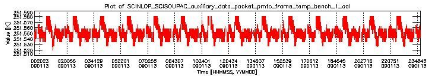
sciamachy_daily_report_level0_KSPT_L0_4303_N_20090113_0.PNG
