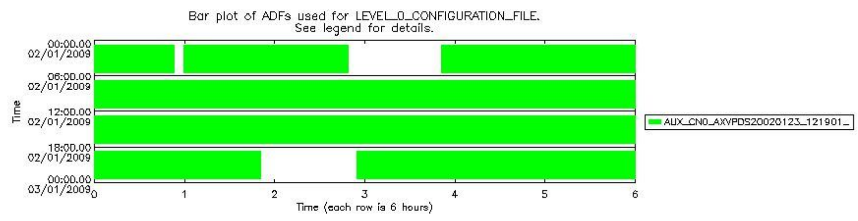
sciamachy_daily_report_level0_KSPT_L0_4303_N_20090102_6.PNG
