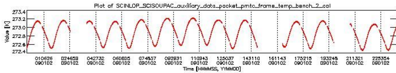
sciamachy_daily_report_level0_KSPT_L0_4303_N_20090102_1.PNG
