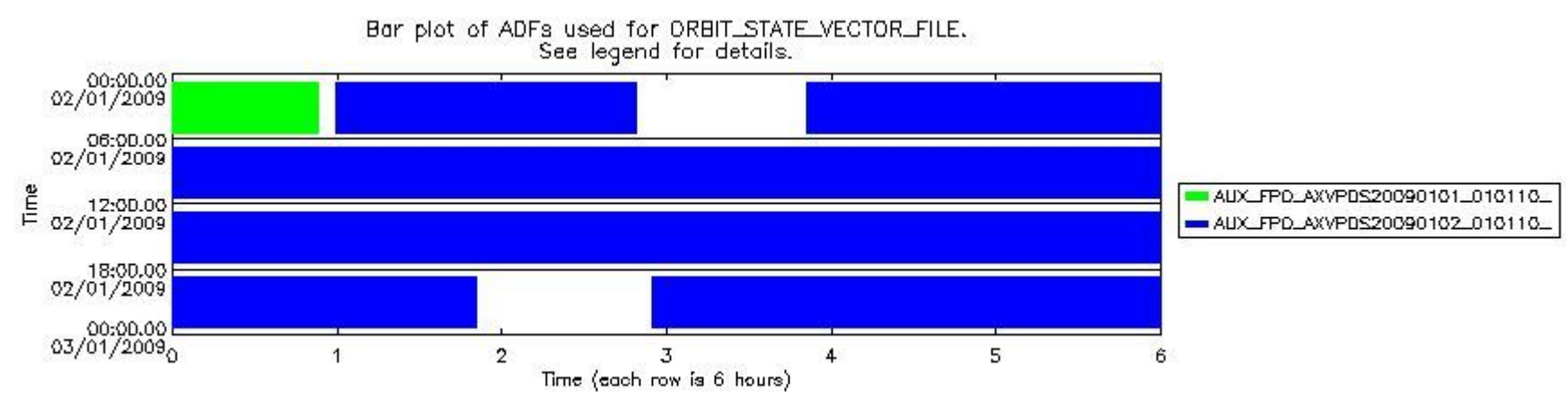
sciamachy_daily_report_level0_KSPT_L0_4303_N_20090102_7.PNG
