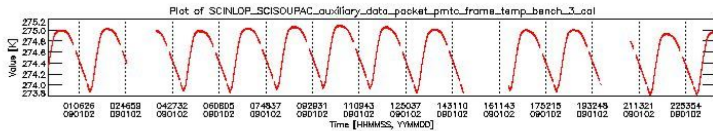
sciamachy_daily_report_level0_KSPT_L0_4303_N_20090102_2.PNG
