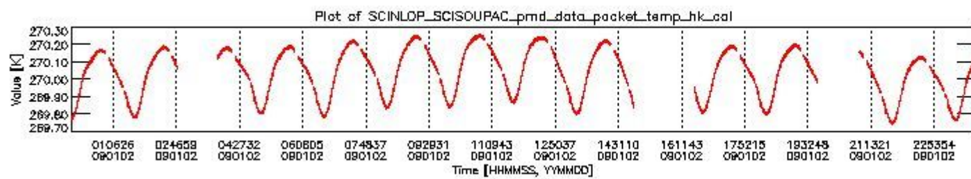
sciamachy_daily_report_level0_KSPT_L0_4303_N_20090102_3.PNG
