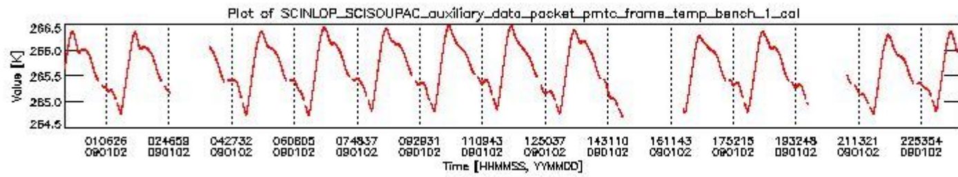
sciamachy_daily_report_level0_KSPT_L0_4303_N_20090102_0.PNG
