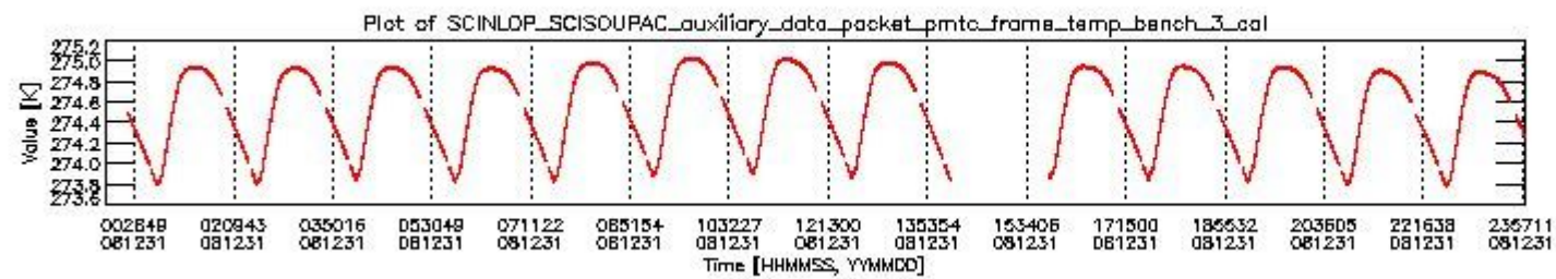
sciamachy_daily_report_level0_KSPT_L0_4303_N_20081231_2.PNG
