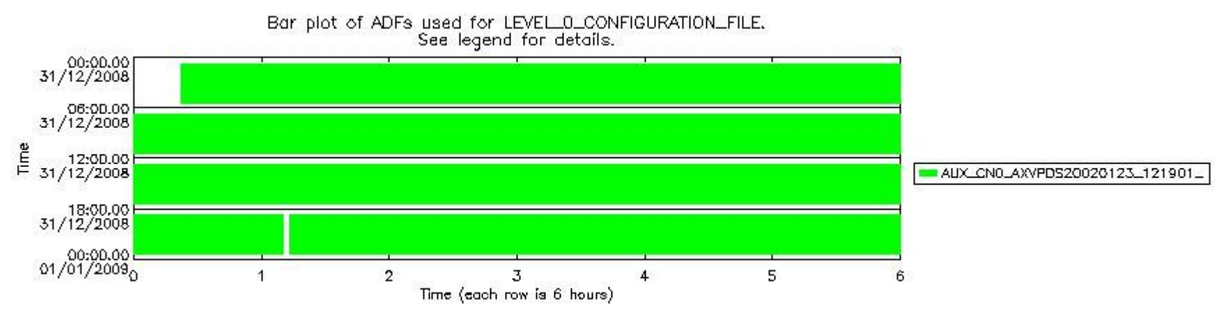
sciamachy_daily_report_level0_KSPT_L0_4303_N_20081231_6.PNG
