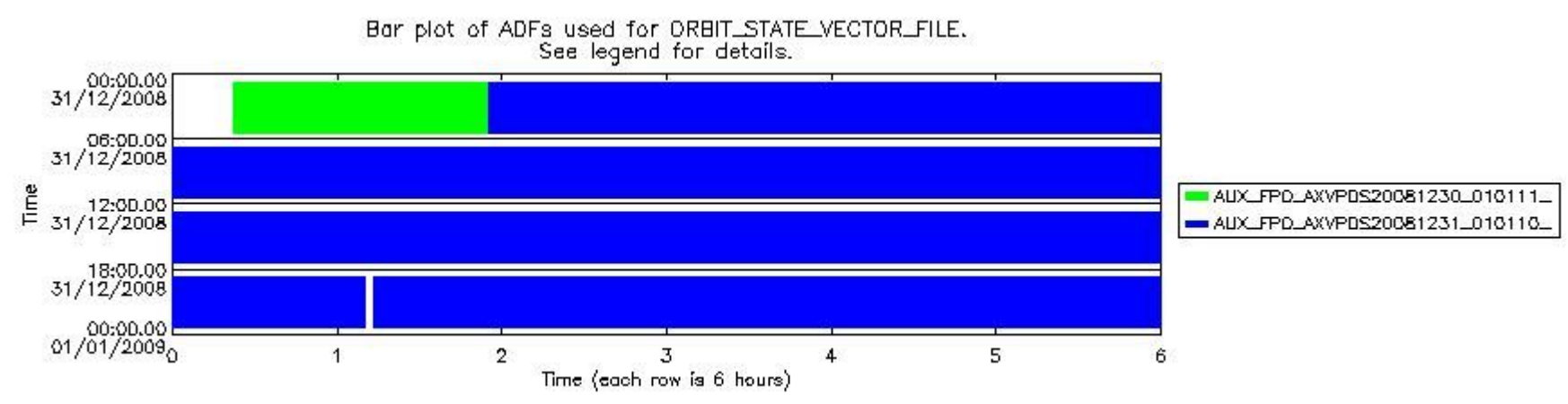
sciamachy_daily_report_level0_KSPT_L0_4303_N_20081231_7.PNG
