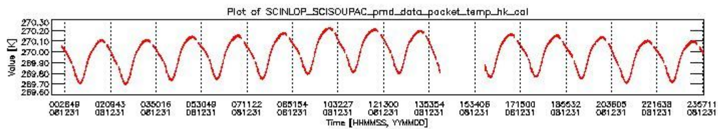
sciamachy_daily_report_level0_KSPT_L0_4303_N_20081231_3.PNG
