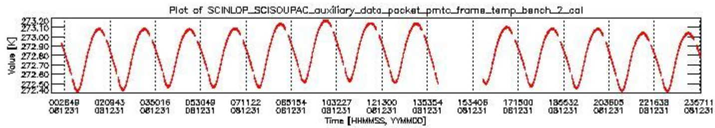
sciamachy_daily_report_level0_KSPT_L0_4303_N_20081231_1.PNG
