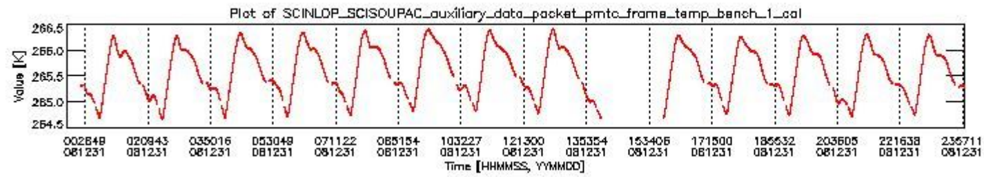
sciamachy_daily_report_level0_KSPT_L0_4303_N_20081231_0.PNG
