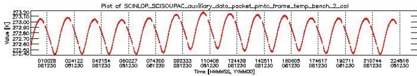
sciamachy_daily_report_level0_KSPT_L0_4303_N_20081230_1.PNG
