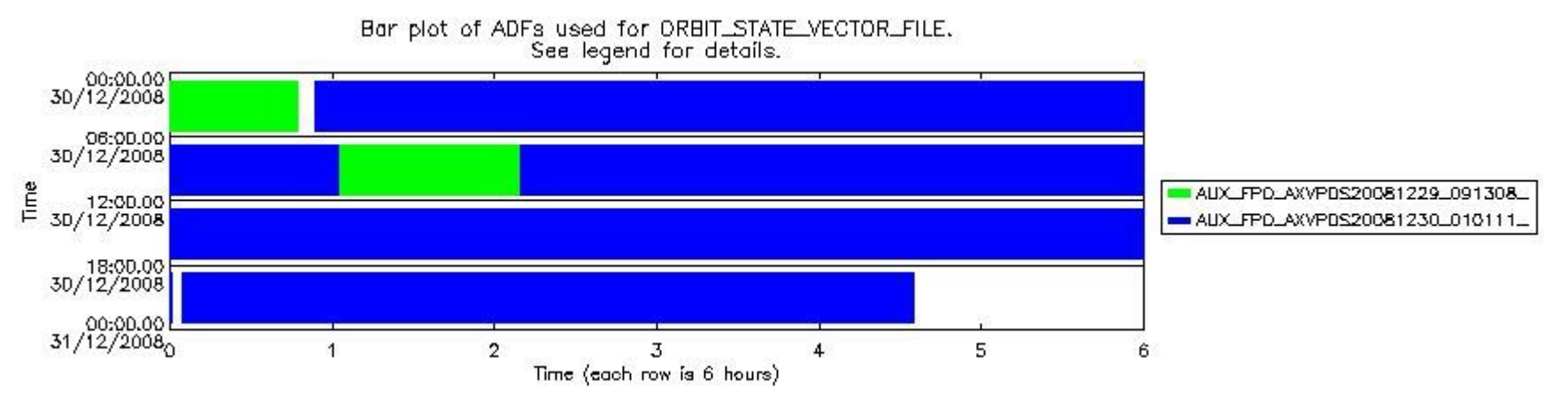
sciamachy_daily_report_level0_KSPT_L0_4303_N_20081230_7.PNG
