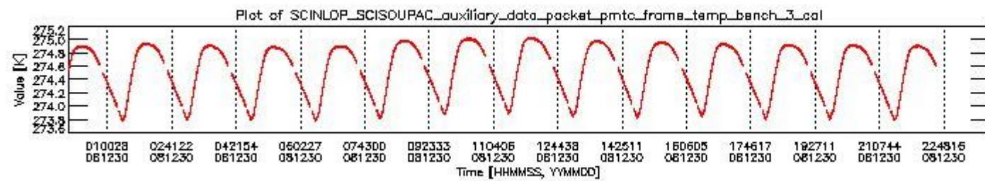
sciamachy_daily_report_level0_KSPT_L0_4303_N_20081230_2.PNG
