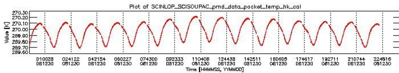
sciamachy_daily_report_level0_KSPT_L0_4303_N_20081230_3.PNG
