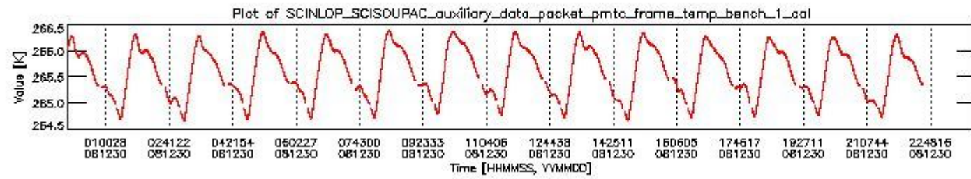
sciamachy_daily_report_level0_KSPT_L0_4303_N_20081230_0.PNG
