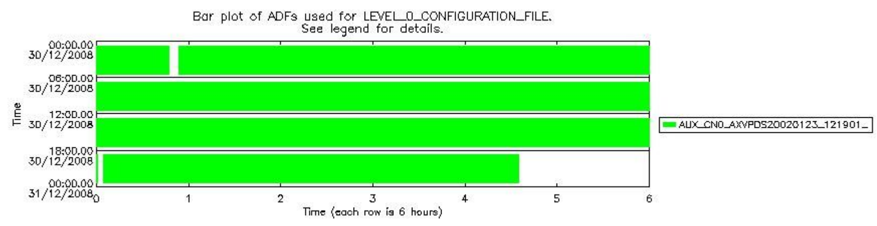
sciamachy_daily_report_level0_KSPT_L0_4303_N_20081230_6.PNG
