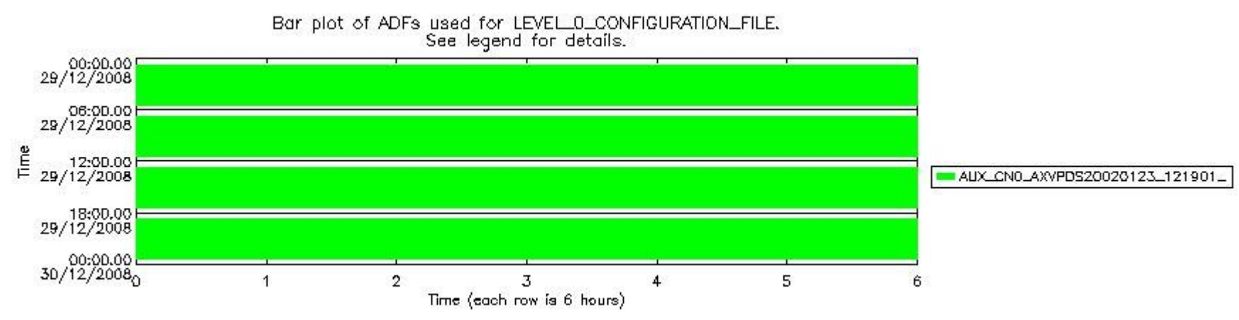
sciamachy_daily_report_level0_KSPT_L0_4303_N_20081229_6.PNG
