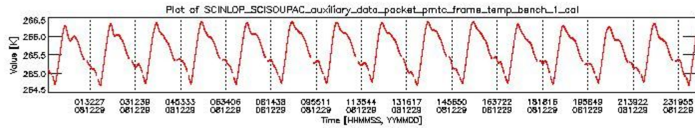
sciamachy_daily_report_level0_KSPT_L0_4303_N_20081229_0.PNG
