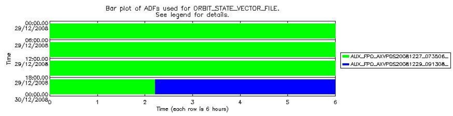
sciamachy_daily_report_level0_KSPT_L0_4303_N_20081229_7.PNG
