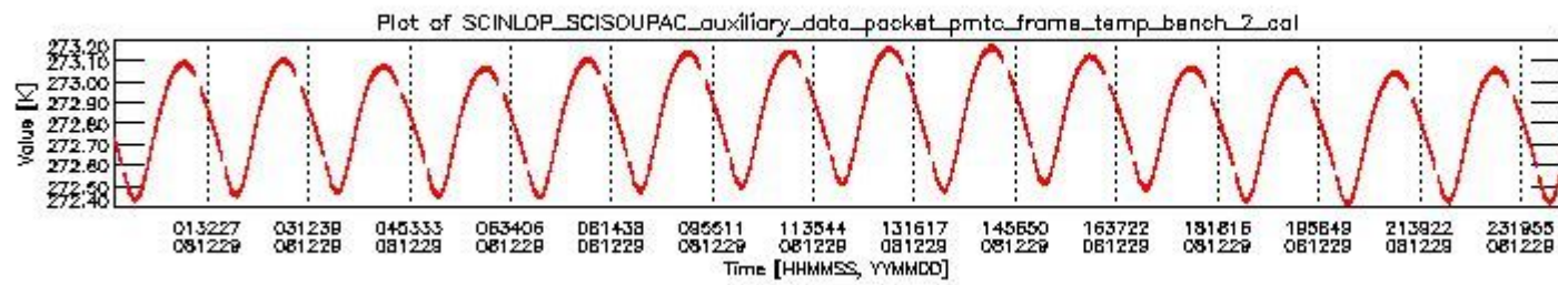
sciamachy_daily_report_level0_KSPT_L0_4303_N_20081229_1.PNG
