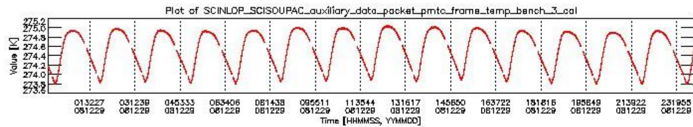
sciamachy_daily_report_level0_KSPT_L0_4303_N_20081229_2.PNG
