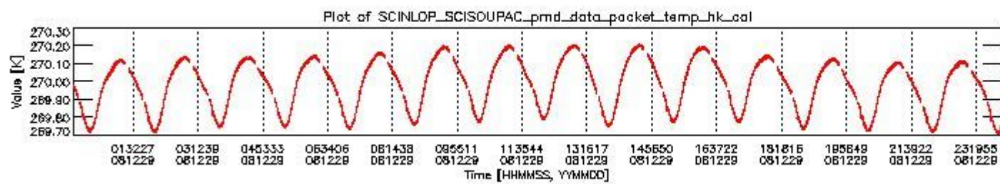
sciamachy_daily_report_level0_KSPT_L0_4303_N_20081229_3.PNG
