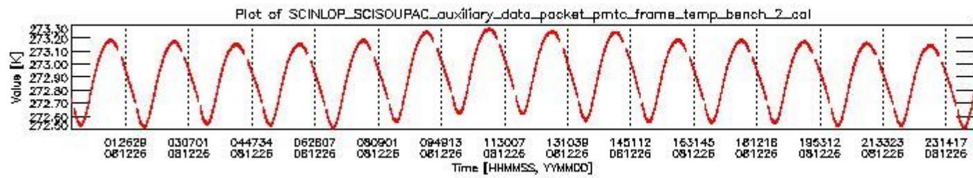
sciamachy_daily_report_level0_KSPT_L0_4303_N_20081226_1.PNG
