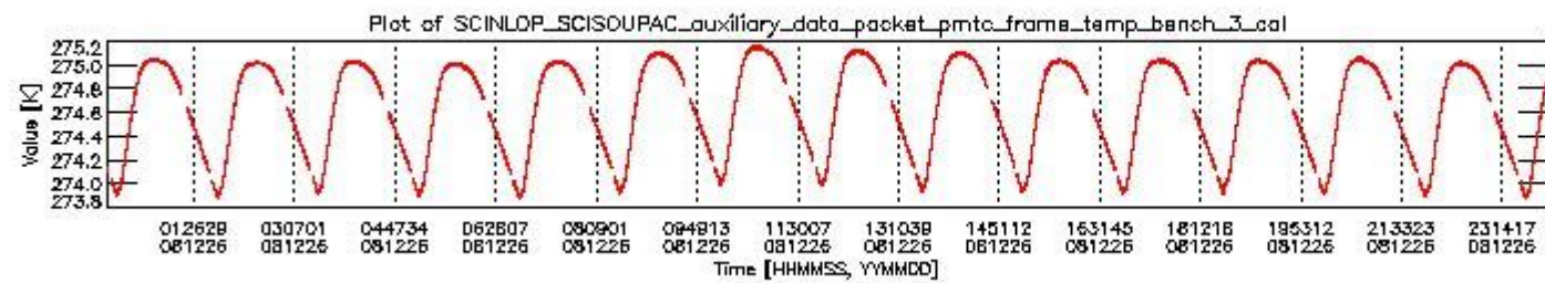
sciamachy_daily_report_level0_KSPT_L0_4303_N_20081226_2.PNG
