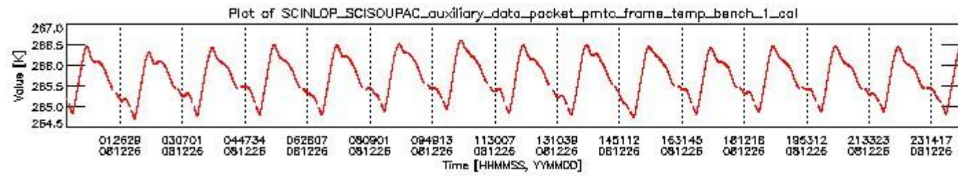
sciamachy_daily_report_level0_KSPT_L0_4303_N_20081226_0.PNG
