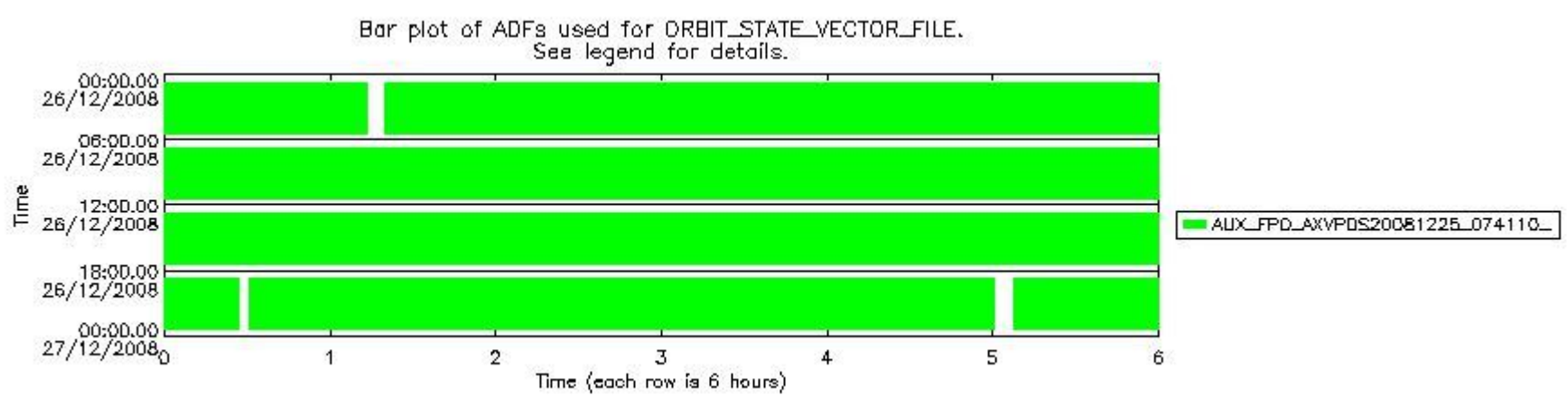
sciamachy_daily_report_level0_KSPT_L0_4303_N_20081226_7.PNG
