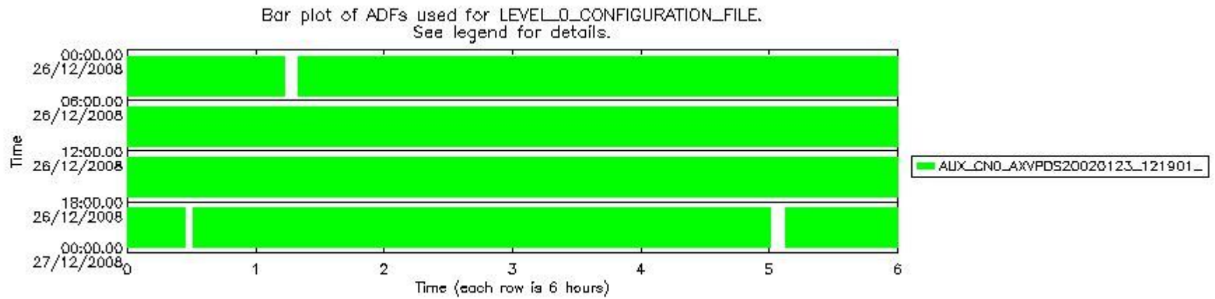
sciamachy_daily_report_level0_KSPT_L0_4303_N_20081226_6.PNG
