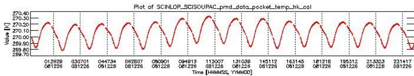
sciamachy_daily_report_level0_KSPT_L0_4303_N_20081226_3.PNG
