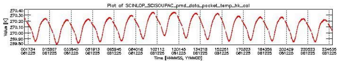
sciamachy_daily_report_level0_KSPT_L0_4303_N_20081225_3.PNG
