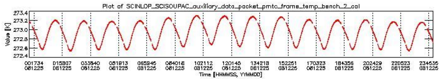
sciamachy_daily_report_level0_KSPT_L0_4303_N_20081225_1.PNG
