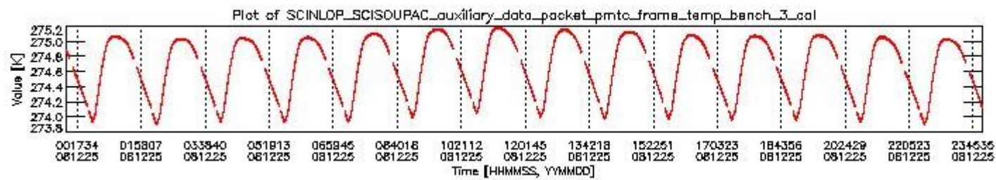
sciamachy_daily_report_level0_KSPT_L0_4303_N_20081225_2.PNG
