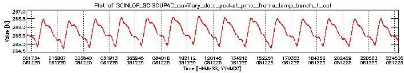
sciamachy_daily_report_level0_KSPT_L0_4303_N_20081225_0.PNG
