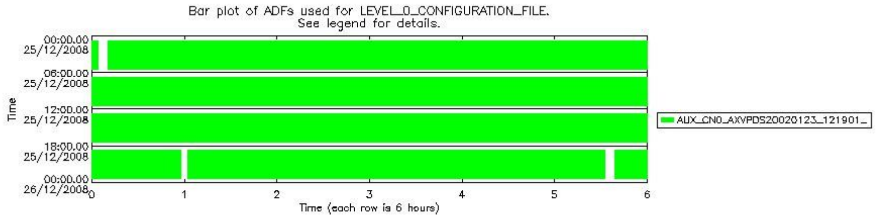
sciamachy_daily_report_level0_KSPT_L0_4303_N_20081225_6.PNG
