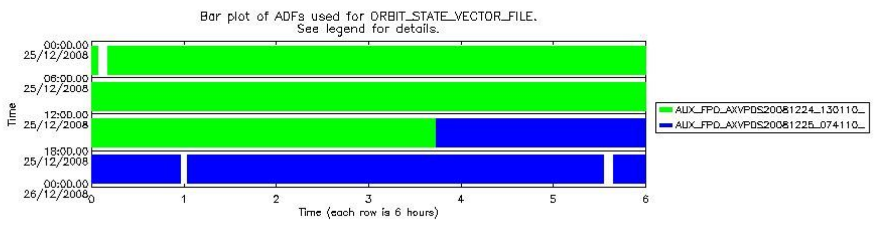
sciamachy_daily_report_level0_KSPT_L0_4303_N_20081225_7.PNG
