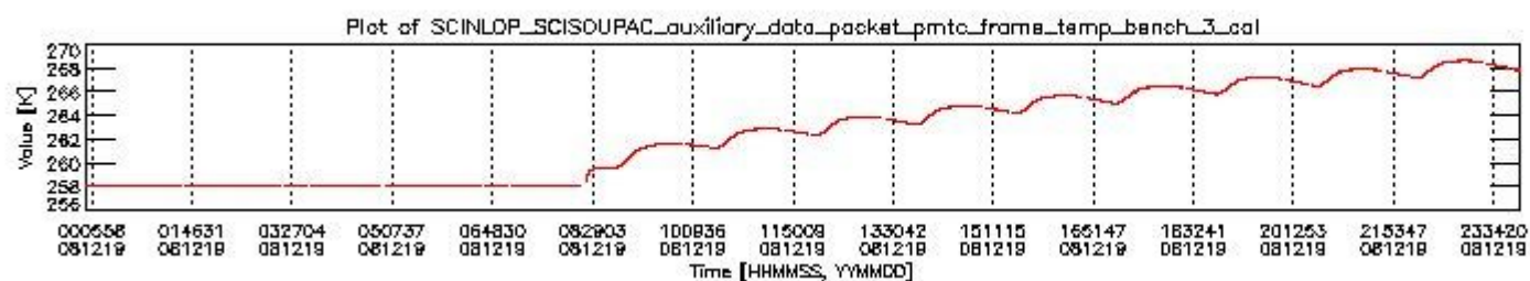
sciamachy_daily_report_level0_KSPT_L0_4303_N_20081219_2.PNG
