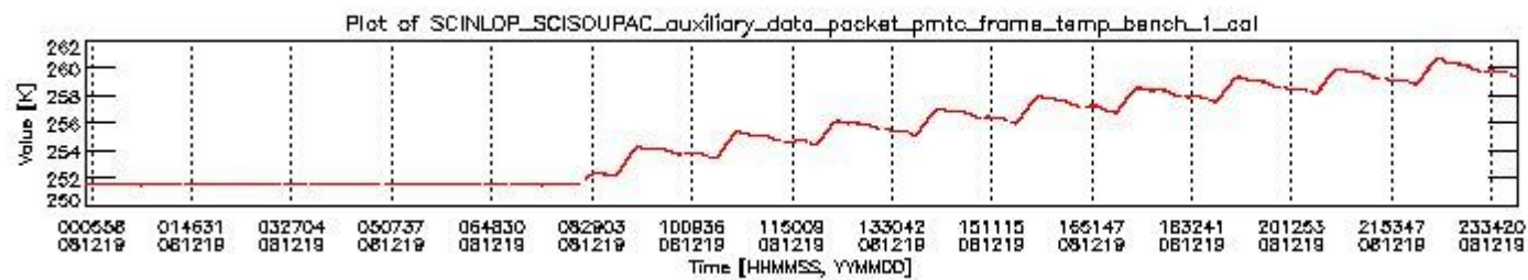
sciamachy_daily_report_level0_KSPT_L0_4303_N_20081219_0.PNG
