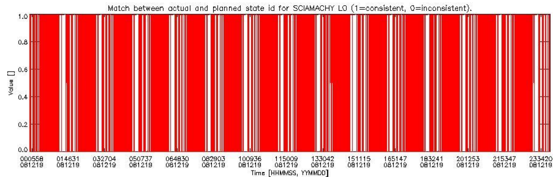
sciamachy_daily_report_level0_KSPT_L0_4303_N_20081219_5.PNG
