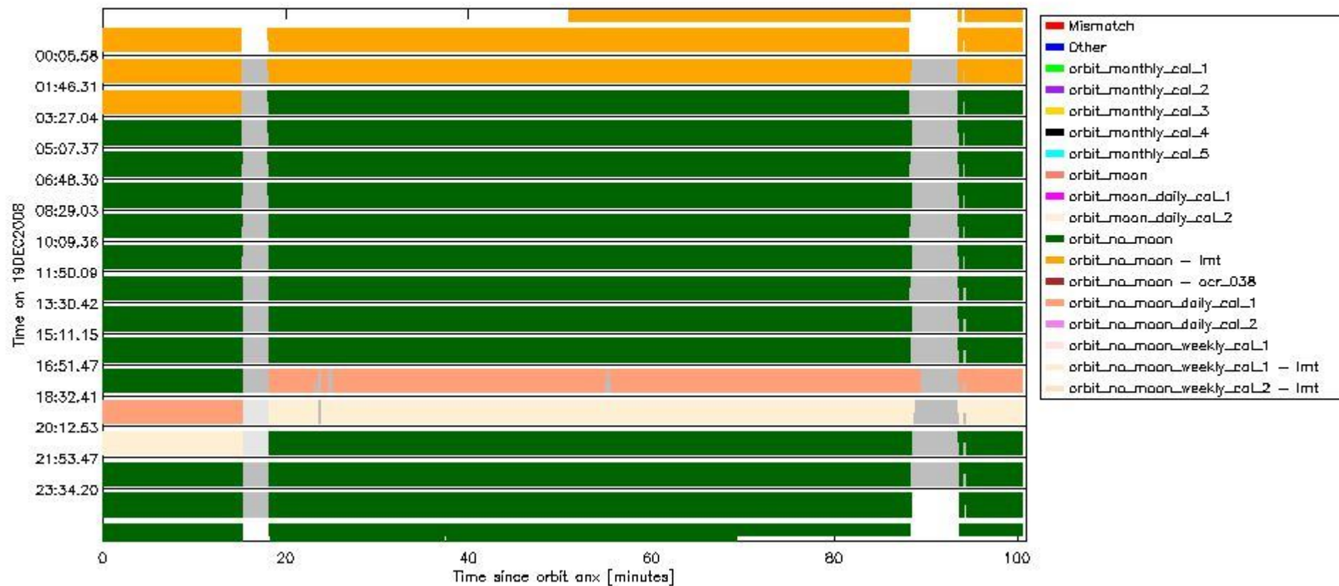
sciamachy_daily_report_level0_KSPT_L0_4303_N_20081219_6.PNG
