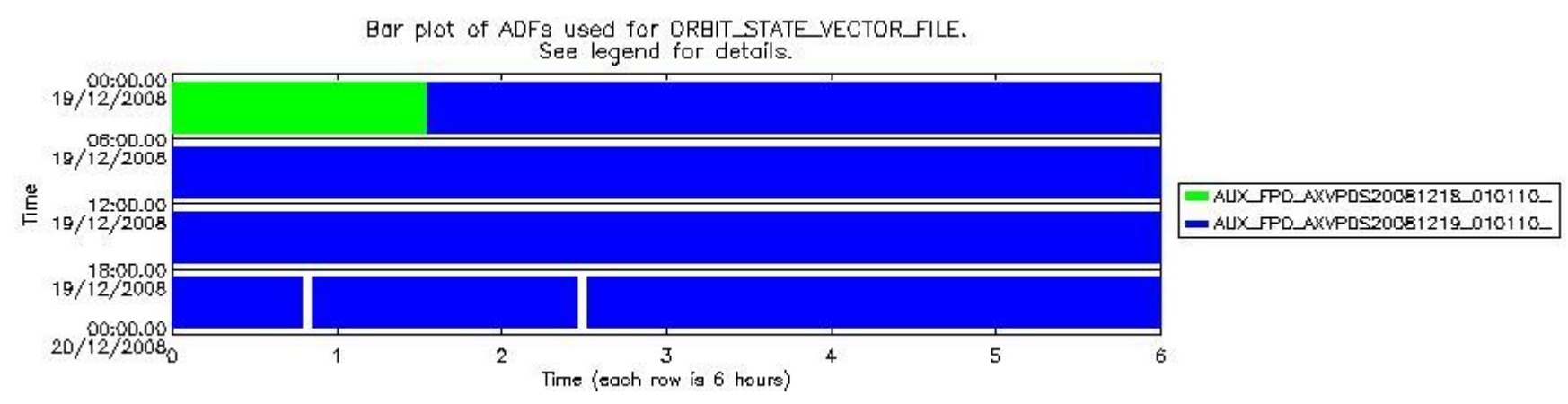
sciamachy_daily_report_level0_KSPT_L0_4303_N_20081219_8.PNG
