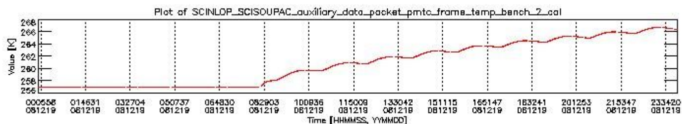
sciamachy_daily_report_level0_KSPT_L0_4303_N_20081219_1.PNG
