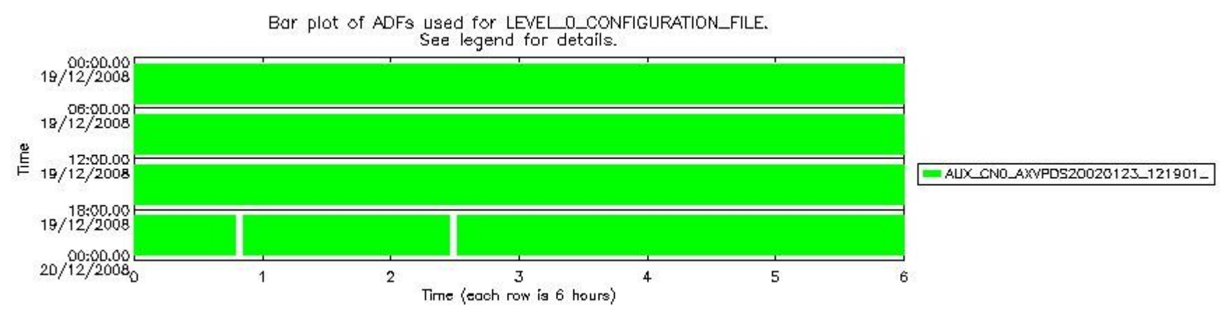
sciamachy_daily_report_level0_KSPT_L0_4303_N_20081219_7.PNG
