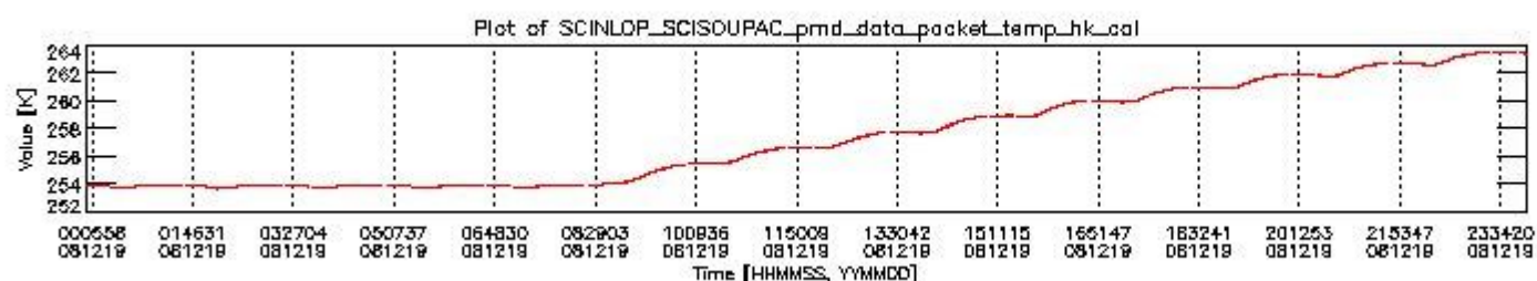
sciamachy_daily_report_level0_KSPT_L0_4303_N_20081219_3.PNG
