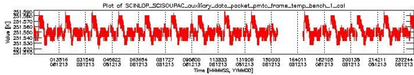
sciamachy_daily_report_level0_KSPT_L0_4303_N_20081213_0.PNG
