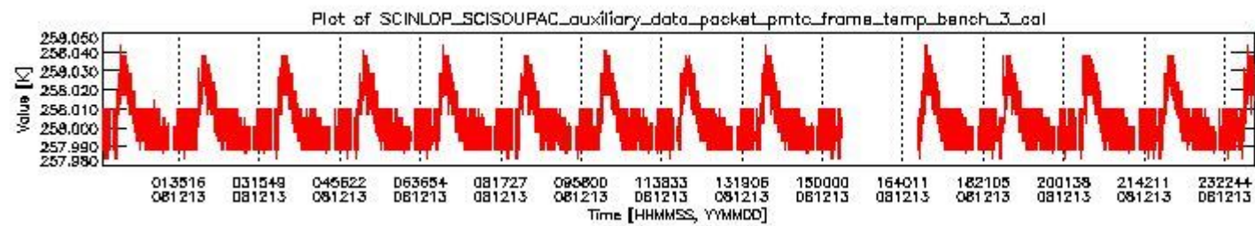
sciamachy_daily_report_level0_KSPT_L0_4303_N_20081213_2.PNG
