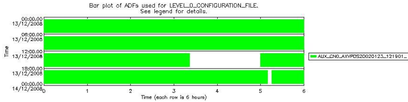
sciamachy_daily_report_level0_KSPT_L0_4303_N_20081213_6.PNG
