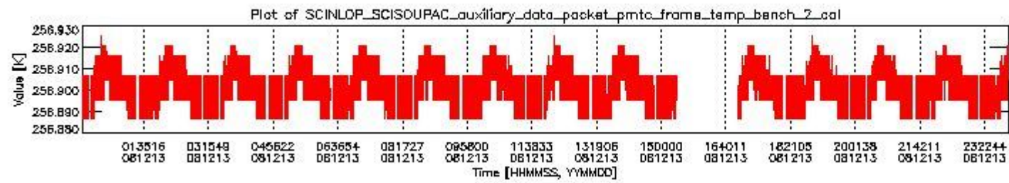
sciamachy_daily_report_level0_KSPT_L0_4303_N_20081213_1.PNG
