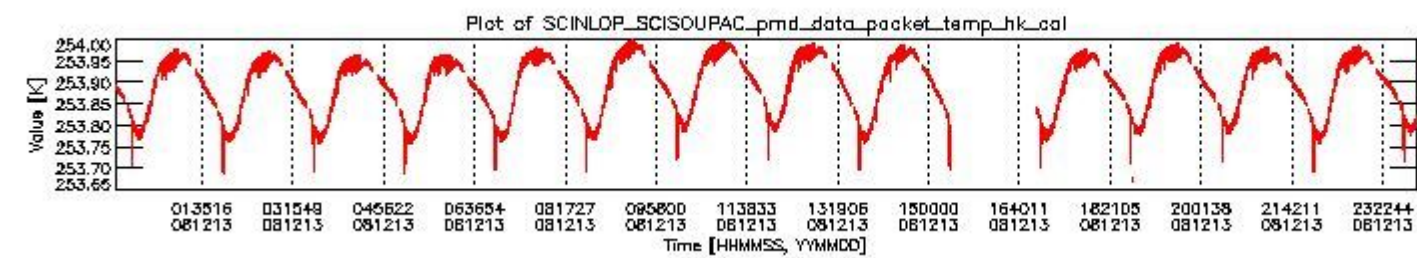
sciamachy_daily_report_level0_KSPT_L0_4303_N_20081213_3.PNG
