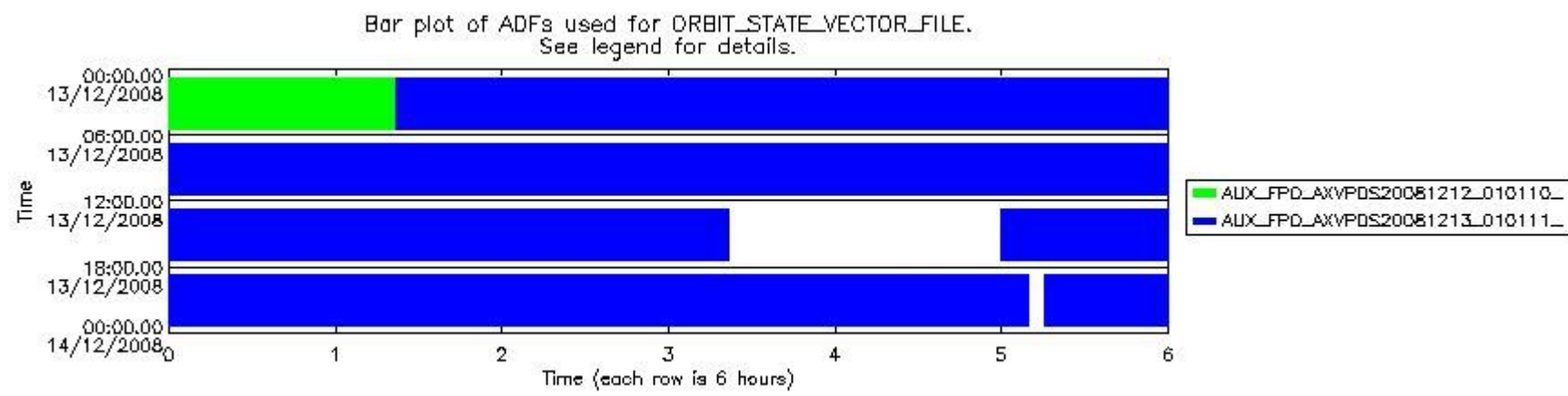
sciamachy_daily_report_level0_KSPT_L0_4303_N_20081213_7.PNG
