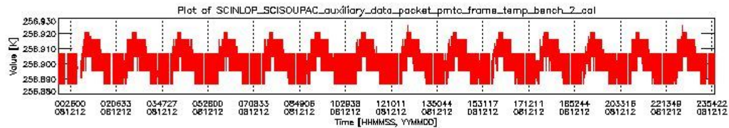
sciamachy_daily_report_level0_KSPT_L0_4303_N_20081212_1.PNG
