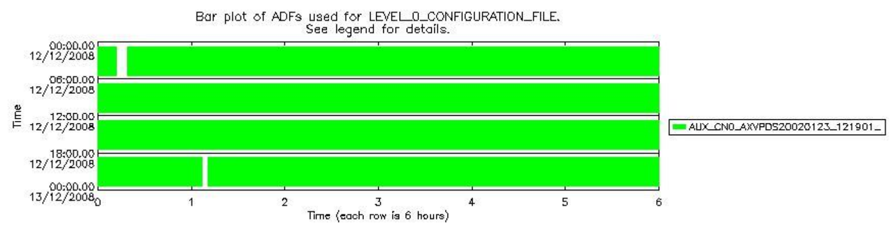
sciamachy_daily_report_level0_KSPT_L0_4303_N_20081212_7.PNG
