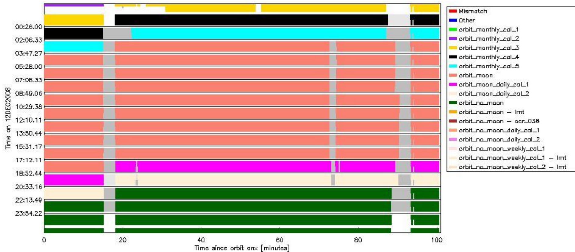
sciamachy_daily_report_level0_KSPT_L0_4303_N_20081212_6.PNG
