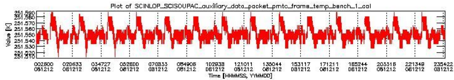
sciamachy_daily_report_level0_KSPT_L0_4303_N_20081212_0.PNG
