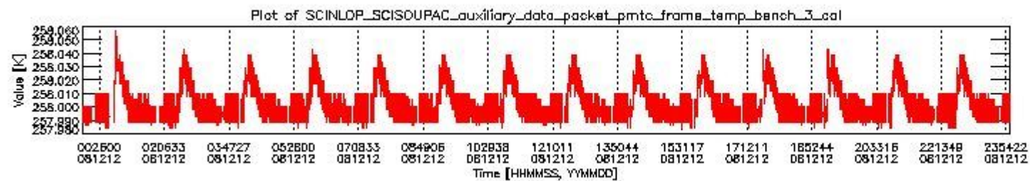
sciamachy_daily_report_level0_KSPT_L0_4303_N_20081212_2.PNG
