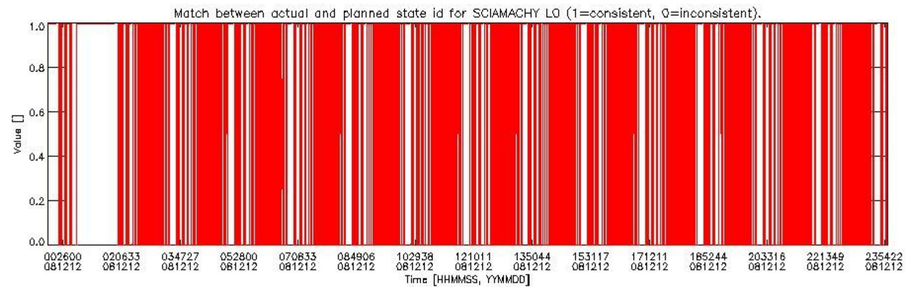
sciamachy_daily_report_level0_KSPT_L0_4303_N_20081212_5.PNG
