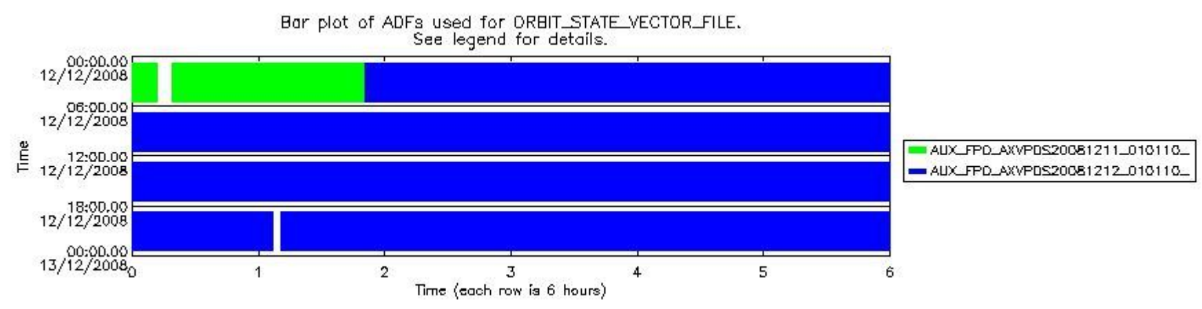
sciamachy_daily_report_level0_KSPT_L0_4303_N_20081212_8.PNG
