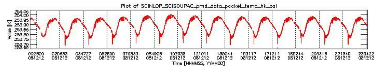
sciamachy_daily_report_level0_KSPT_L0_4303_N_20081212_3.PNG
