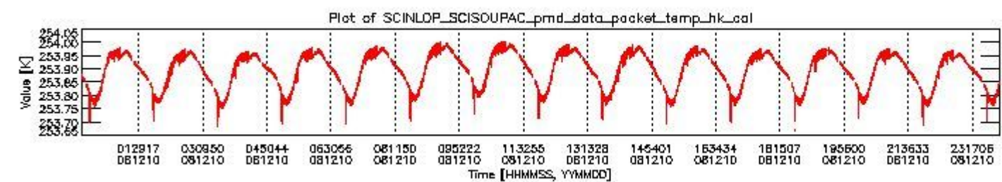
sciamachy_daily_report_level0_KSPT_L0_4303_N_20081210_3.PNG
