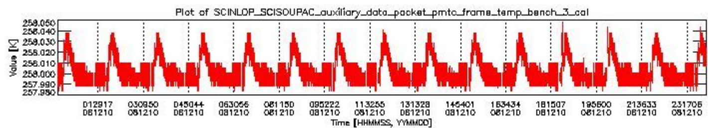
sciamachy_daily_report_level0_KSPT_L0_4303_N_20081210_2.PNG
