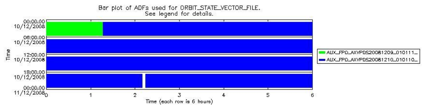
sciamachy_daily_report_level0_KSPT_L0_4303_N_20081210_7.PNG
