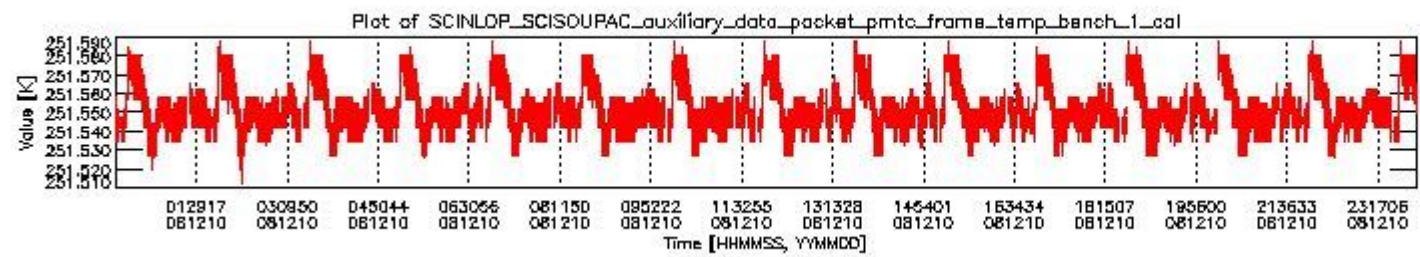
sciamachy_daily_report_level0_KSPT_L0_4303_N_20081210_0.PNG
