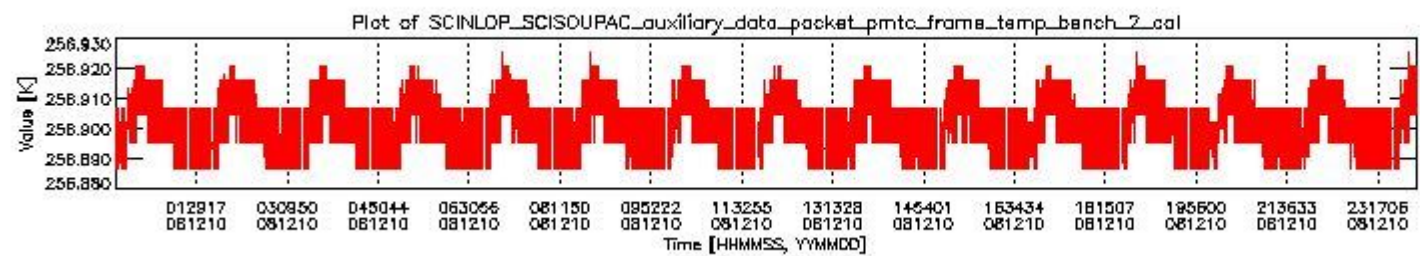
sciamachy_daily_report_level0_KSPT_L0_4303_N_20081210_1.PNG
