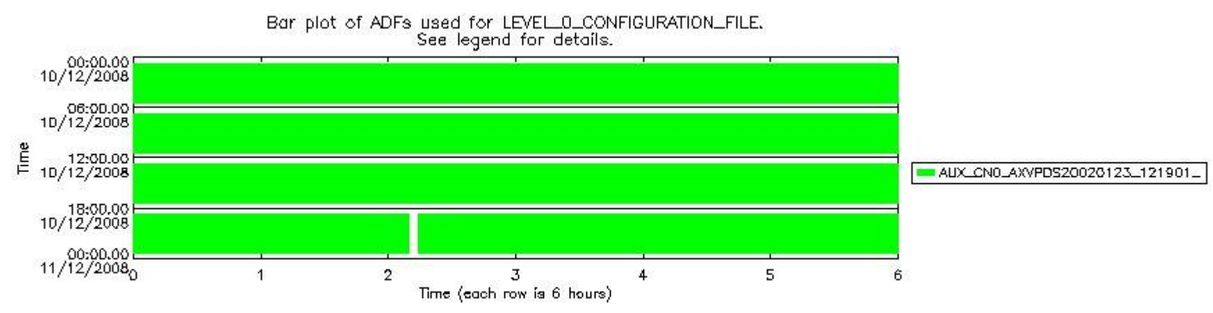
sciamachy_daily_report_level0_KSPT_L0_4303_N_20081210_6.PNG
