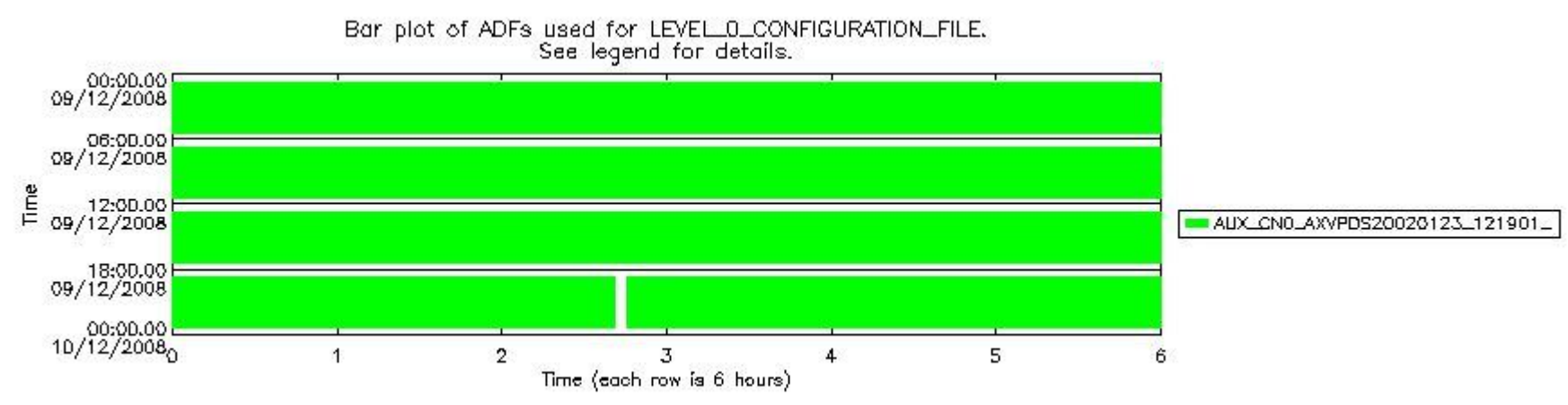
sciamachy_daily_report_level0_KSPT_L0_4303_N_20081209_7.PNG
