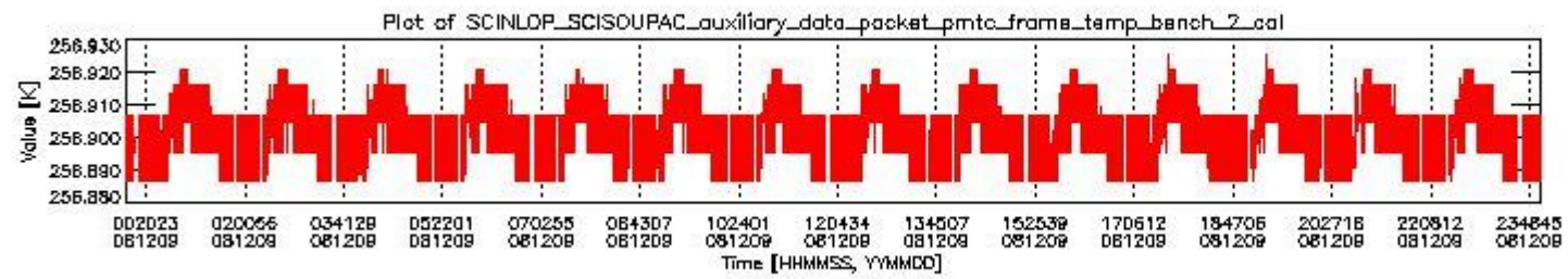
sciamachy_daily_report_level0_KSPT_L0_4303_N_20081209_1.PNG
