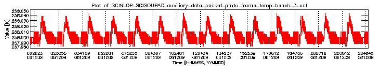
sciamachy_daily_report_level0_KSPT_L0_4303_N_20081209_2.PNG
