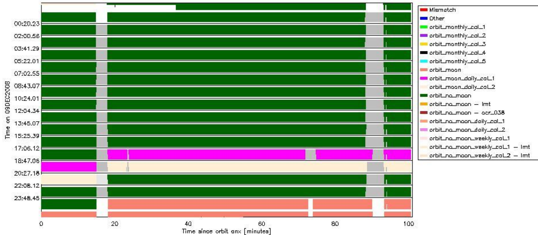
sciamachy_daily_report_level0_KSPT_L0_4303_N_20081209_6.PNG
