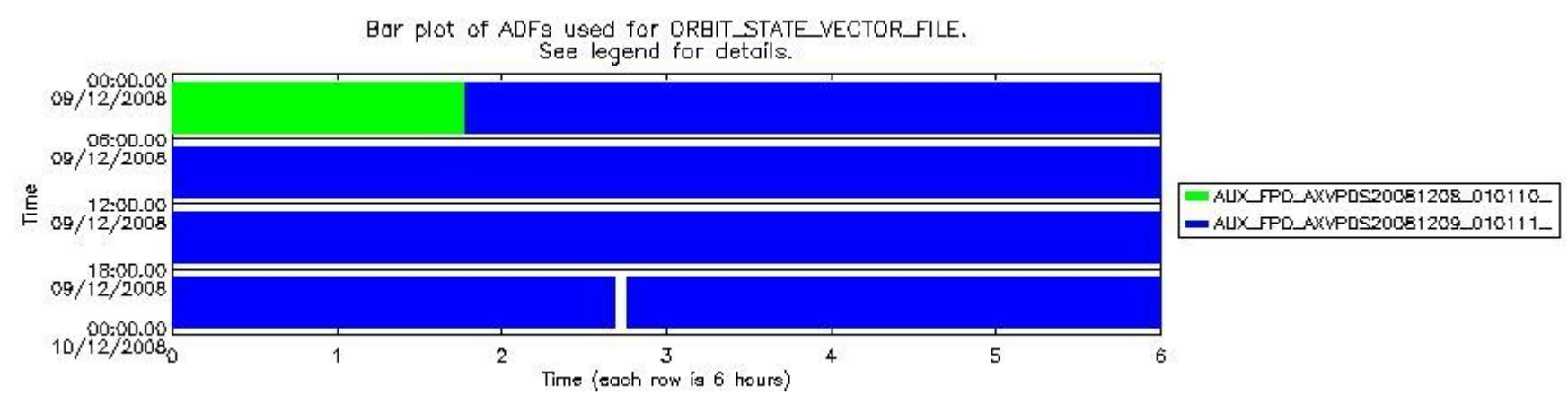
sciamachy_daily_report_level0_KSPT_L0_4303_N_20081209_8.PNG
