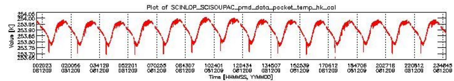
sciamachy_daily_report_level0_KSPT_L0_4303_N_20081209_3.PNG
