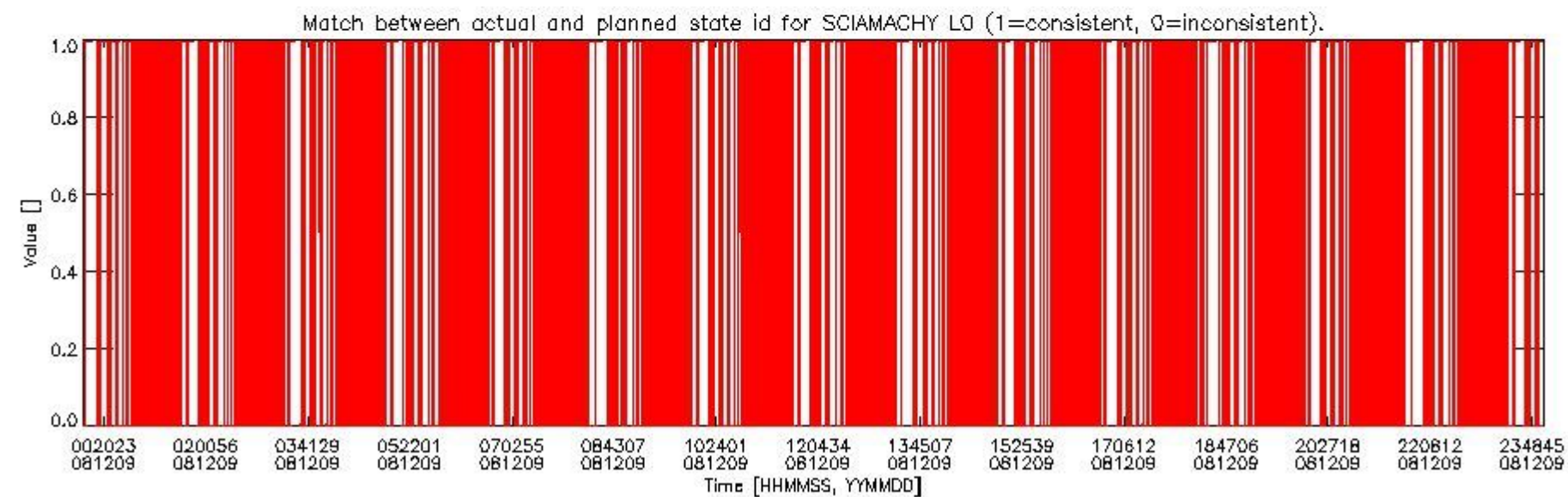
sciamachy_daily_report_level0_KSPT_L0_4303_N_20081209_5.PNG
