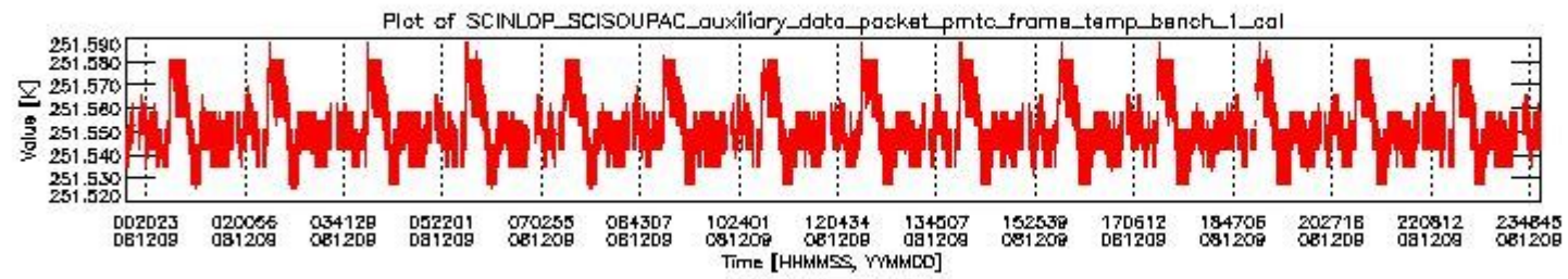
sciamachy_daily_report_level0_KSPT_L0_4303_N_20081209_0.PNG
