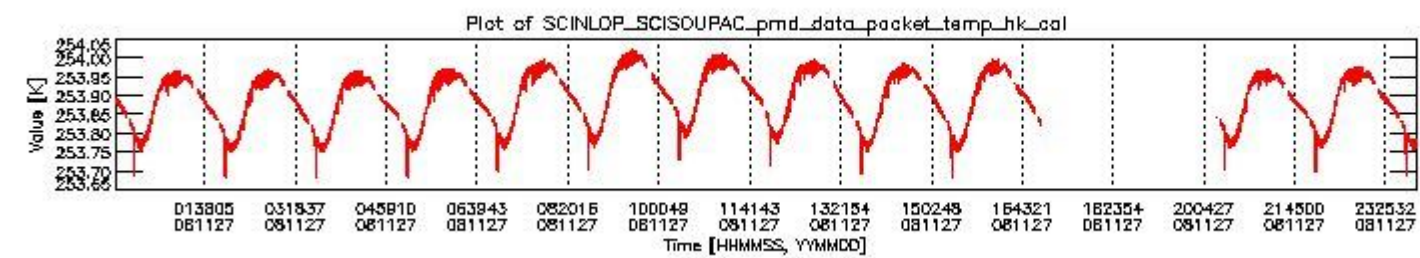
sciamachy_daily_report_level0_KSPT_L0_4303_N_20081127_3.PNG
