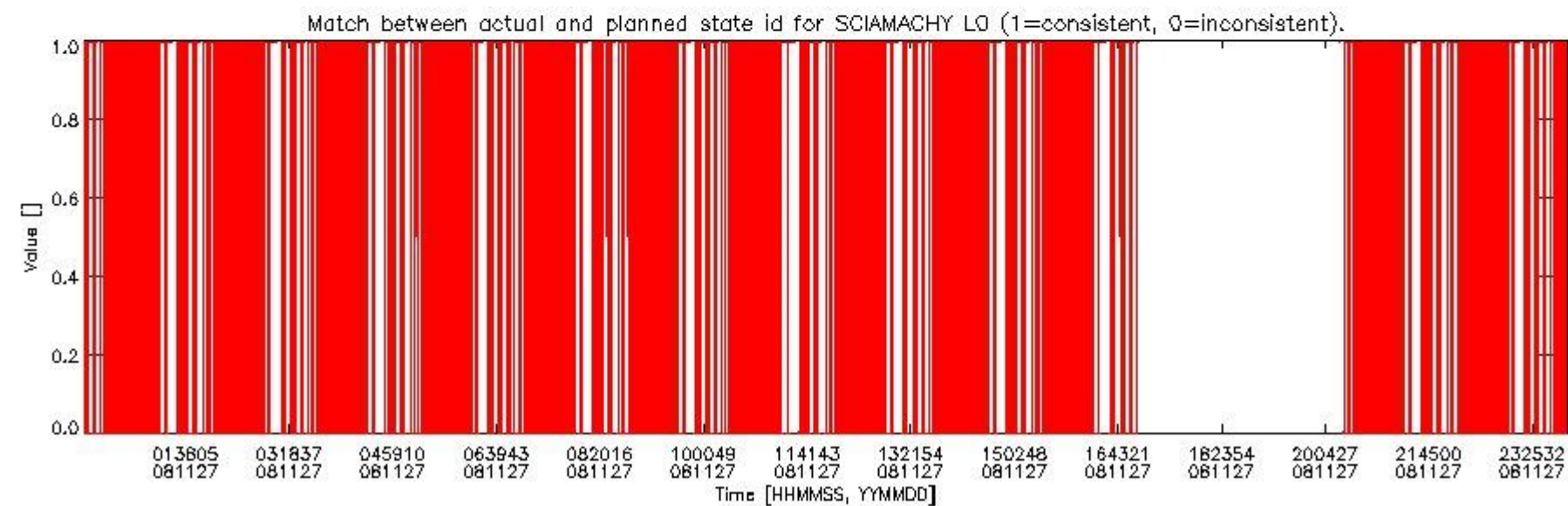
sciamachy_daily_report_level0_KSPT_L0_4303_N_20081127_5.PNG
