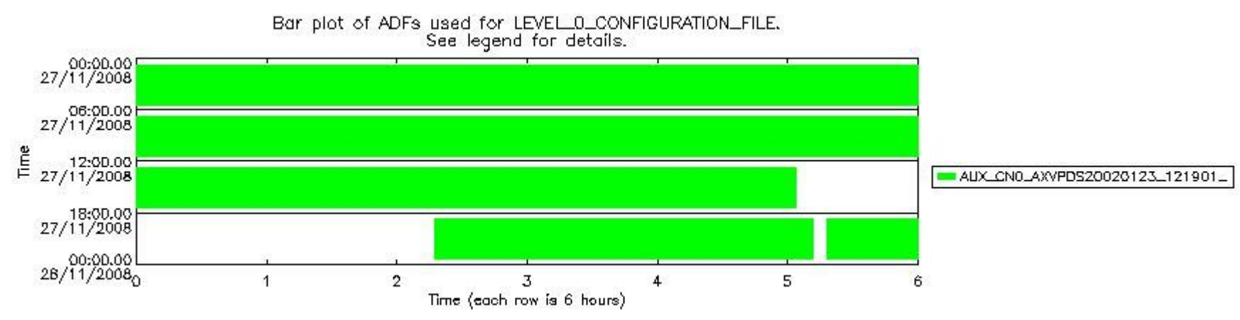
sciamachy_daily_report_level0_KSPT_L0_4303_N_20081127_7.PNG
