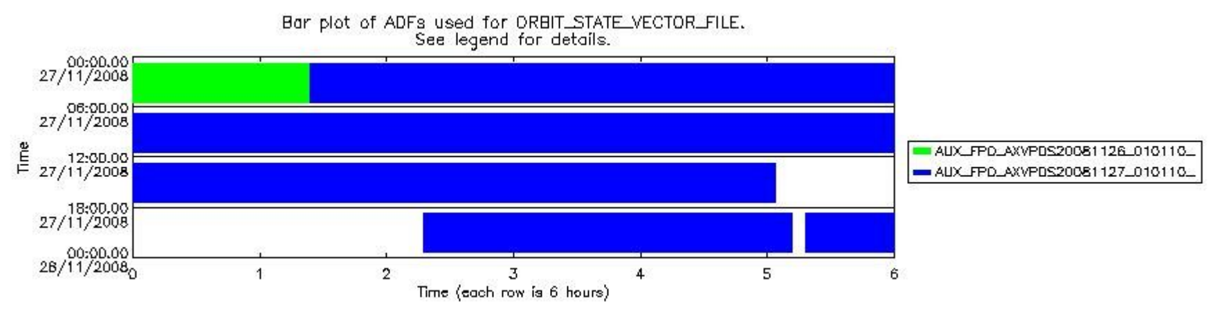
sciamachy_daily_report_level0_KSPT_L0_4303_N_20081127_8.PNG
