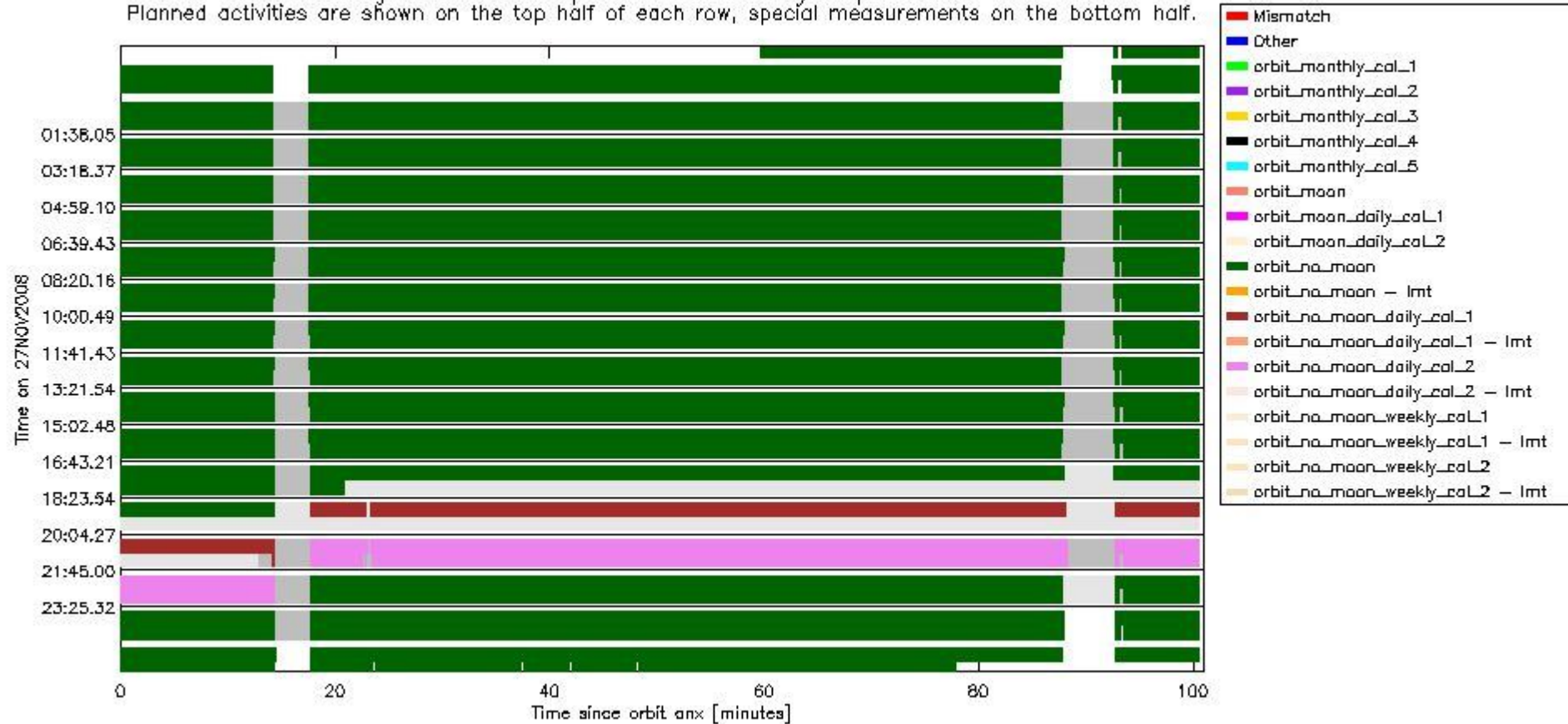
sciamachy_daily_report_level0_KSPT_L0_4303_N_20081127_6.PNG
