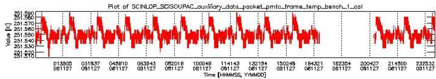
sciamachy_daily_report_level0_KSPT_L0_4303_N_20081127_0.PNG
