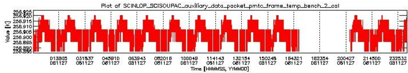
sciamachy_daily_report_level0_KSPT_L0_4303_N_20081127_1.PNG
