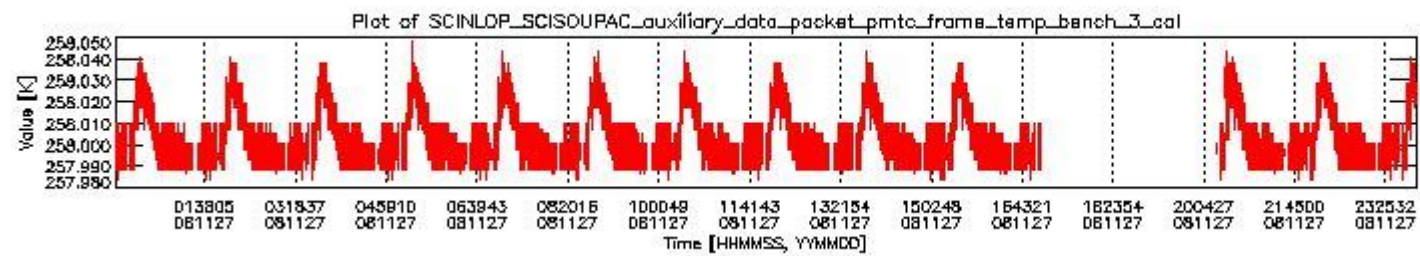
sciamachy_daily_report_level0_KSPT_L0_4303_N_20081127_2.PNG
