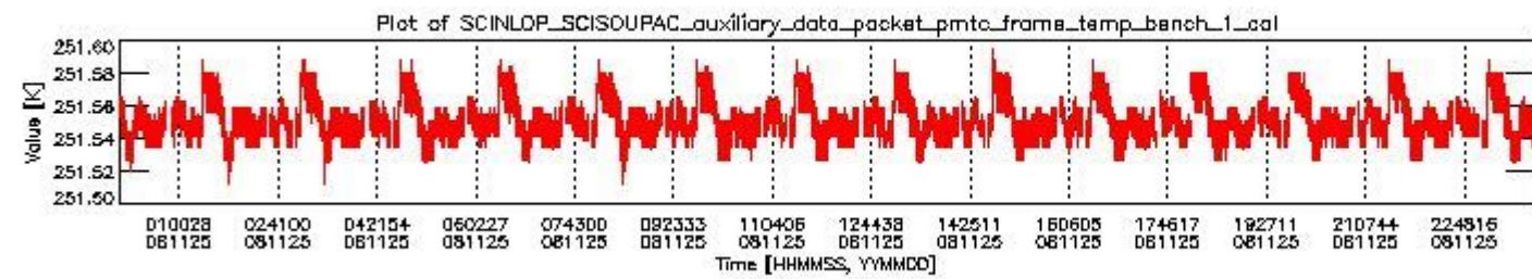
sciamachy_daily_report_level0_KSPT_L0_4303_N_20081125_0.PNG
