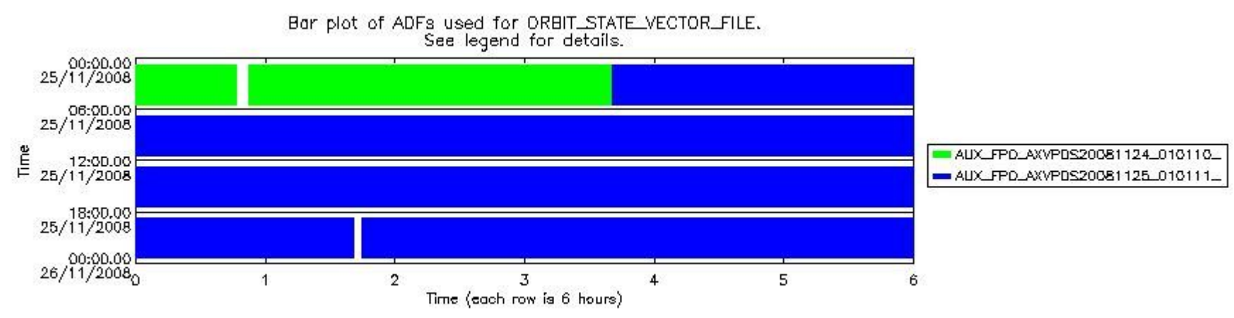
sciamachy_daily_report_level0_KSPT_L0_4303_N_20081125_8.PNG
