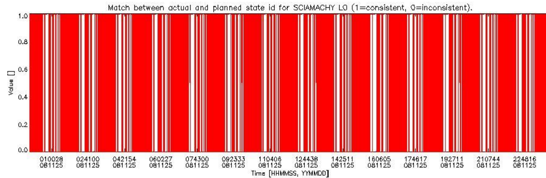
sciamachy_daily_report_level0_KSPT_L0_4303_N_20081125_5.PNG
