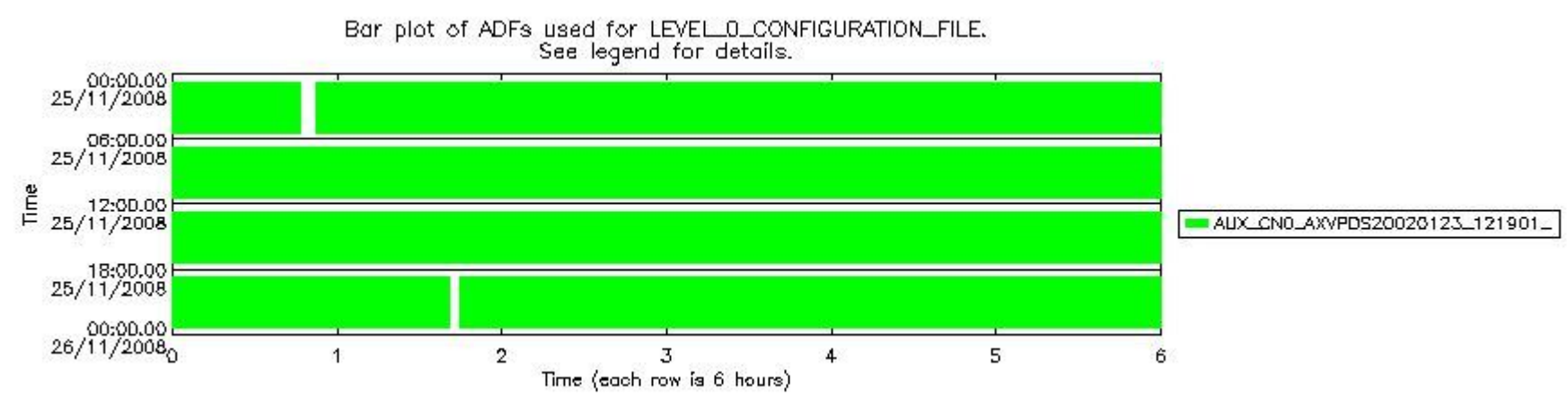
sciamachy_daily_report_level0_KSPT_L0_4303_N_20081125_7.PNG
