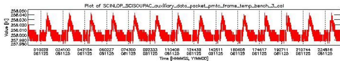
sciamachy_daily_report_level0_KSPT_L0_4303_N_20081125_2.PNG
