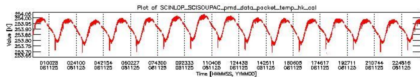
sciamachy_daily_report_level0_KSPT_L0_4303_N_20081125_3.PNG
