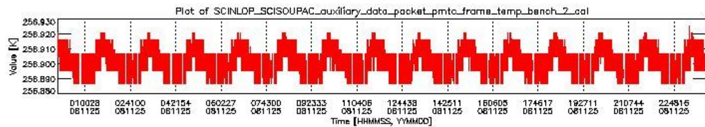
sciamachy_daily_report_level0_KSPT_L0_4303_N_20081125_1.PNG
