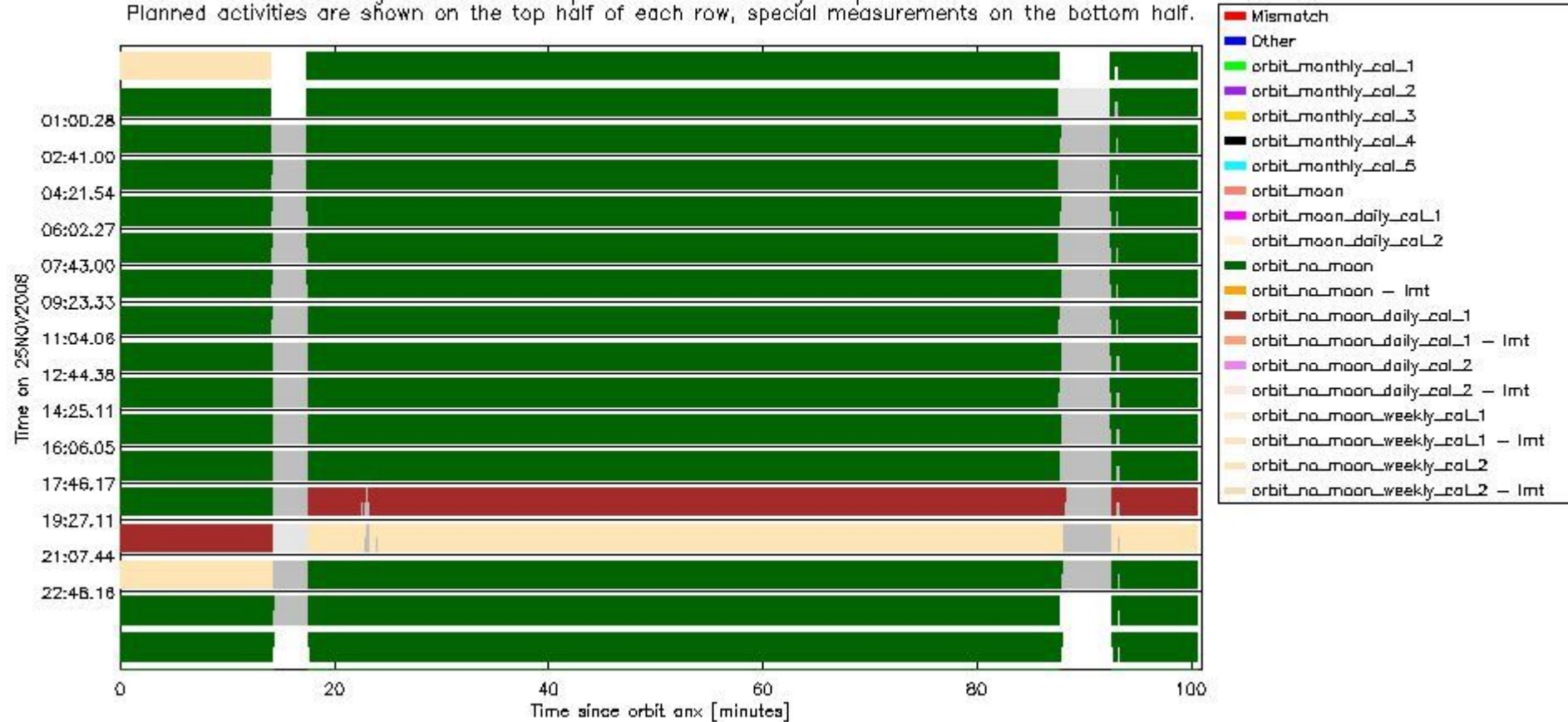
sciamachy_daily_report_level0_KSPT_L0_4303_N_20081125_6.PNG
