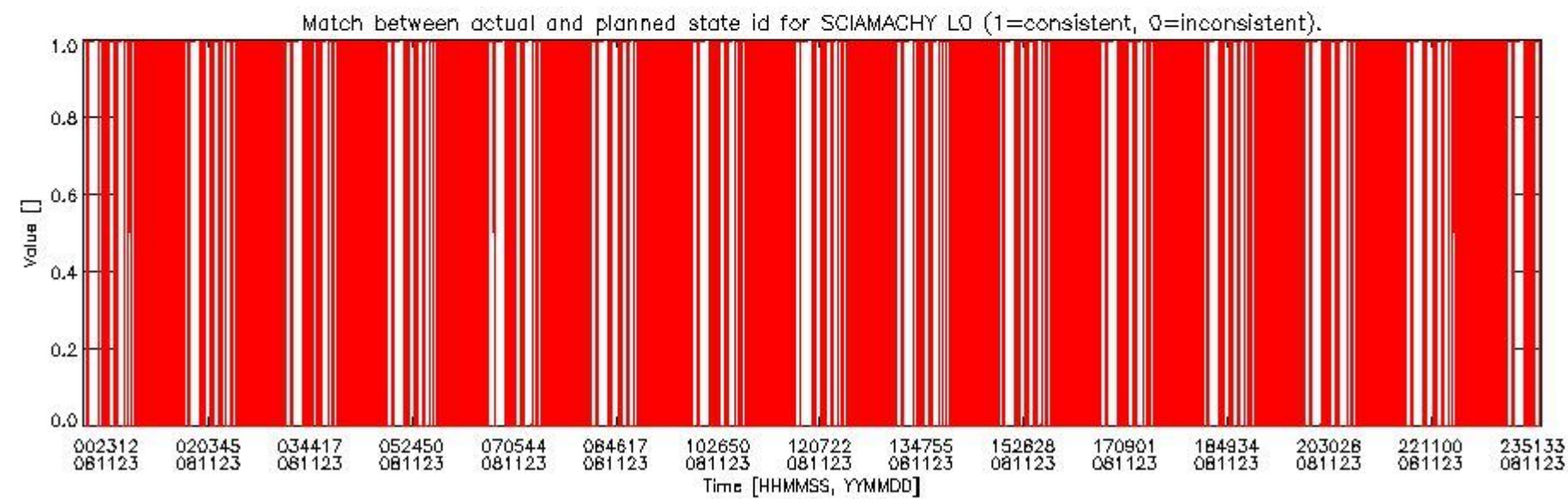
sciamachy_daily_report_level0_KSPT_L0_4303_N_20081123_5.PNG
