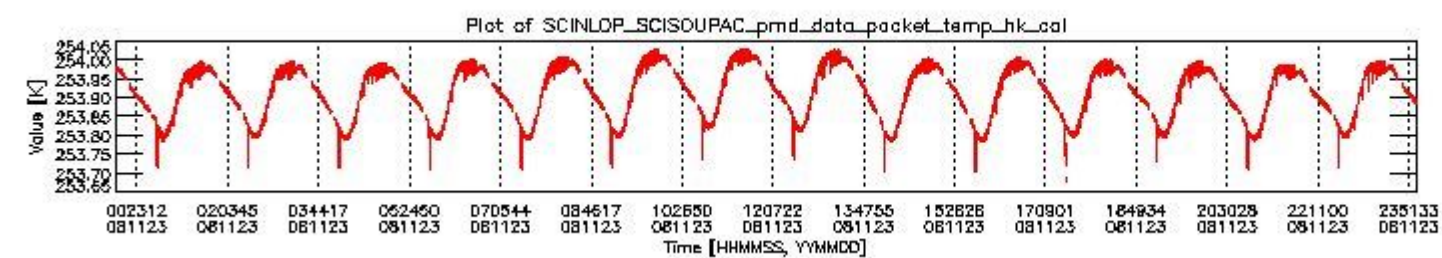
sciamachy_daily_report_level0_KSPT_L0_4303_N_20081123_3.PNG
