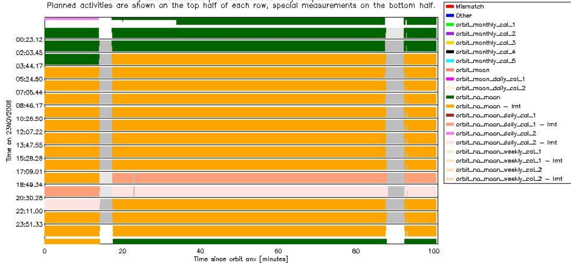
sciamachy_daily_report_level0_KSPT_L0_4303_N_20081123_6.PNG
