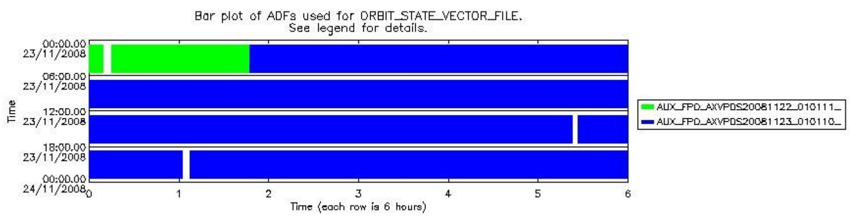
sciamachy_daily_report_level0_KSPT_L0_4303_N_20081123_8.PNG
