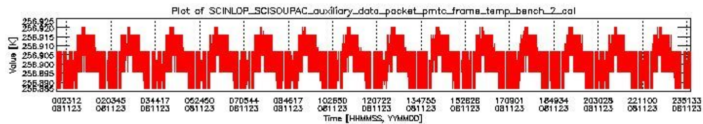
sciamachy_daily_report_level0_KSPT_L0_4303_N_20081123_1.PNG
