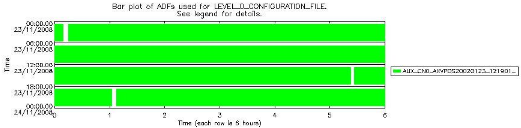
sciamachy_daily_report_level0_KSPT_L0_4303_N_20081123_7.PNG
