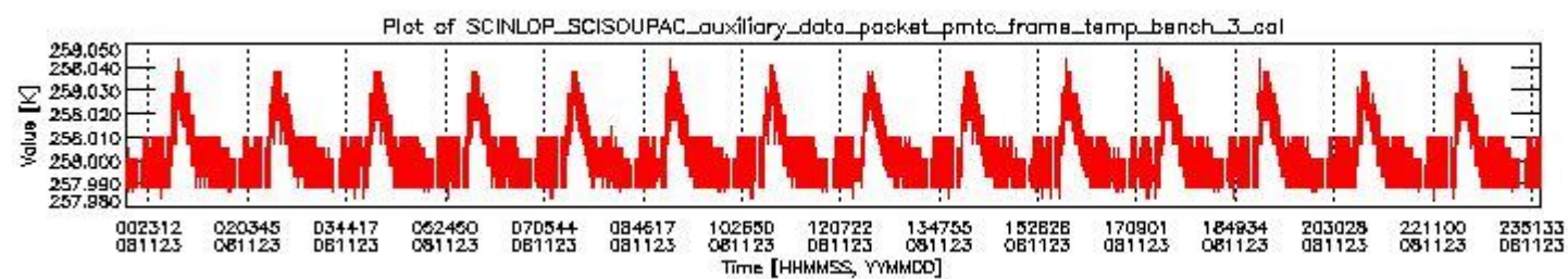
sciamachy_daily_report_level0_KSPT_L0_4303_N_20081123_2.PNG
