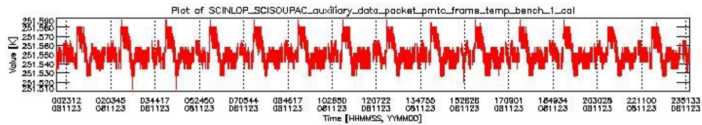
sciamachy_daily_report_level0_KSPT_L0_4303_N_20081123_0.PNG
