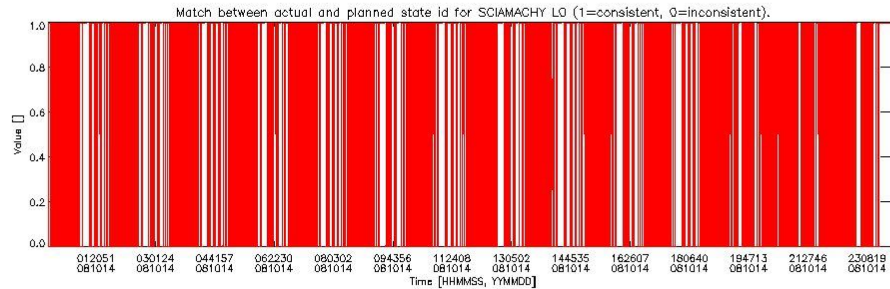
sciamachy_daily_report_level0_KSPT_L0_4303_N_20081014_5.PNG
