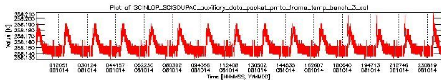
sciamachy_daily_report_level0_KSPT_L0_4303_N_20081014_2.PNG
