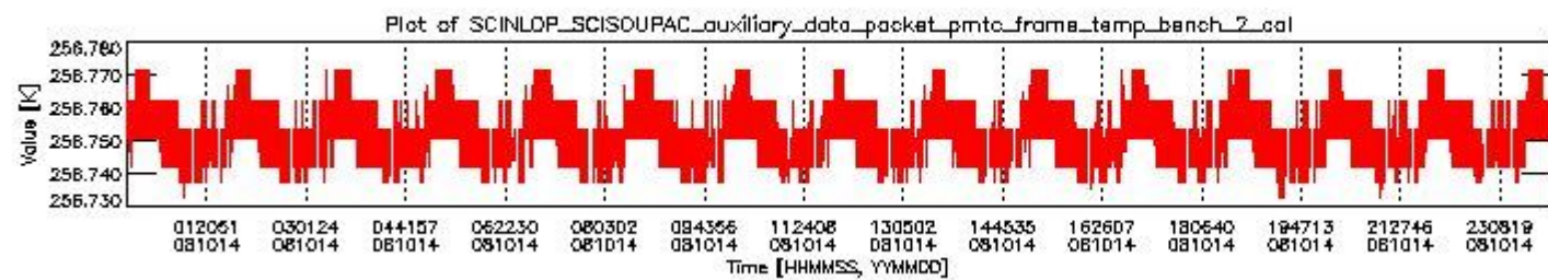
sciamachy_daily_report_level0_KSPT_L0_4303_N_20081014_1.PNG
