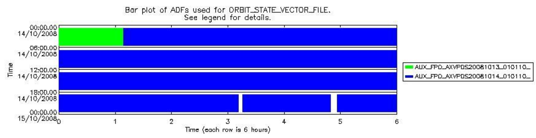
sciamachy_daily_report_level0_KSPT_L0_4303_N_20081014_8.PNG
