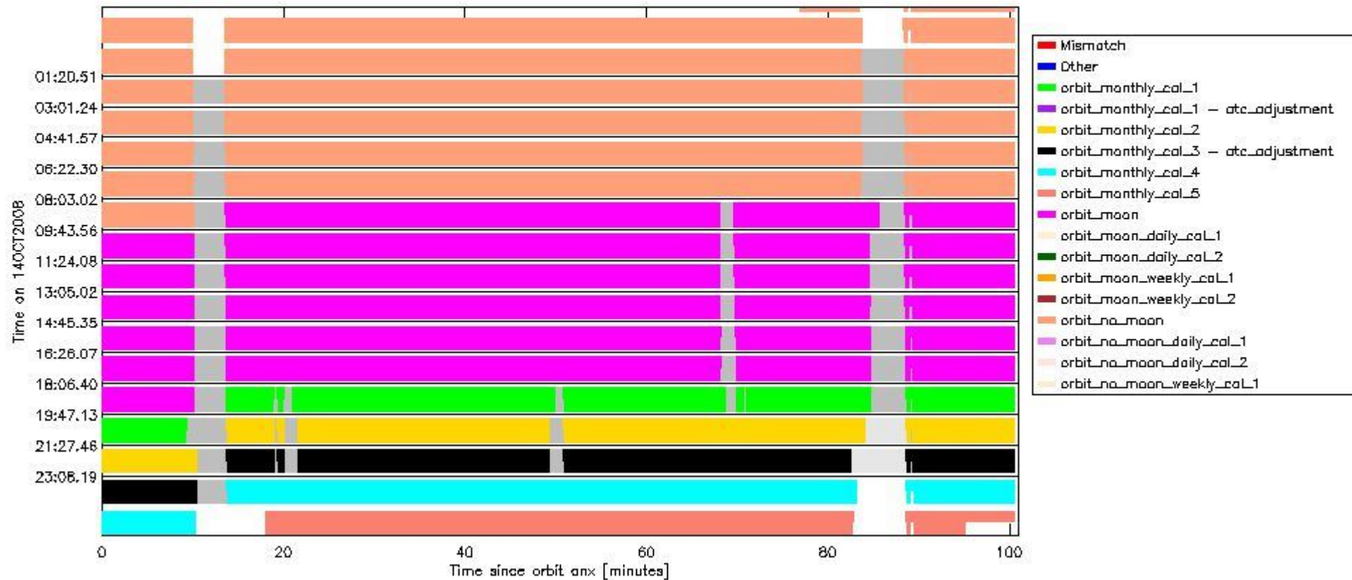
sciamachy_daily_report_level0_KSPT_L0_4303_N_20081014_6.PNG
