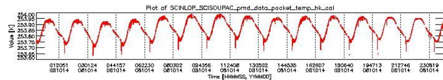
sciamachy_daily_report_level0_KSPT_L0_4303_N_20081014_3.PNG
