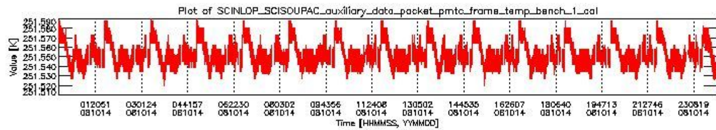
sciamachy_daily_report_level0_KSPT_L0_4303_N_20081014_0.PNG
