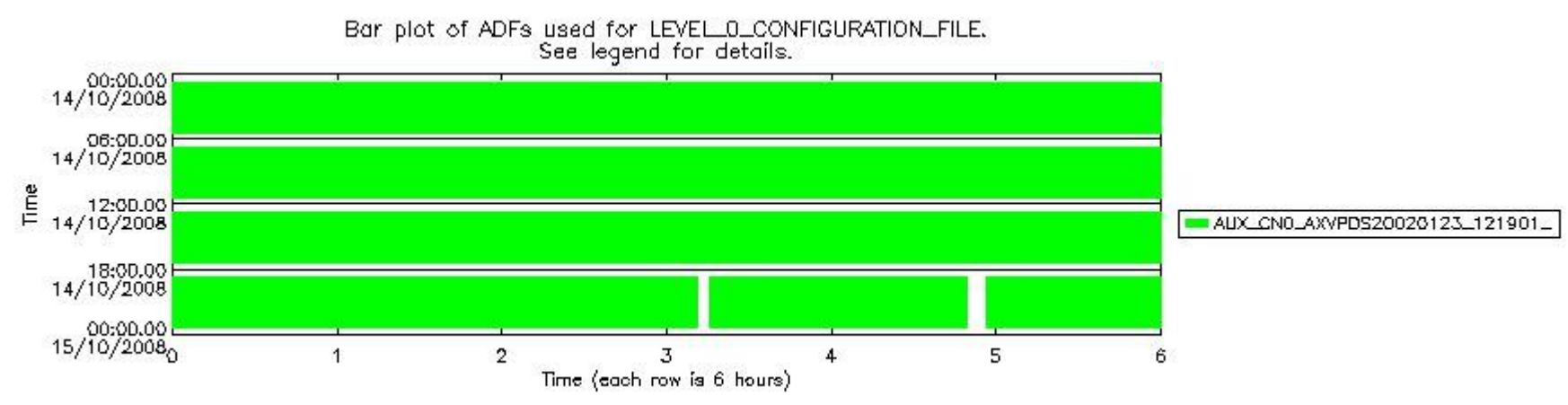
sciamachy_daily_report_level0_KSPT_L0_4303_N_20081014_7.PNG
