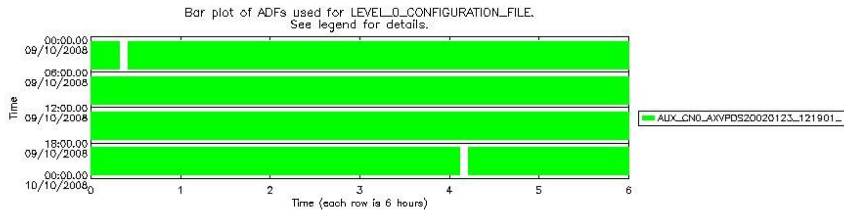
sciamachy_daily_report_level0_KSPT_L0_4303_N_20081009_7.PNG
