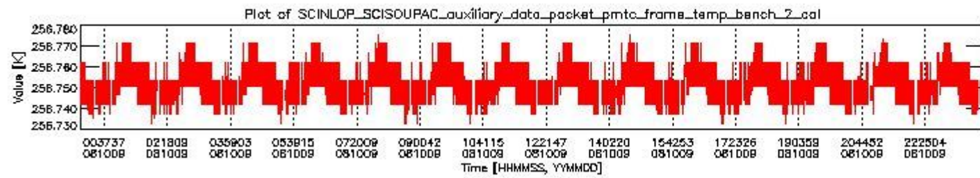
sciamachy_daily_report_level0_KSPT_L0_4303_N_20081009_1.PNG
