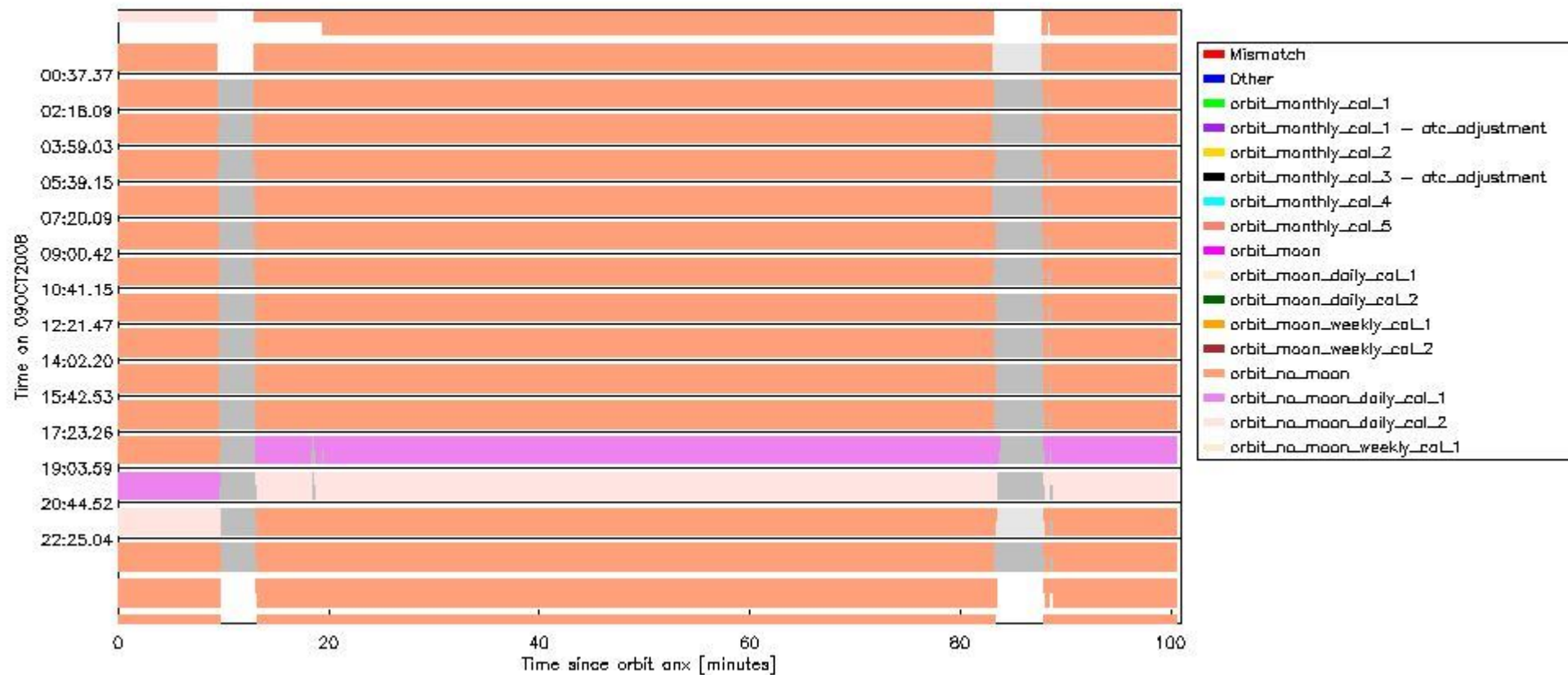
sciamachy_daily_report_level0_KSPT_L0_4303_N_20081009_6.PNG
