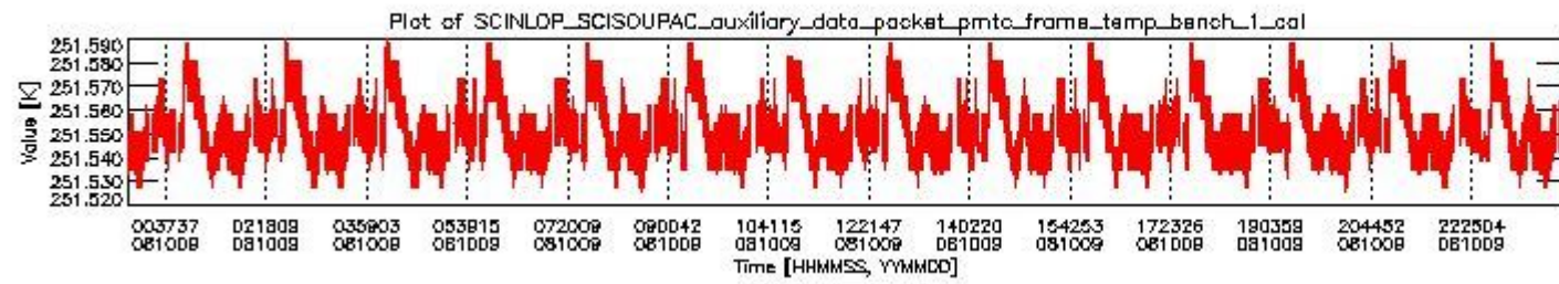
sciamachy_daily_report_level0_KSPT_L0_4303_N_20081009_0.PNG
