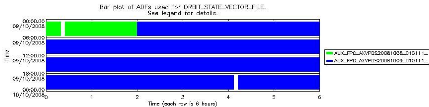
sciamachy_daily_report_level0_KSPT_L0_4303_N_20081009_8.PNG
