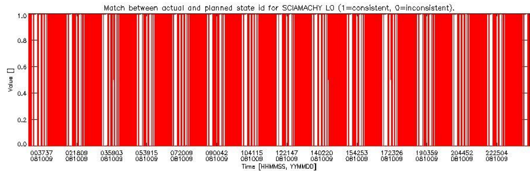
sciamachy_daily_report_level0_KSPT_L0_4303_N_20081009_5.PNG
