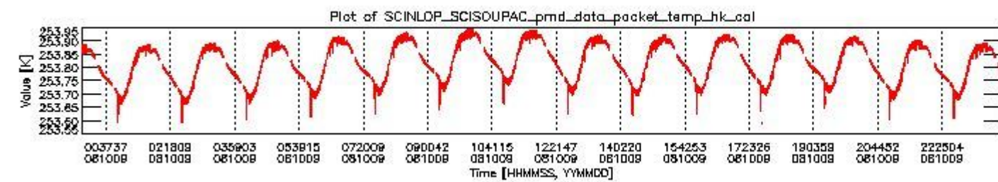
sciamachy_daily_report_level0_KSPT_L0_4303_N_20081009_3.PNG
