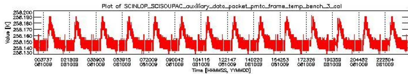
sciamachy_daily_report_level0_KSPT_L0_4303_N_20081009_2.PNG
