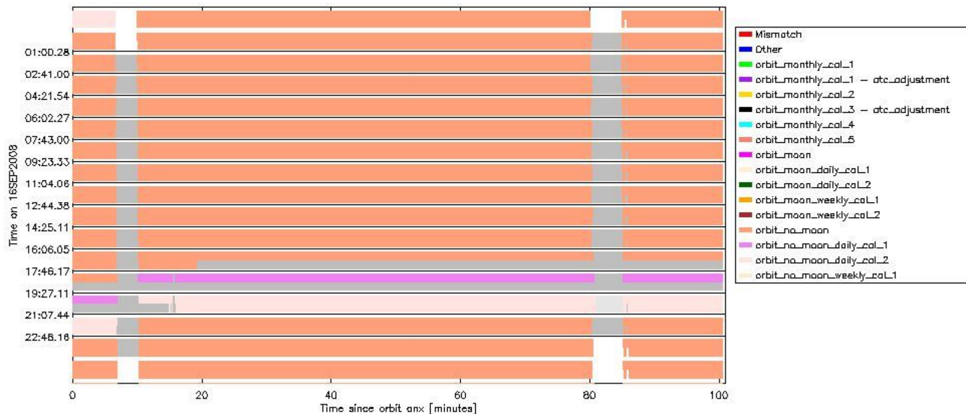
sciamachy_daily_report_level0_KSPT_L0_4303_N_20080916_6.PNG
