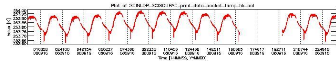
sciamachy_daily_report_level0_KSPT_L0_4303_N_20080916_3.PNG
