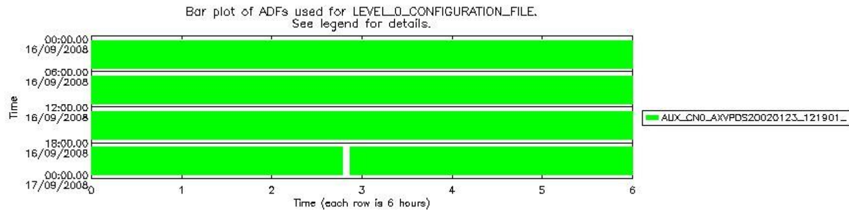
sciamachy_daily_report_level0_KSPT_L0_4303_N_20080916_7.PNG
