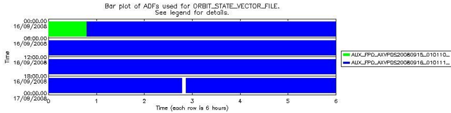
sciamachy_daily_report_level0_KSPT_L0_4303_N_20080916_8.PNG
