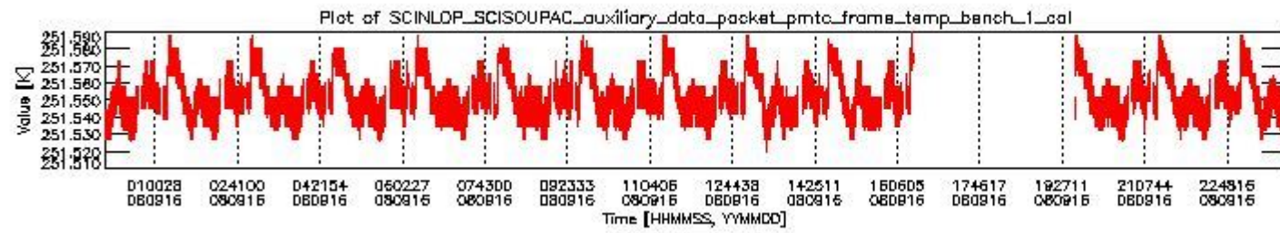
sciamachy_daily_report_level0_KSPT_L0_4303_N_20080916_0.PNG
