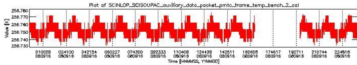
sciamachy_daily_report_level0_KSPT_L0_4303_N_20080916_1.PNG
