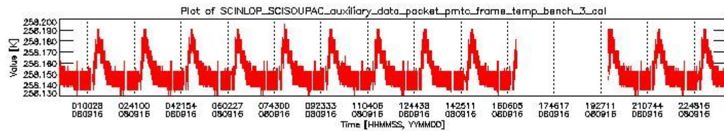
sciamachy_daily_report_level0_KSPT_L0_4303_N_20080916_2.PNG
