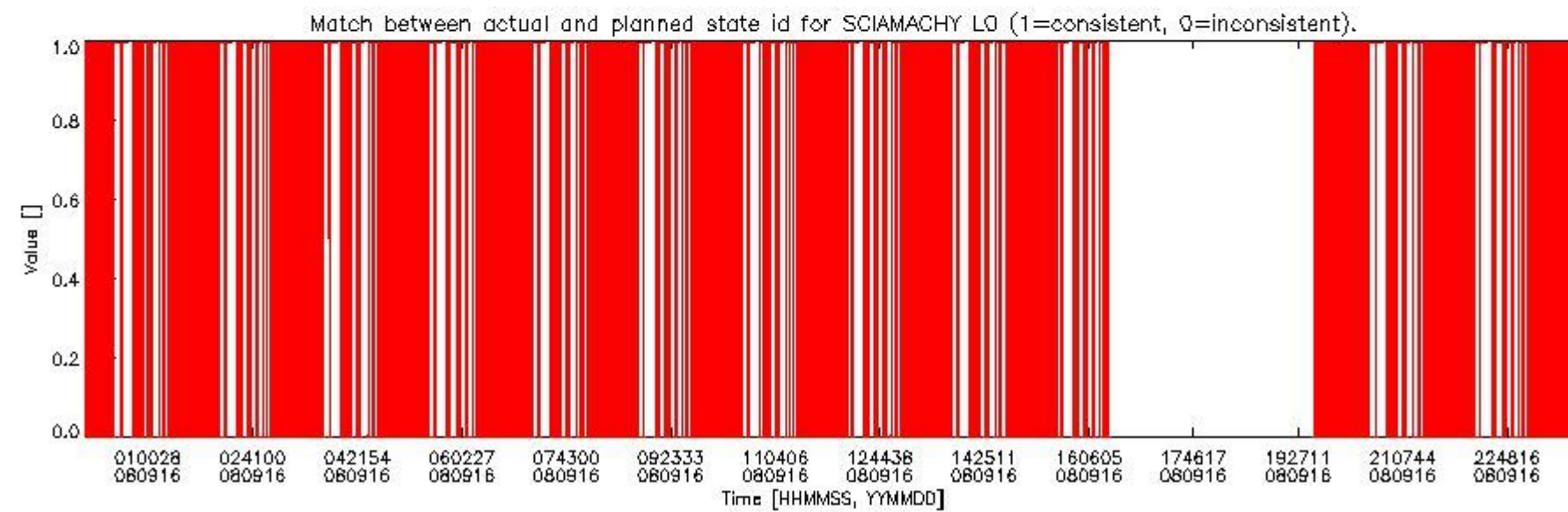
sciamachy_daily_report_level0_KSPT_L0_4303_N_20080916_5.PNG
