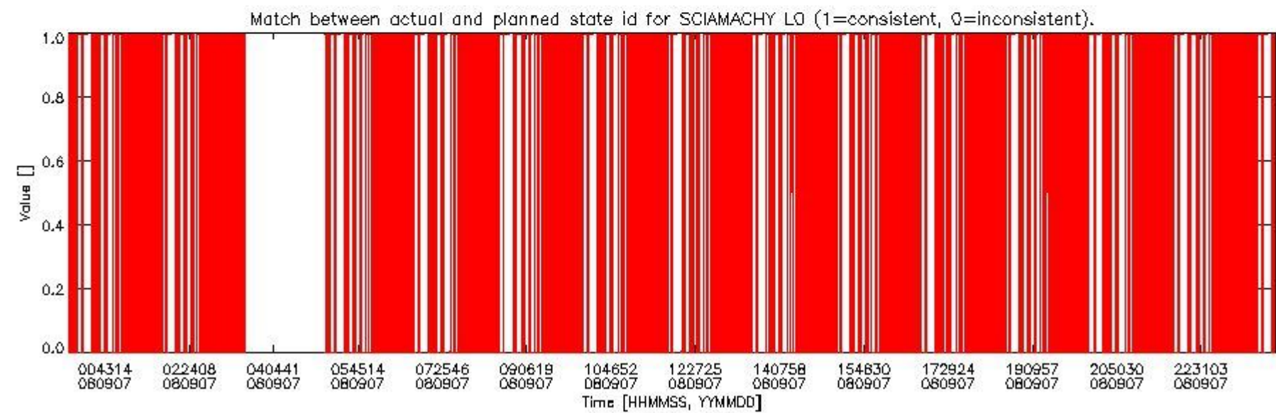
sciamachy_daily_report_level0_KSPT_L0_4303_N_20080907_5.PNG
