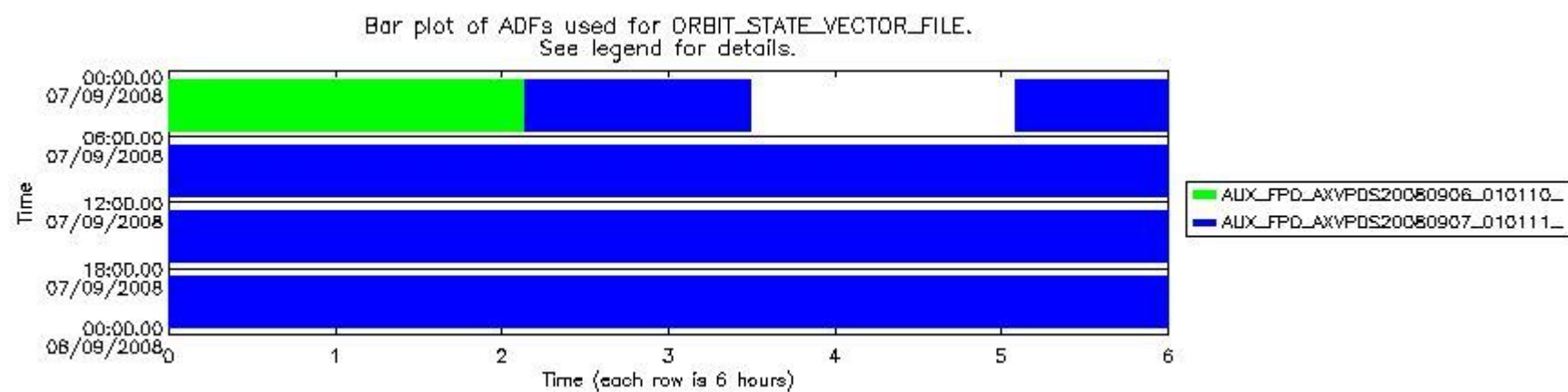
sciamachy_daily_report_level0_KSPT_L0_4303_N_20080907_8.PNG
