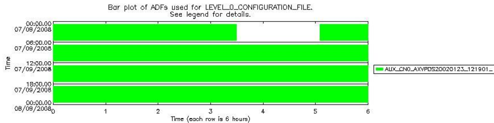
sciamachy_daily_report_level0_KSPT_L0_4303_N_20080907_7.PNG
