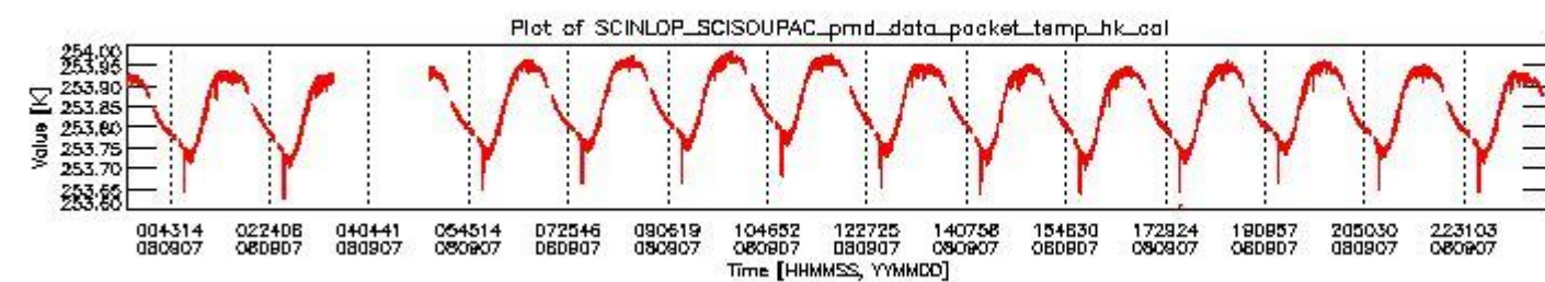
sciamachy_daily_report_level0_KSPT_L0_4303_N_20080907_3.PNG
