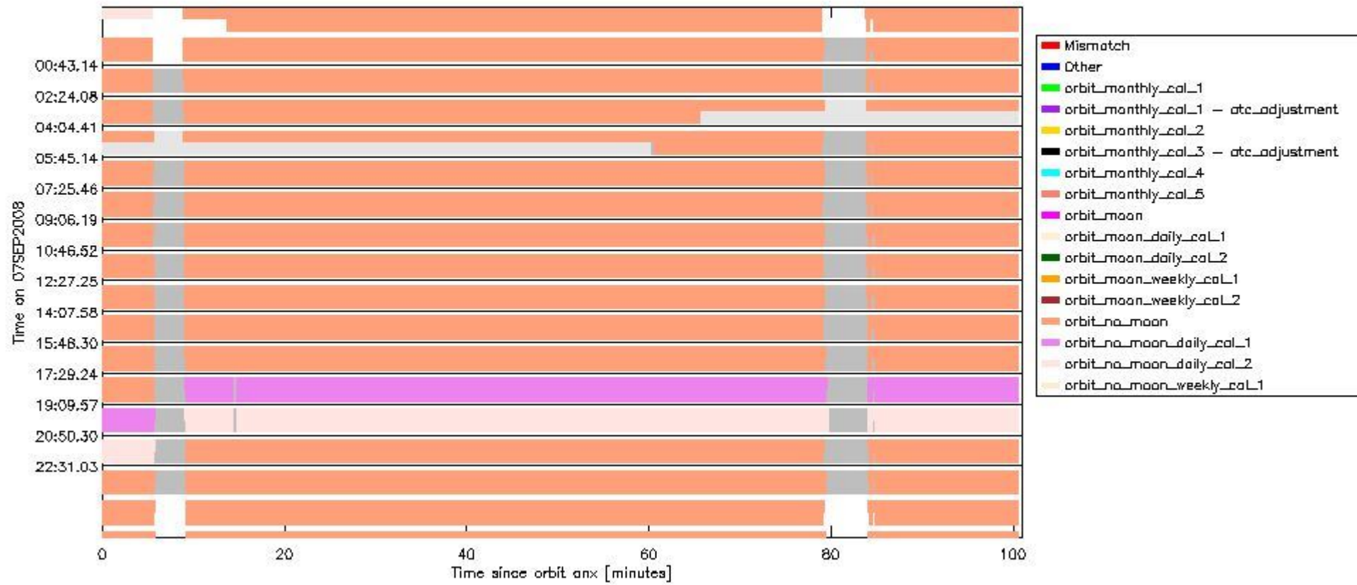
sciamachy_daily_report_level0_KSPT_L0_4303_N_20080907_6.PNG
