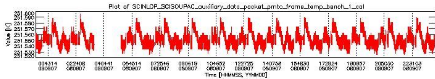
sciamachy_daily_report_level0_KSPT_L0_4303_N_20080907_0.PNG
