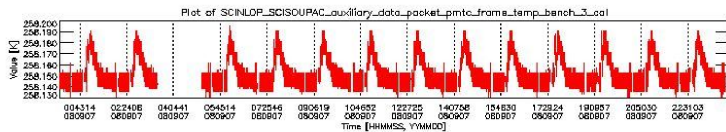
sciamachy_daily_report_level0_KSPT_L0_4303_N_20080907_2.PNG
