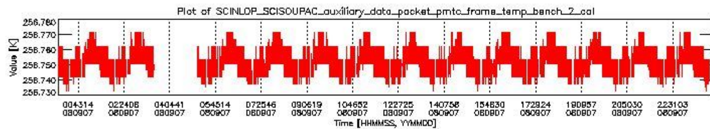
sciamachy_daily_report_level0_KSPT_L0_4303_N_20080907_1.PNG
