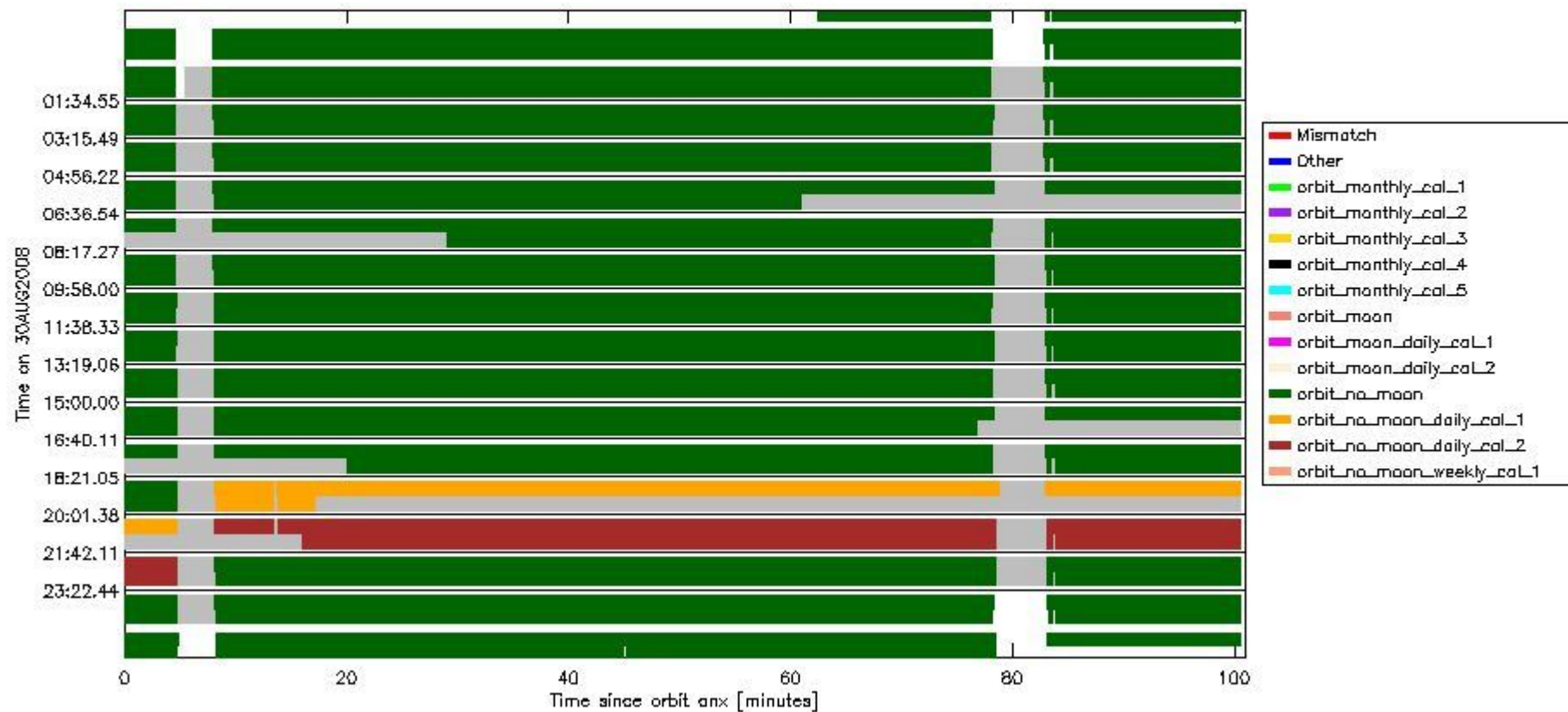
sciamachy_daily_report_level0_KSPT_L0_4303_N_20080830_6.PNG
