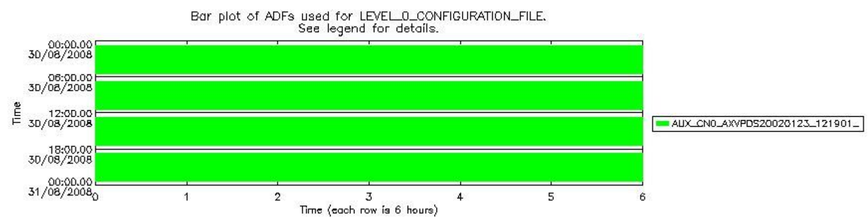
sciamachy_daily_report_level0_KSPT_L0_4303_N_20080830_7.PNG
