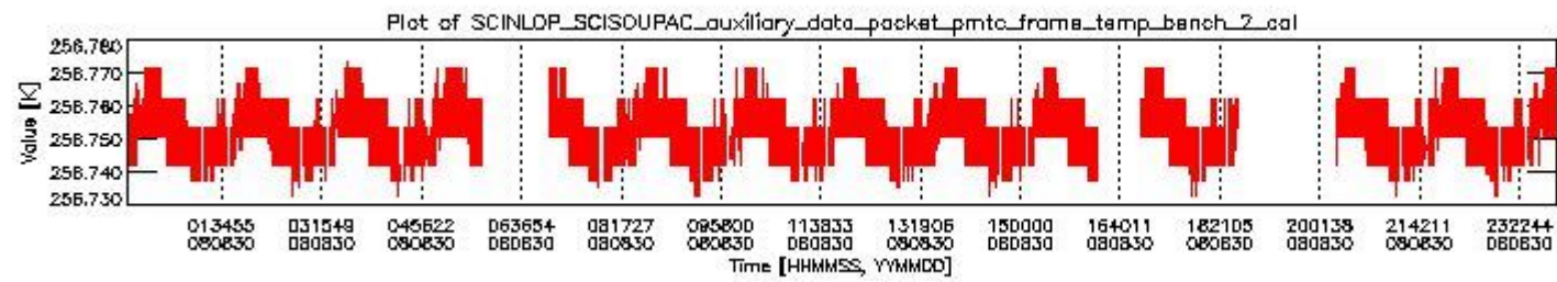
sciamachy_daily_report_level0_KSPT_L0_4303_N_20080830_1.PNG
