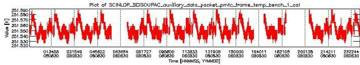
sciamachy_daily_report_level0_KSPT_L0_4303_N_20080830_0.PNG
