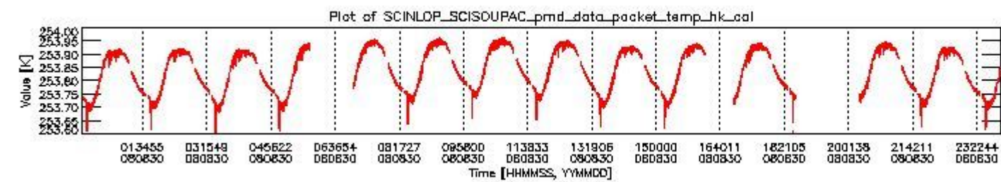
sciamachy_daily_report_level0_KSPT_L0_4303_N_20080830_3.PNG
