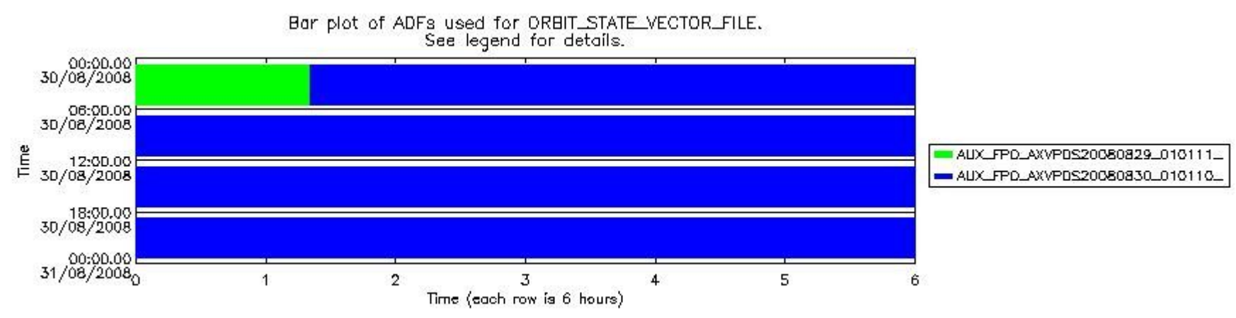
sciamachy_daily_report_level0_KSPT_L0_4303_N_20080830_8.PNG
