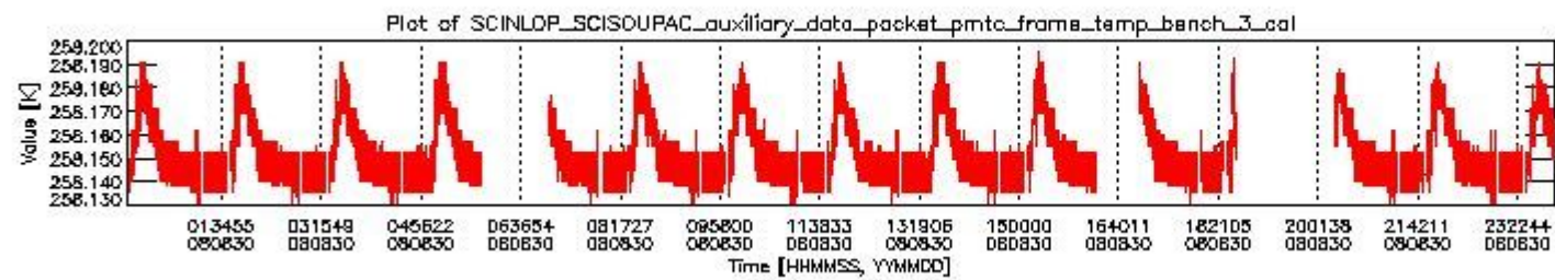
sciamachy_daily_report_level0_KSPT_L0_4303_N_20080830_2.PNG
