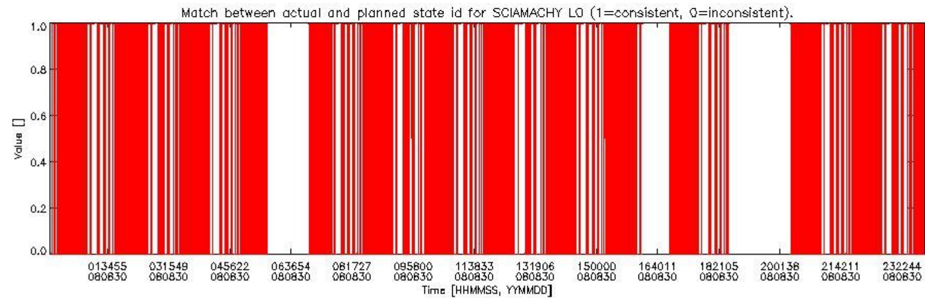
sciamachy_daily_report_level0_KSPT_L0_4303_N_20080830_5.PNG
