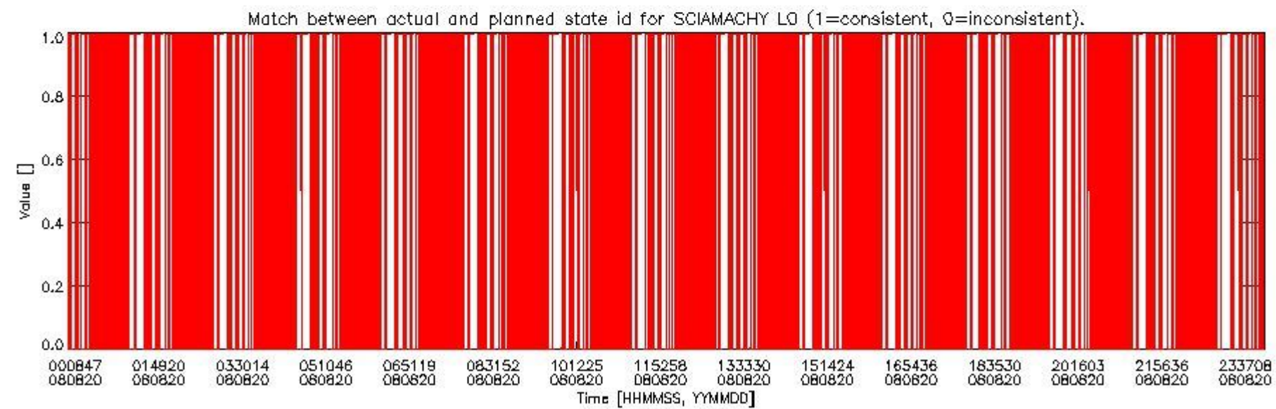
sciamachy_daily_report_level0_KSPT_L0_4303_N_20080820_5.PNG
