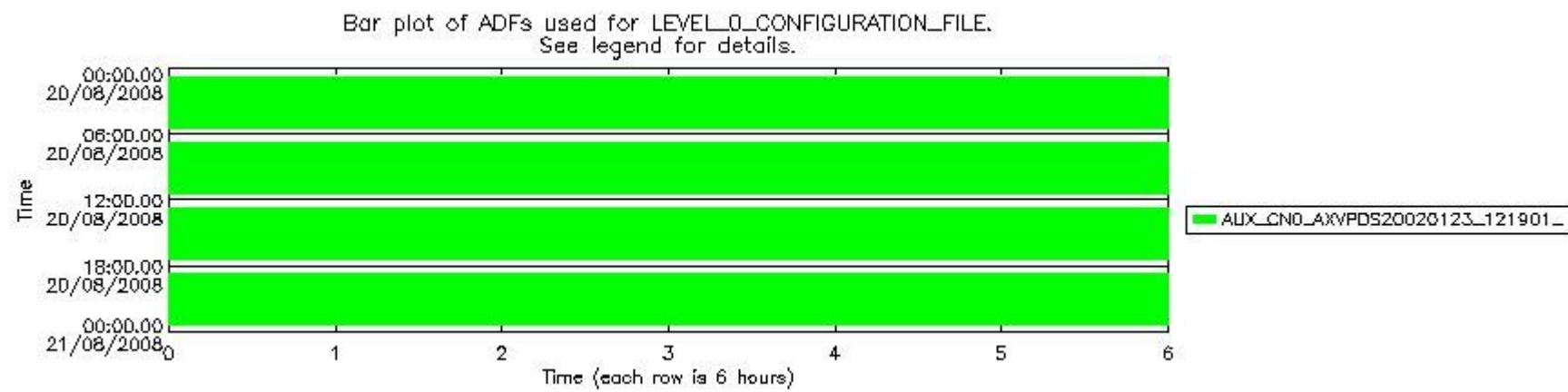
sciamachy_daily_report_level0_KSPT_L0_4303_N_20080820_7.PNG
