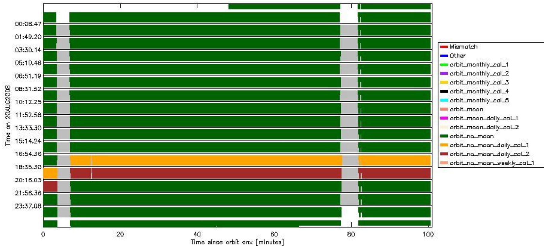
sciamachy_daily_report_level0_KSPT_L0_4303_N_20080820_6.PNG
