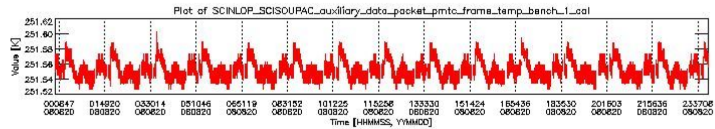
sciamachy_daily_report_level0_KSPT_L0_4303_N_20080820_0.PNG
