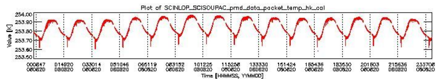
sciamachy_daily_report_level0_KSPT_L0_4303_N_20080820_3.PNG
