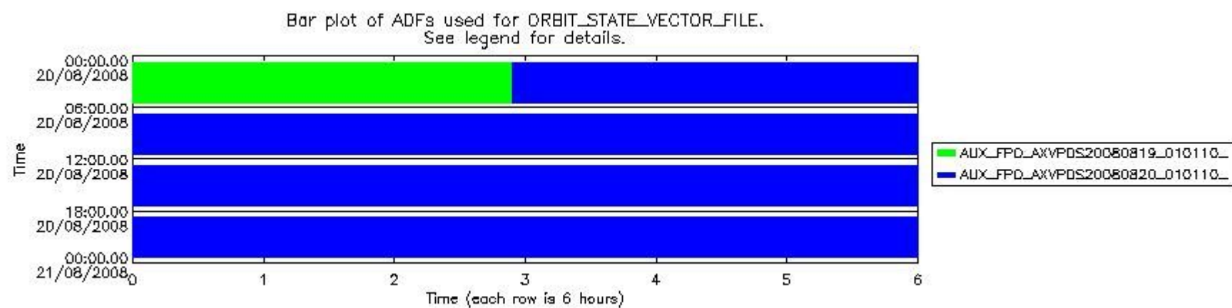
sciamachy_daily_report_level0_KSPT_L0_4303_N_20080820_8.PNG
