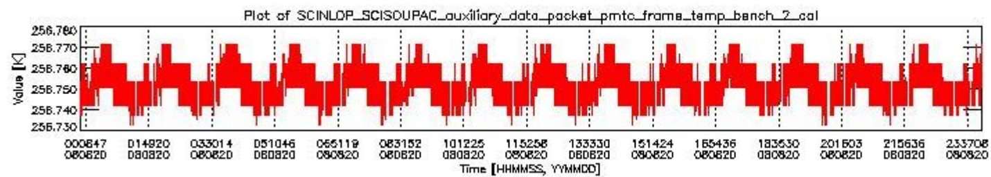
sciamachy_daily_report_level0_KSPT_L0_4303_N_20080820_1.PNG
