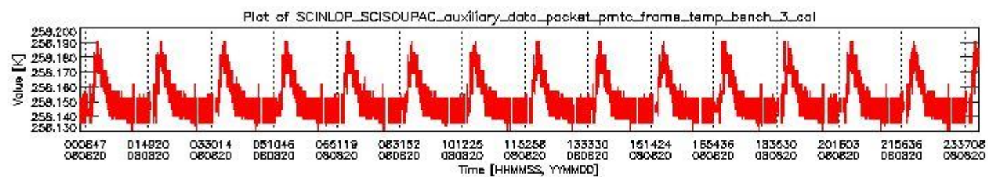
sciamachy_daily_report_level0_KSPT_L0_4303_N_20080820_2.PNG
