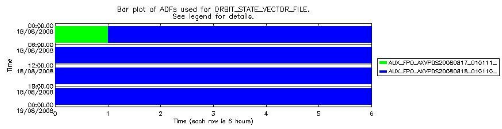
sciamachy_daily_report_level0_KSPT_L0_4303_N_20080818_8.PNG
