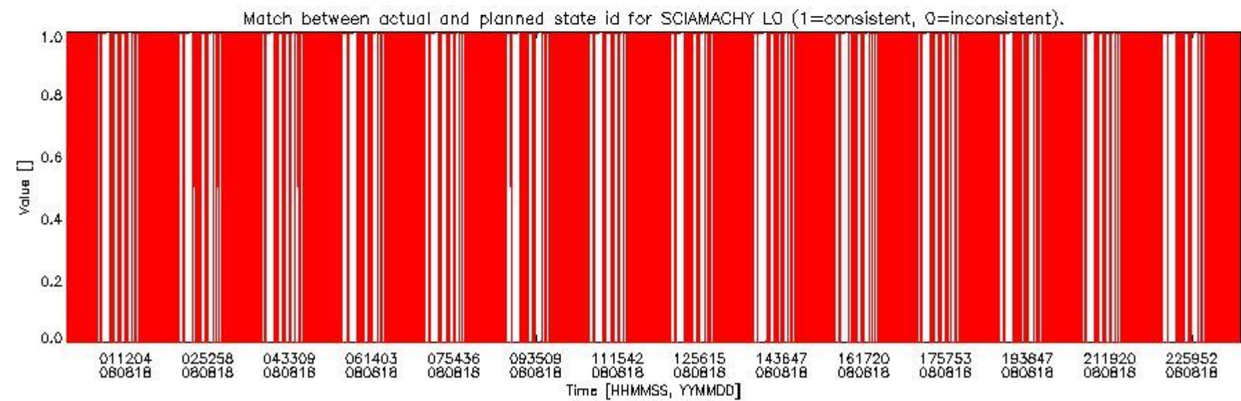
sciamachy_daily_report_level0_KSPT_L0_4303_N_20080818_5.PNG
