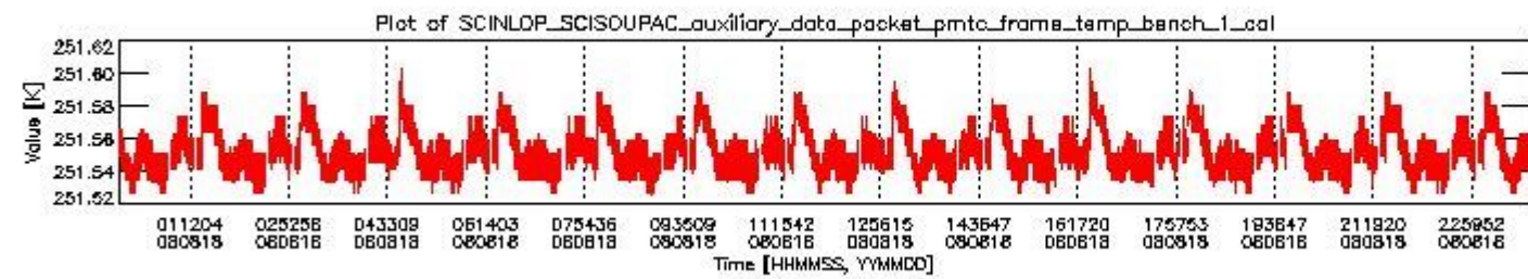
sciamachy_daily_report_level0_KSPT_L0_4303_N_20080818_0.PNG
