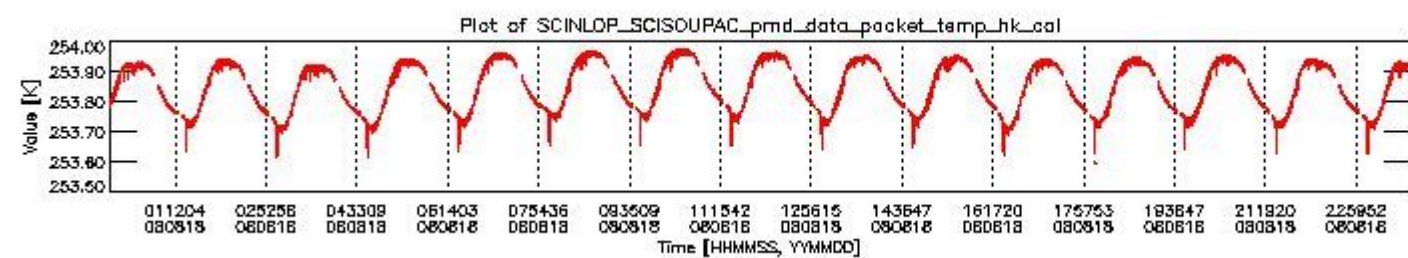
sciamachy_daily_report_level0_KSPT_L0_4303_N_20080818_3.PNG
