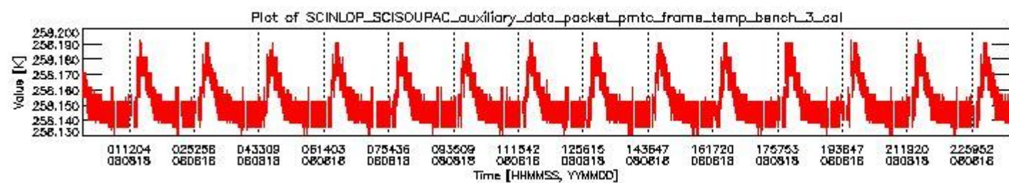
sciamachy_daily_report_level0_KSPT_L0_4303_N_20080818_2.PNG
