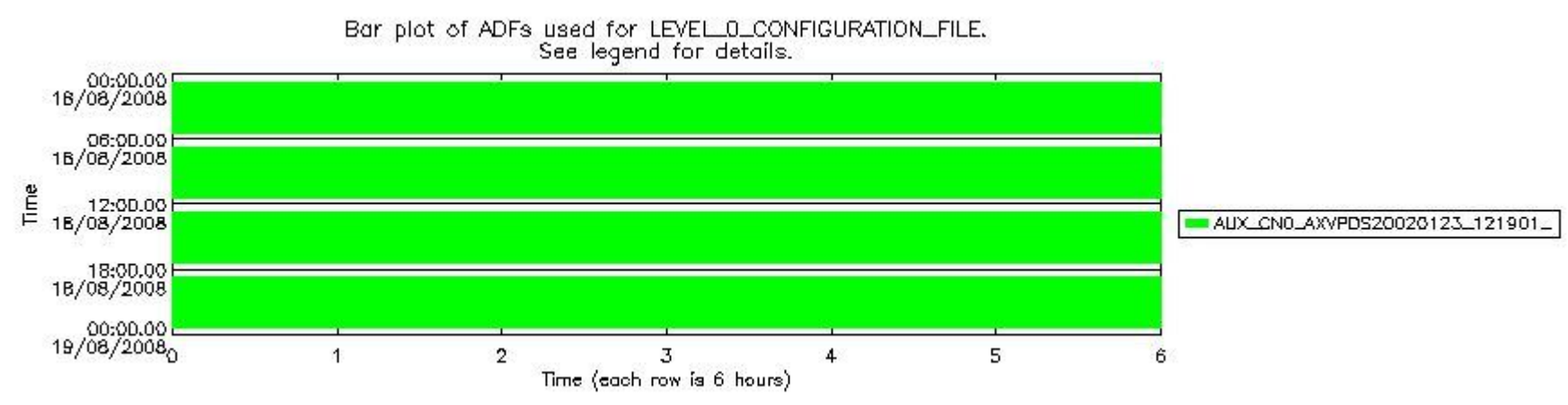
sciamachy_daily_report_level0_KSPT_L0_4303_N_20080818_7.PNG
