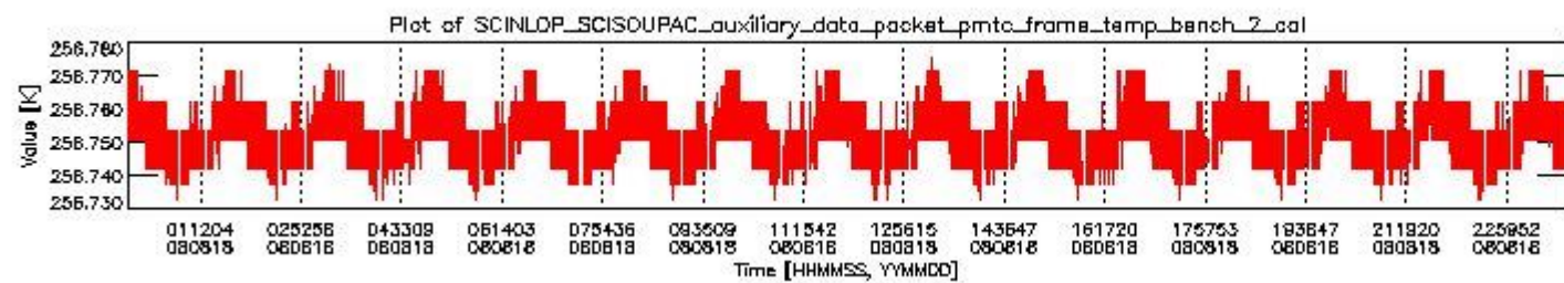
sciamachy_daily_report_level0_KSPT_L0_4303_N_20080818_1.PNG
