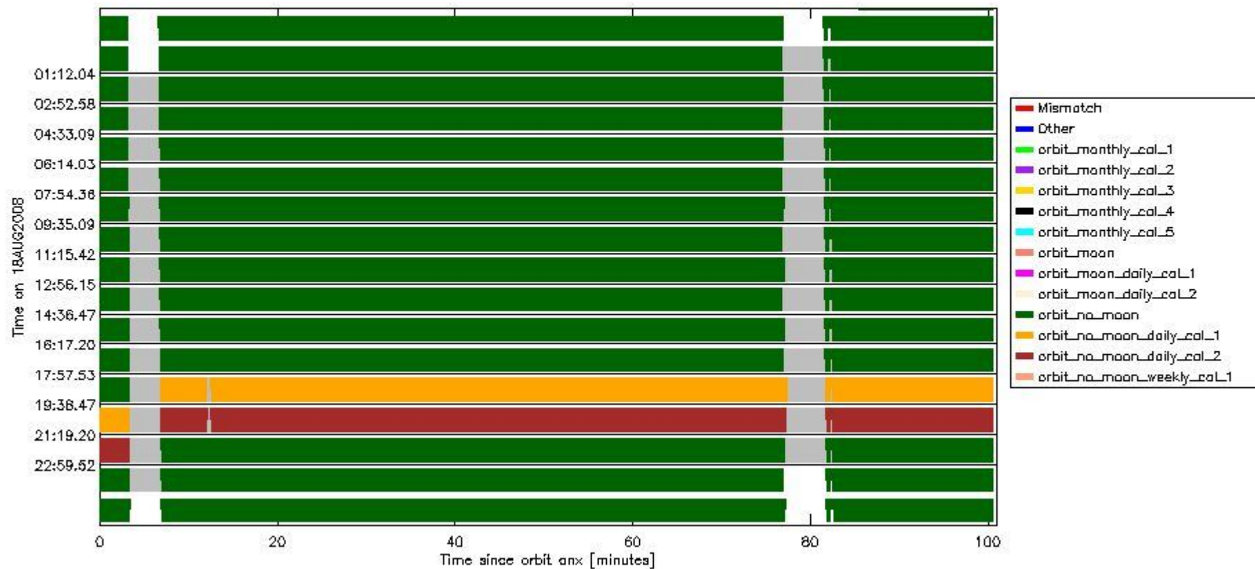
sciamachy_daily_report_level0_KSPT_L0_4303_N_20080818_6.PNG
