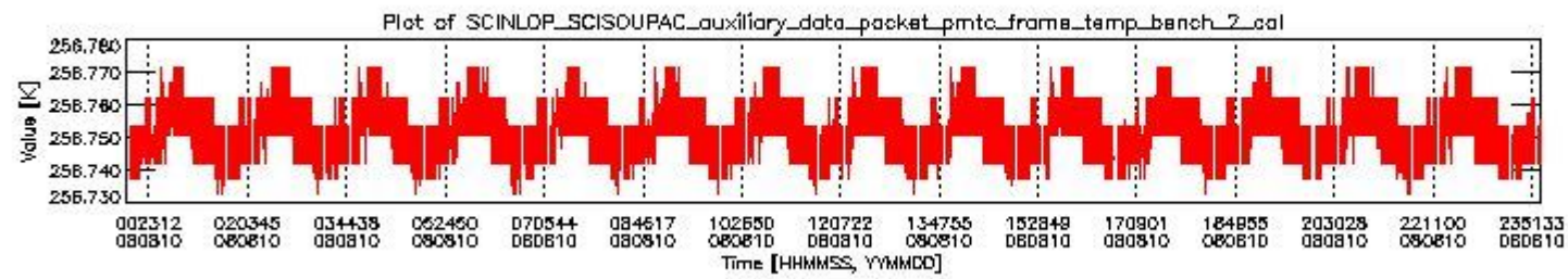
sciamachy_daily_report_level0_KSPT_L0_4303_N_20080810_1.PNG
