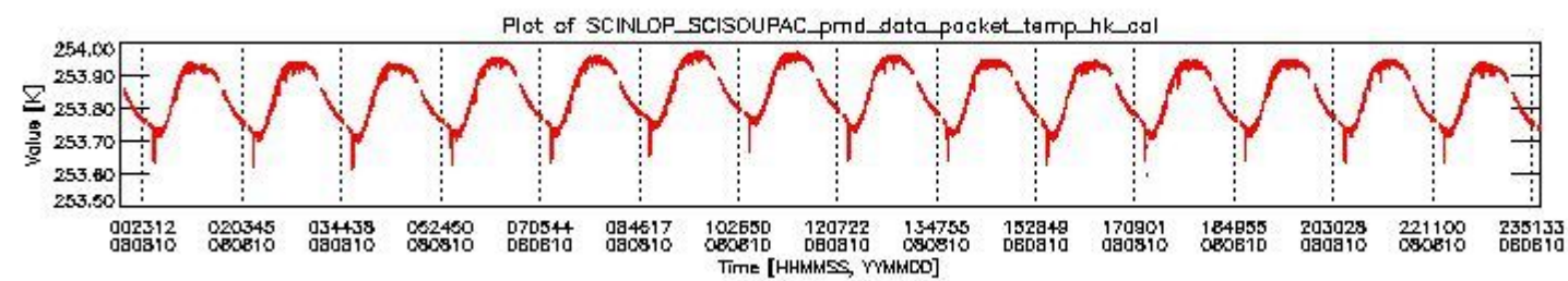
sciamachy_daily_report_level0_KSPT_L0_4303_N_20080810_3.PNG
