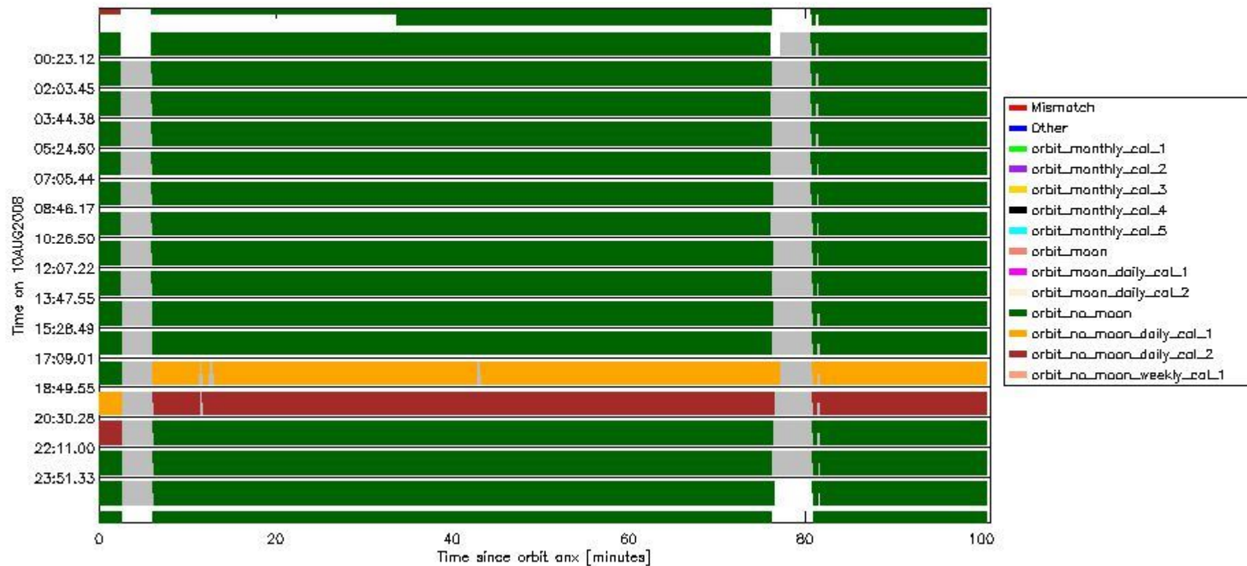
sciamachy_daily_report_level0_KSPT_L0_4303_N_20080810_6.PNG
