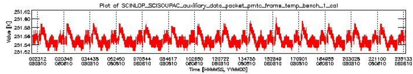
sciamachy_daily_report_level0_KSPT_L0_4303_N_20080810_0.PNG
