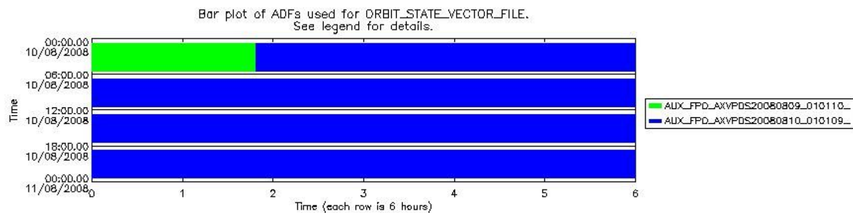
sciamachy_daily_report_level0_KSPT_L0_4303_N_20080810_8.PNG
