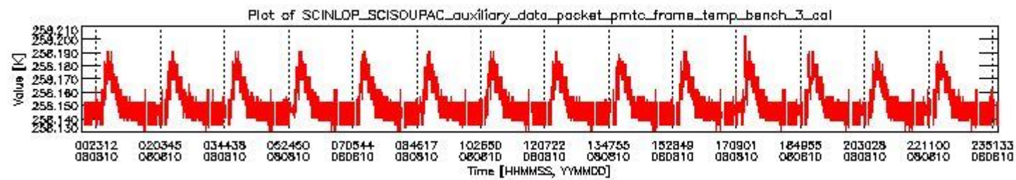
sciamachy_daily_report_level0_KSPT_L0_4303_N_20080810_2.PNG
