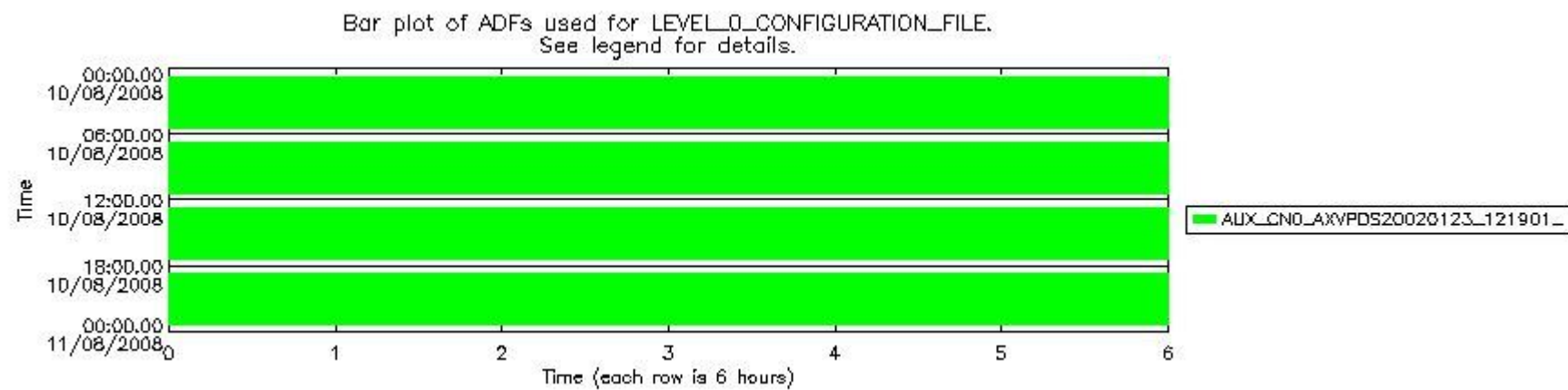
sciamachy_daily_report_level0_KSPT_L0_4303_N_20080810_7.PNG
