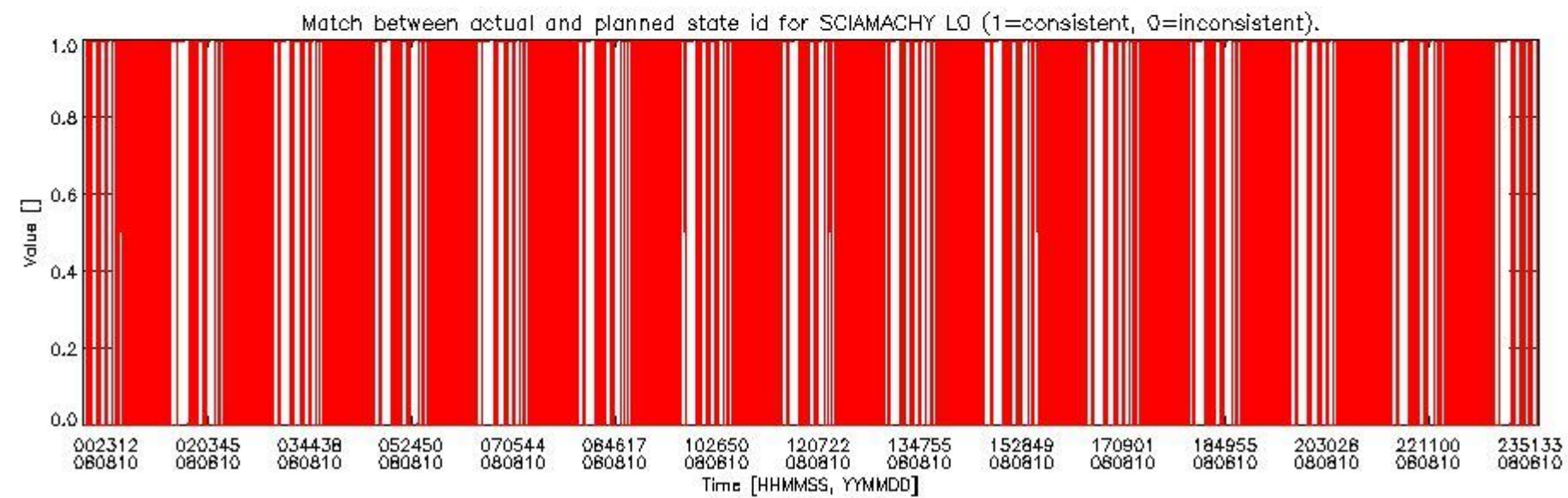
sciamachy_daily_report_level0_KSPT_L0_4303_N_20080810_5.PNG
