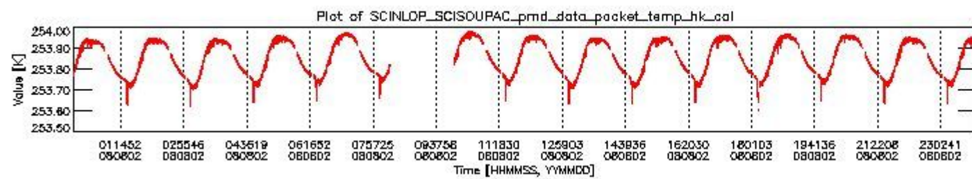
sciamachy_daily_report_level0_KSPT_L0_4303_N_20080802_3.PNG
