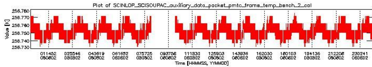
sciamachy_daily_report_level0_KSPT_L0_4303_N_20080802_1.PNG
