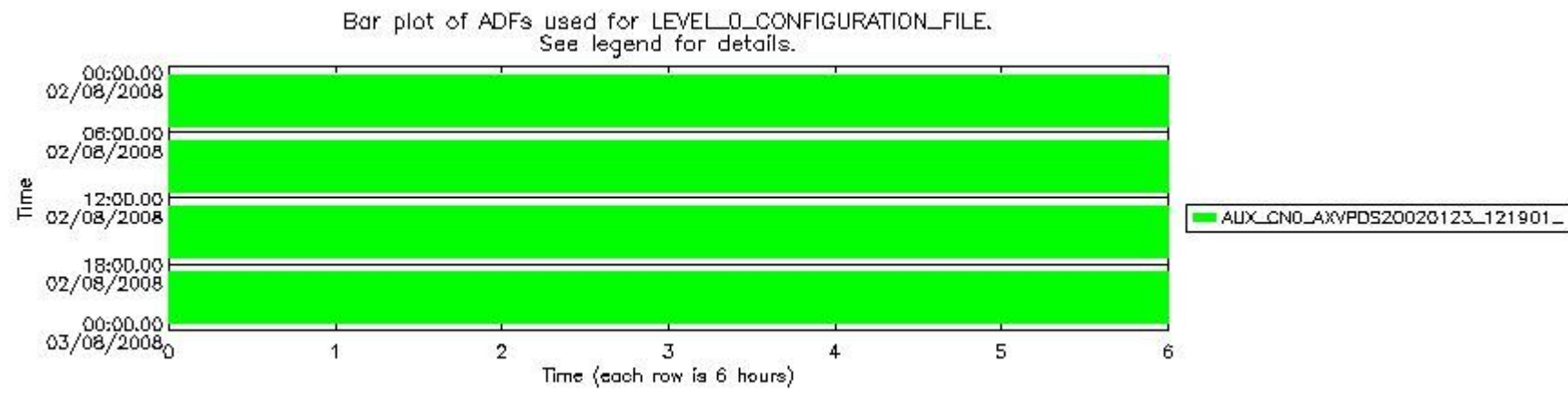
sciamachy_daily_report_level0_KSPT_L0_4303_N_20080802_7.PNG
