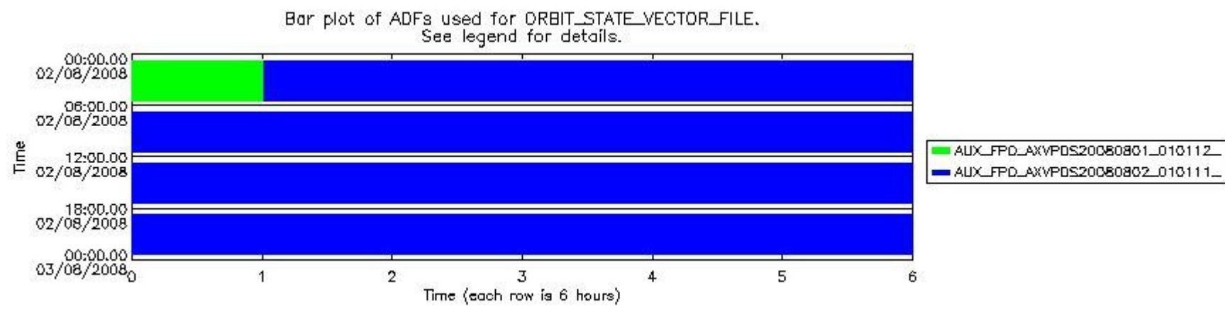
sciamachy_daily_report_level0_KSPT_L0_4303_N_20080802_8.PNG
