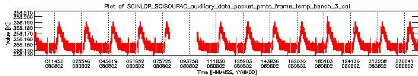
sciamachy_daily_report_level0_KSPT_L0_4303_N_20080802_2.PNG
