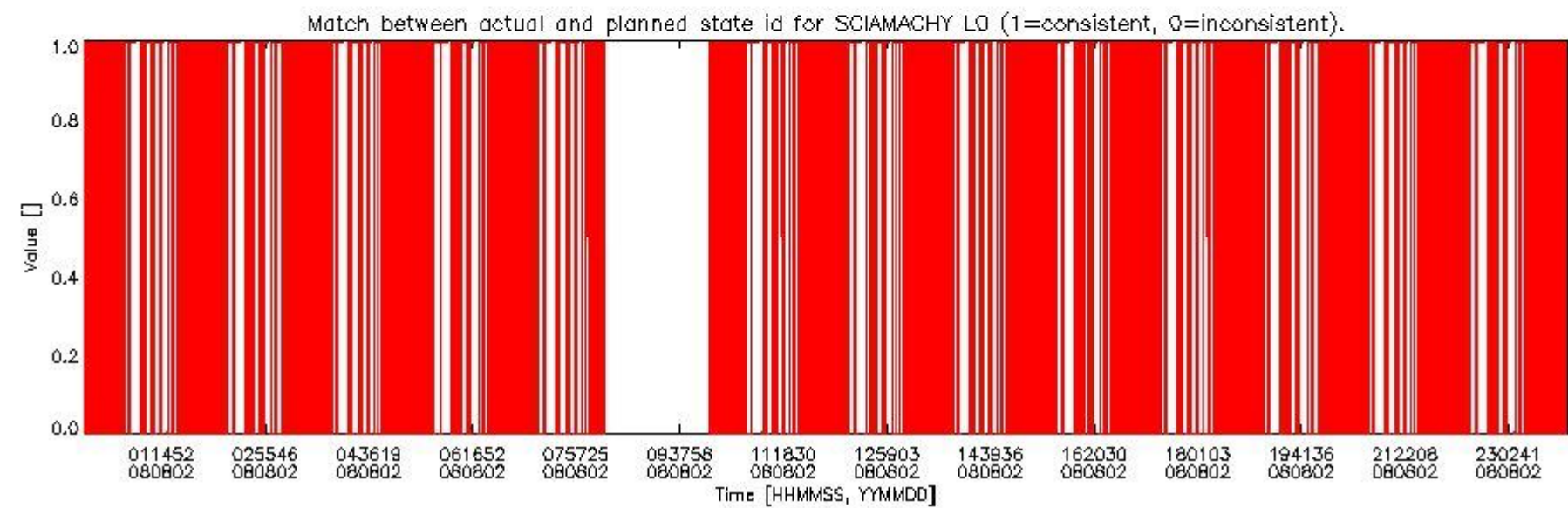
sciamachy_daily_report_level0_KSPT_L0_4303_N_20080802_5.PNG
