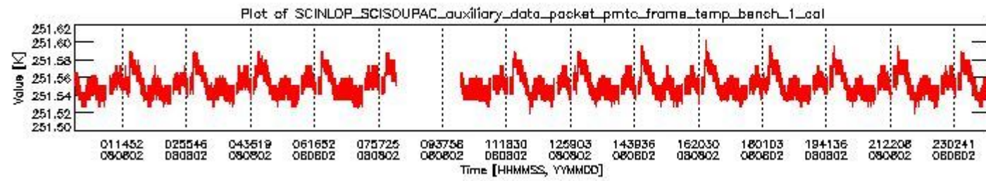
sciamachy_daily_report_level0_KSPT_L0_4303_N_20080802_0.PNG
