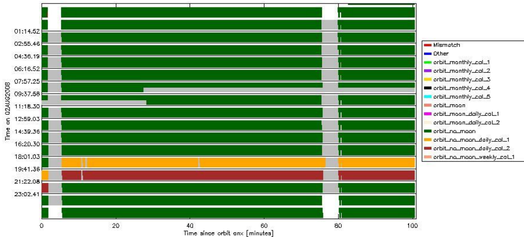
sciamachy_daily_report_level0_KSPT_L0_4303_N_20080802_6.PNG
