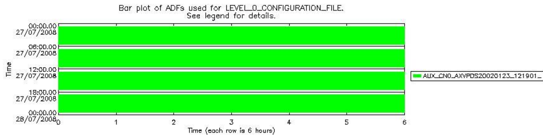
sciamachy_daily_report_level0_KSPT_L0_4303_N_20080727_6.PNG
