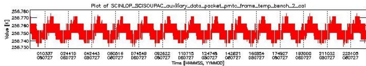
sciamachy_daily_report_level0_KSPT_L0_4303_N_20080727_1.PNG
