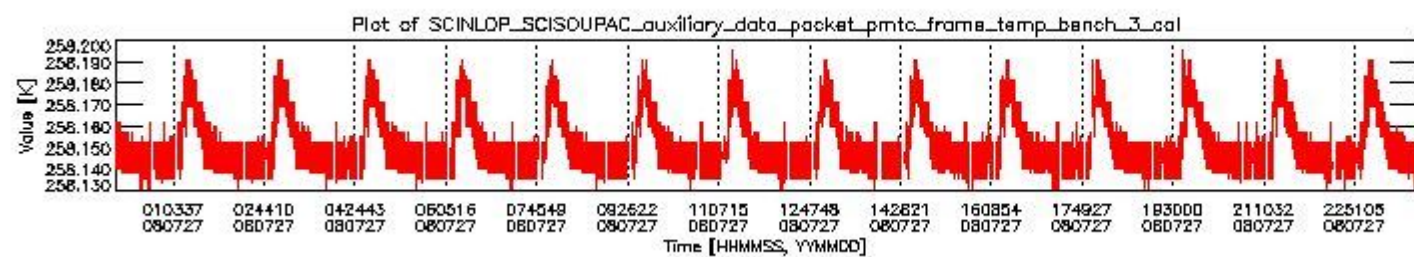
sciamachy_daily_report_level0_KSPT_L0_4303_N_20080727_2.PNG
