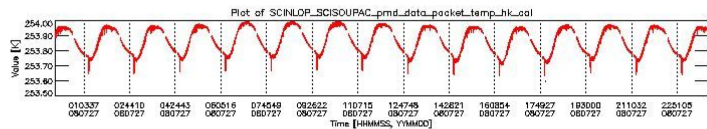
sciamachy_daily_report_level0_KSPT_L0_4303_N_20080727_3.PNG
