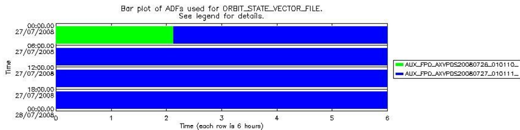
sciamachy_daily_report_level0_KSPT_L0_4303_N_20080727_7.PNG
