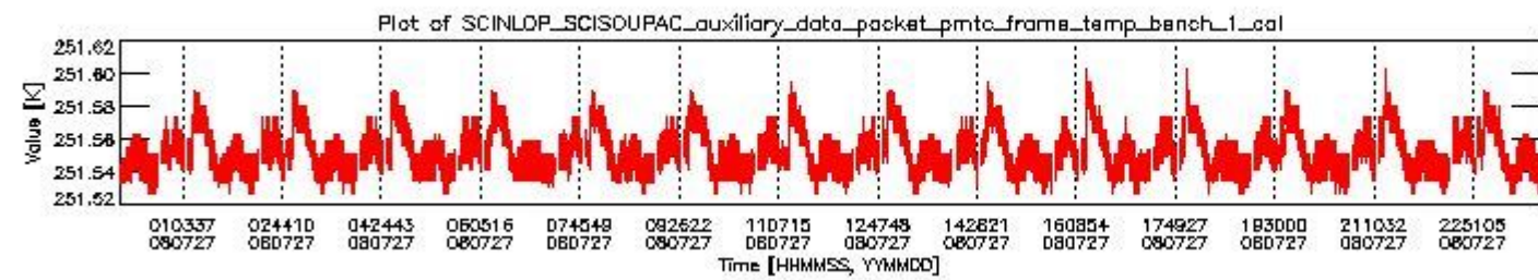
sciamachy_daily_report_level0_KSPT_L0_4303_N_20080727_0.PNG
