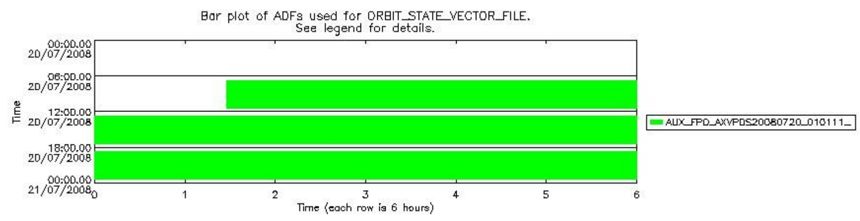
sciamachy_daily_report_level0_KSPT_L0_4303_N_20080720_8.PNG
