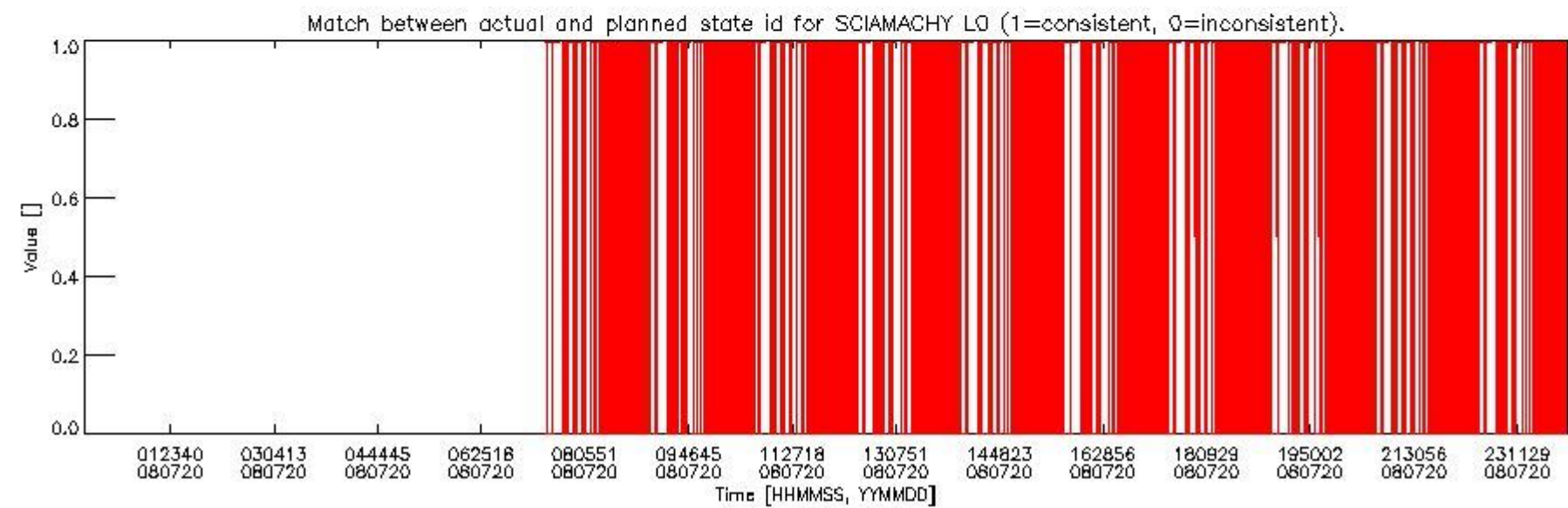
sciamachy_daily_report_level0_KSPT_L0_4303_N_20080720_5.PNG
