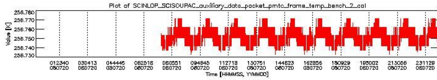
sciamachy_daily_report_level0_KSPT_L0_4303_N_20080720_1.PNG
