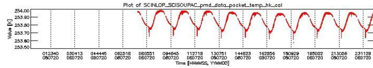
sciamachy_daily_report_level0_KSPT_L0_4303_N_20080720_3.PNG
