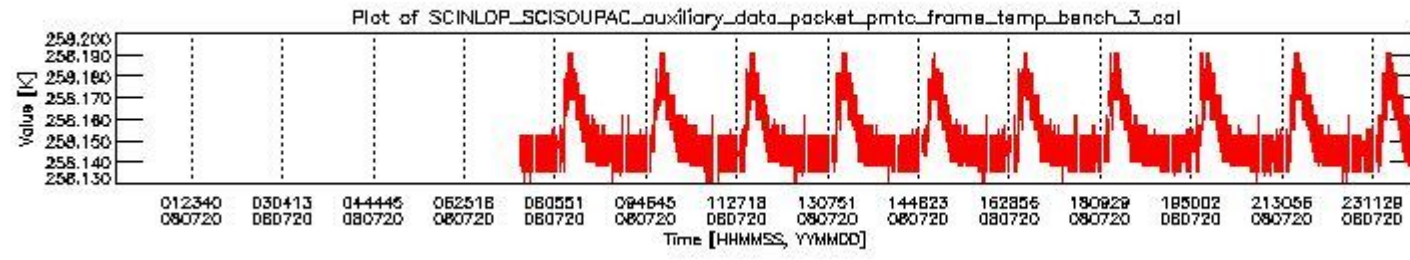
sciamachy_daily_report_level0_KSPT_L0_4303_N_20080720_2.PNG
