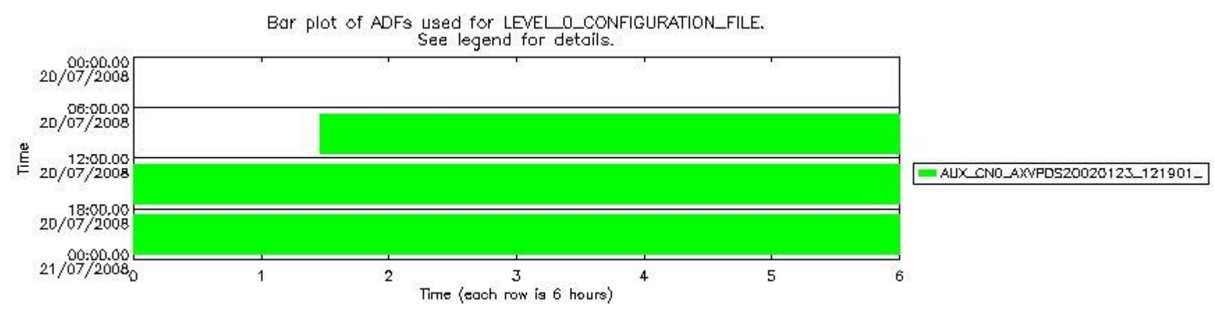
sciamachy_daily_report_level0_KSPT_L0_4303_N_20080720_7.PNG
