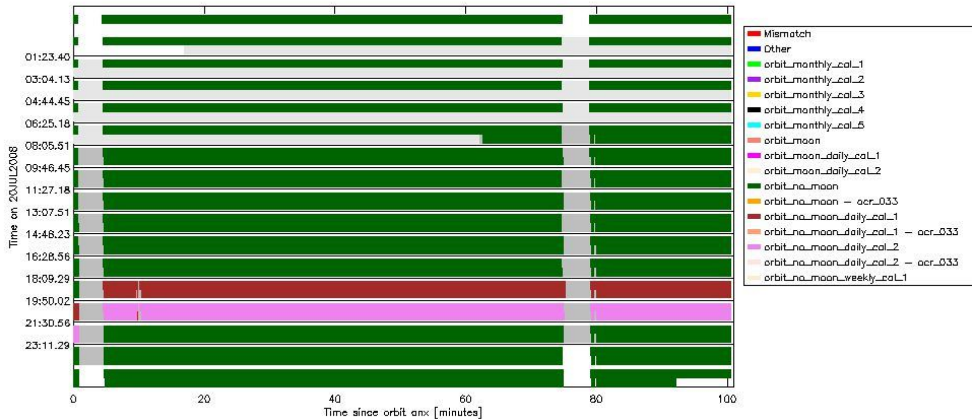
sciamachy_daily_report_level0_KSPT_L0_4303_N_20080720_6.PNG
