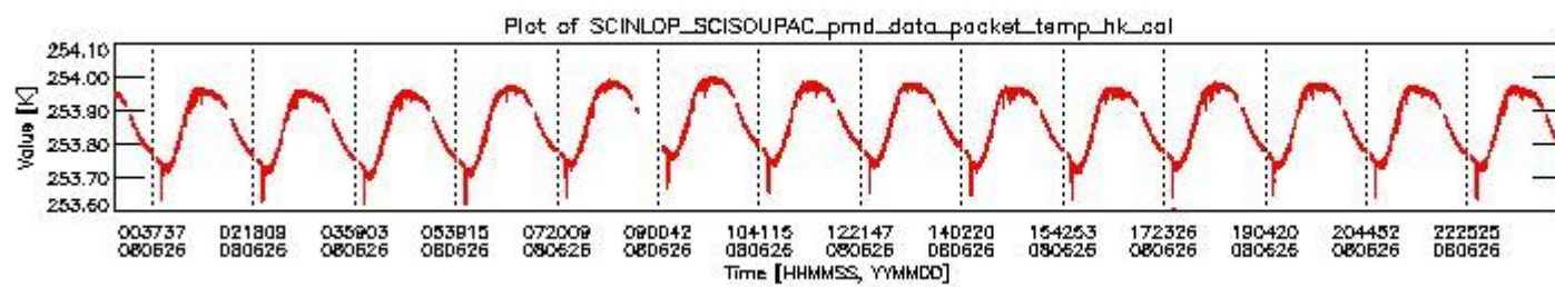
sciamachy_daily_report_level0_KSPT_L0_4303_N_20080626_3.PNG
