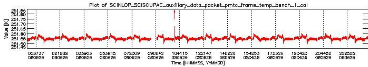
sciamachy_daily_report_level0_KSPT_L0_4303_N_20080626_0.PNG
