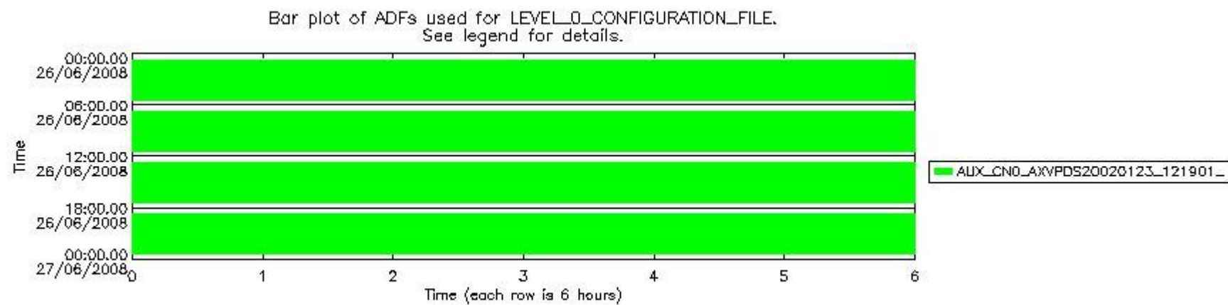
sciamachy_daily_report_level0_KSPT_L0_4303_N_20080626_7.PNG
