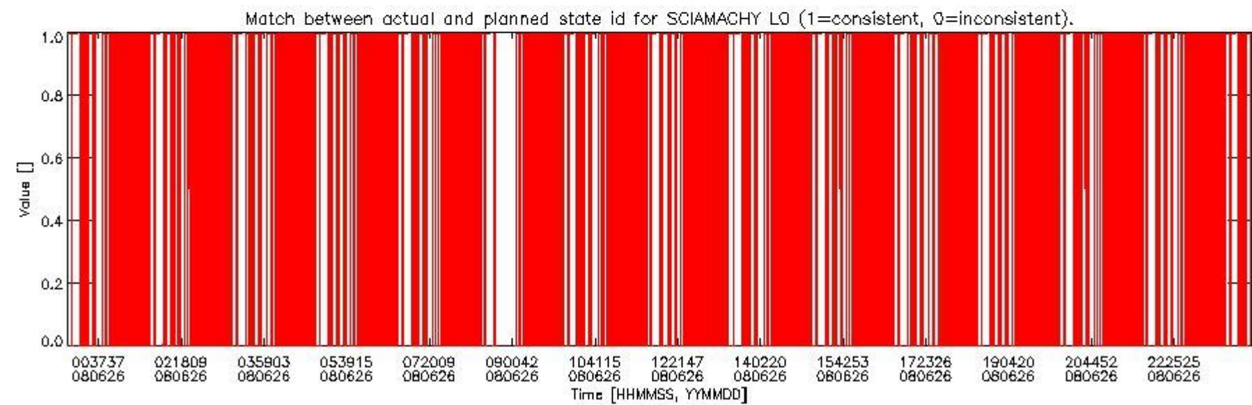
sciamachy_daily_report_level0_KSPT_L0_4303_N_20080626_5.PNG
