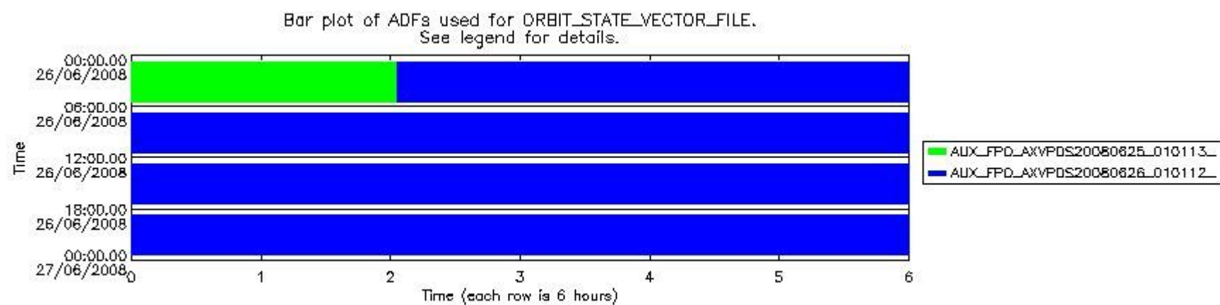
sciamachy_daily_report_level0_KSPT_L0_4303_N_20080626_8.PNG
