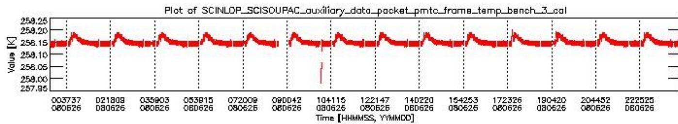
sciamachy_daily_report_level0_KSPT_L0_4303_N_20080626_2.PNG
