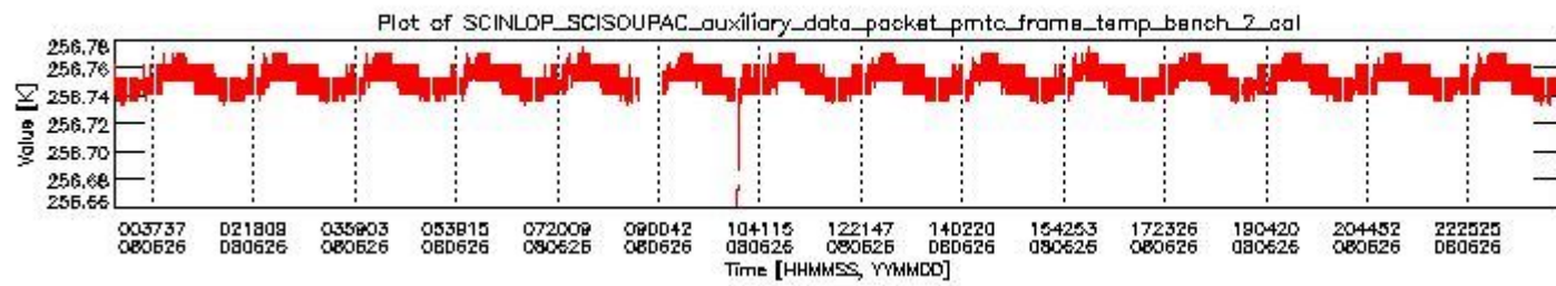
sciamachy_daily_report_level0_KSPT_L0_4303_N_20080626_1.PNG
