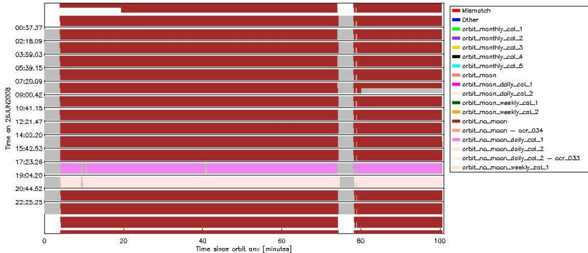
sciamachy_daily_report_level0_KSPT_L0_4303_N_20080626_6.PNG
