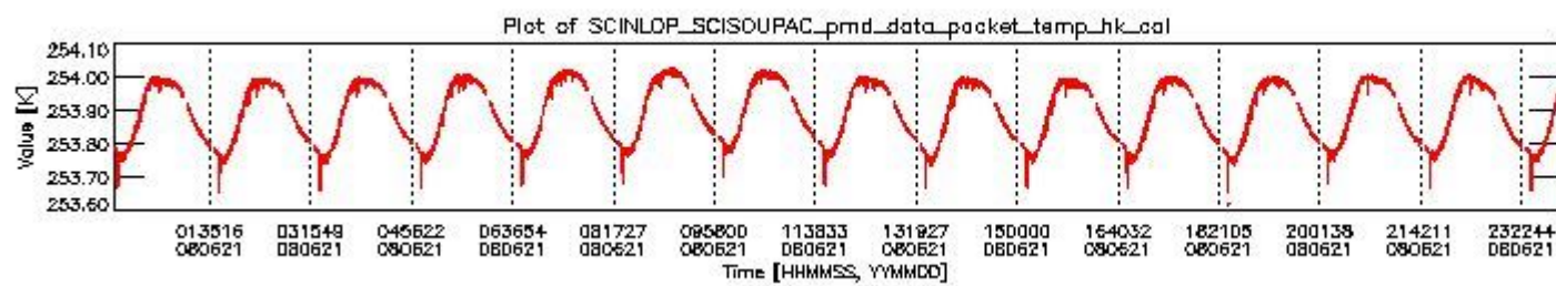
sciamachy_daily_report_level0_KSPT_L0_4303_N_20080621_3.PNG
