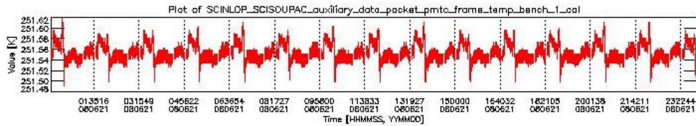
sciamachy_daily_report_level0_KSPT_L0_4303_N_20080621_0.PNG
