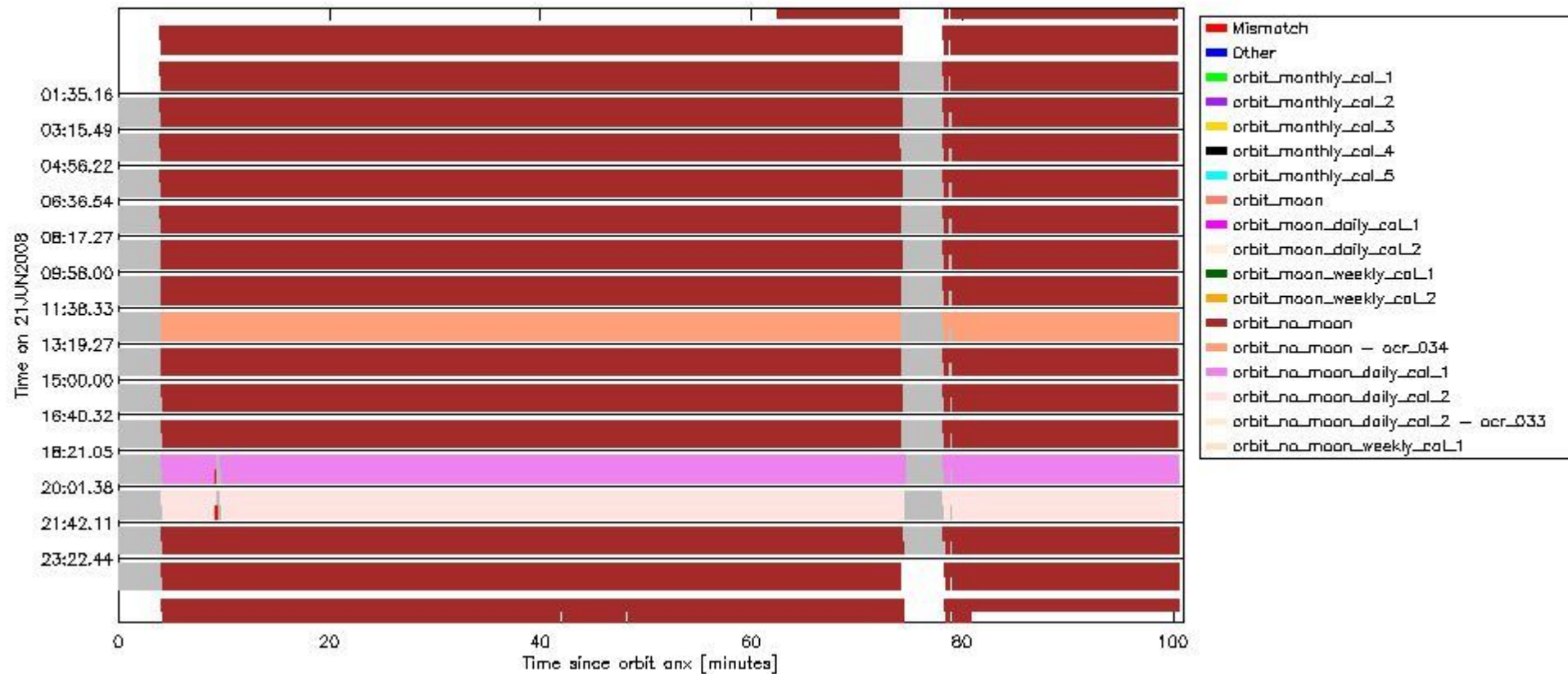
sciamachy_daily_report_level0_KSPT_L0_4303_N_20080621_6.PNG
