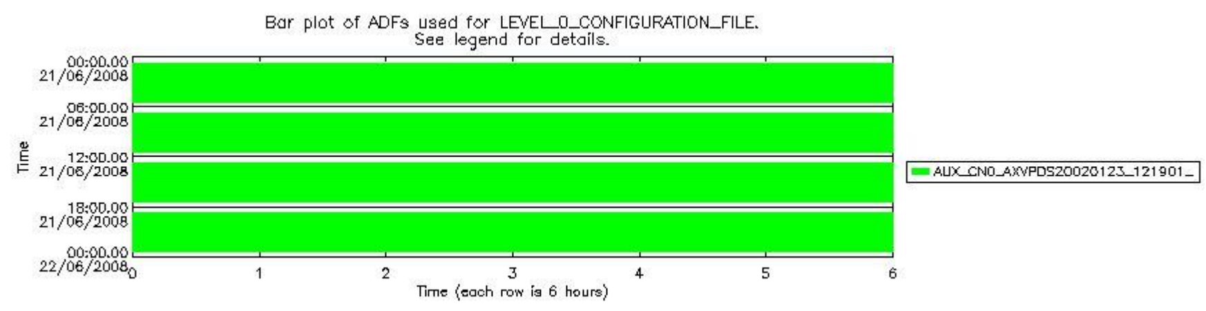
sciamachy_daily_report_level0_KSPT_L0_4303_N_20080621_7.PNG
