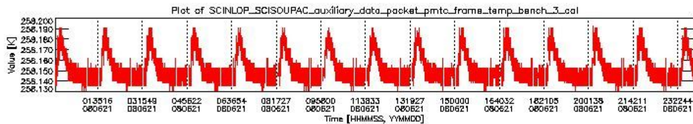
sciamachy_daily_report_level0_KSPT_L0_4303_N_20080621_2.PNG
