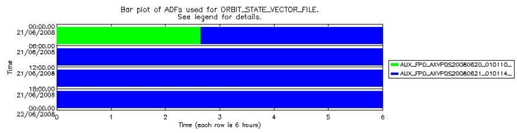
sciamachy_daily_report_level0_KSPT_L0_4303_N_20080621_8.PNG
