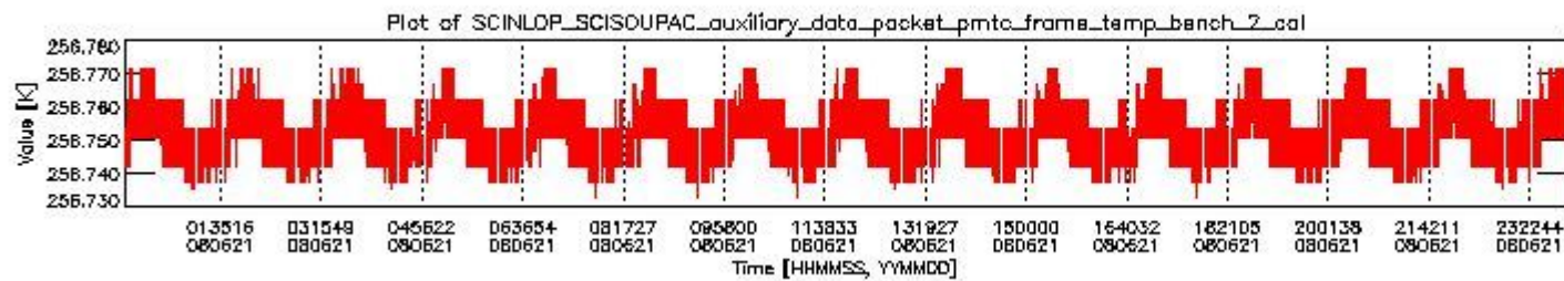
sciamachy_daily_report_level0_KSPT_L0_4303_N_20080621_1.PNG
