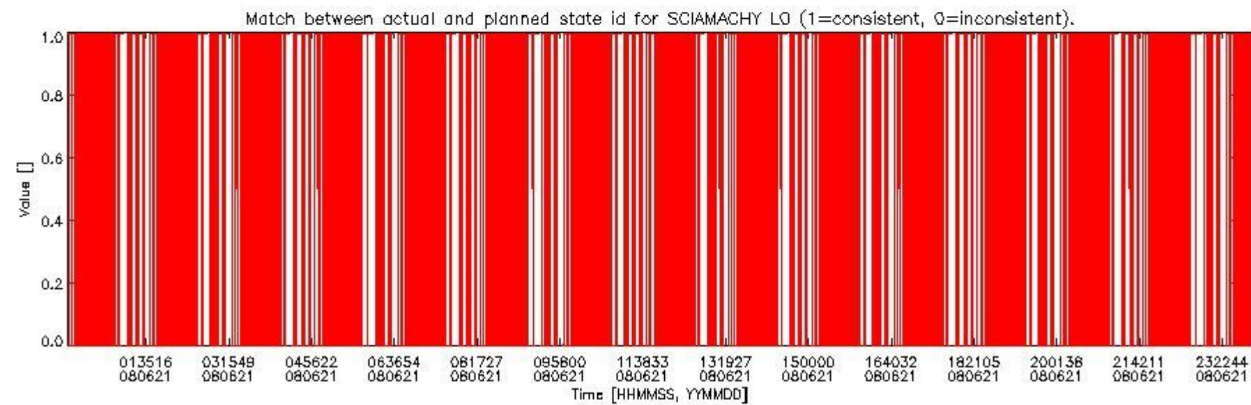
sciamachy_daily_report_level0_KSPT_L0_4303_N_20080621_5.PNG
