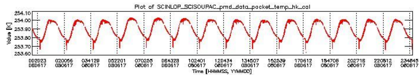
sciamachy_daily_report_level0_KSPT_L0_4303_N_20080617_3.PNG
