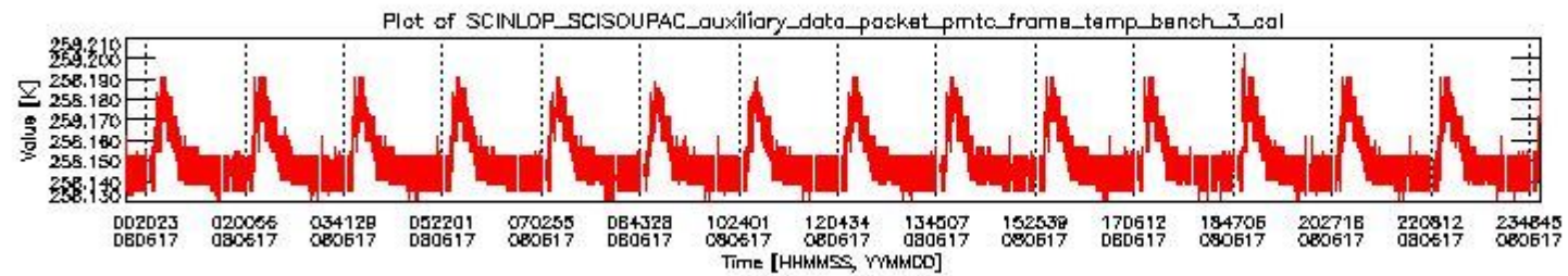
sciamachy_daily_report_level0_KSPT_L0_4303_N_20080617_2.PNG
