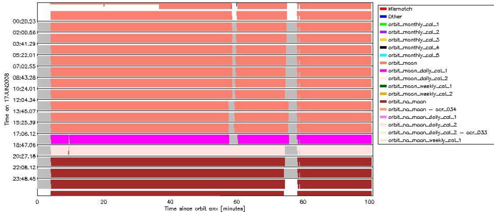
sciamachy_daily_report_level0_KSPT_L0_4303_N_20080617_6.PNG
