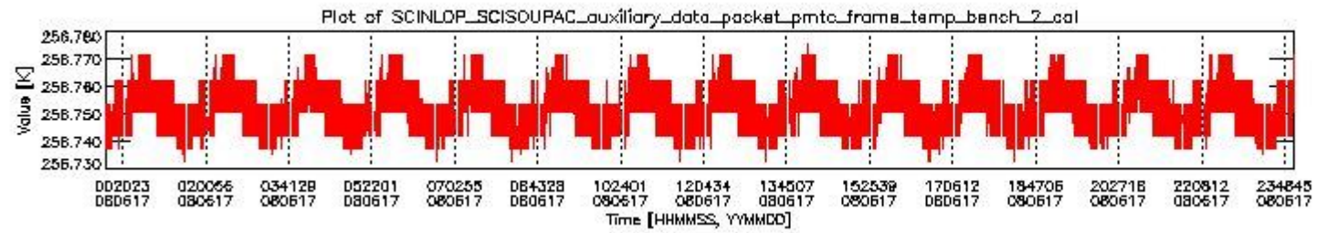
sciamachy_daily_report_level0_KSPT_L0_4303_N_20080617_1.PNG
