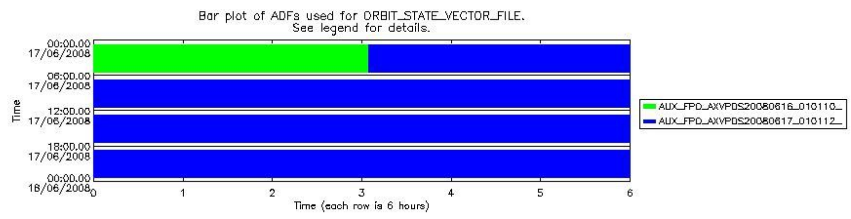
sciamachy_daily_report_level0_KSPT_L0_4303_N_20080617_8.PNG
