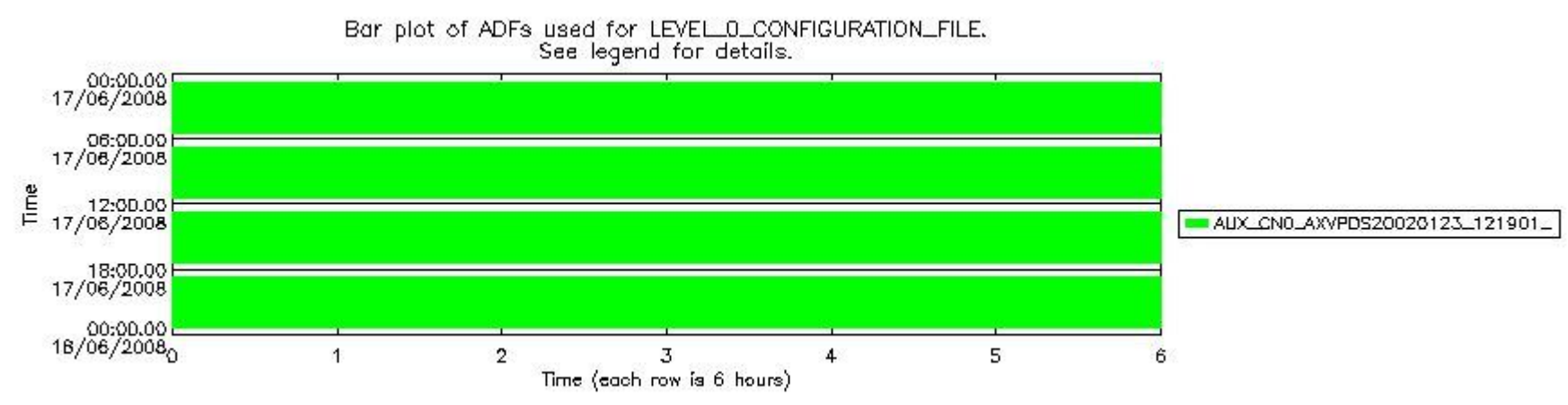
sciamachy_daily_report_level0_KSPT_L0_4303_N_20080617_7.PNG
