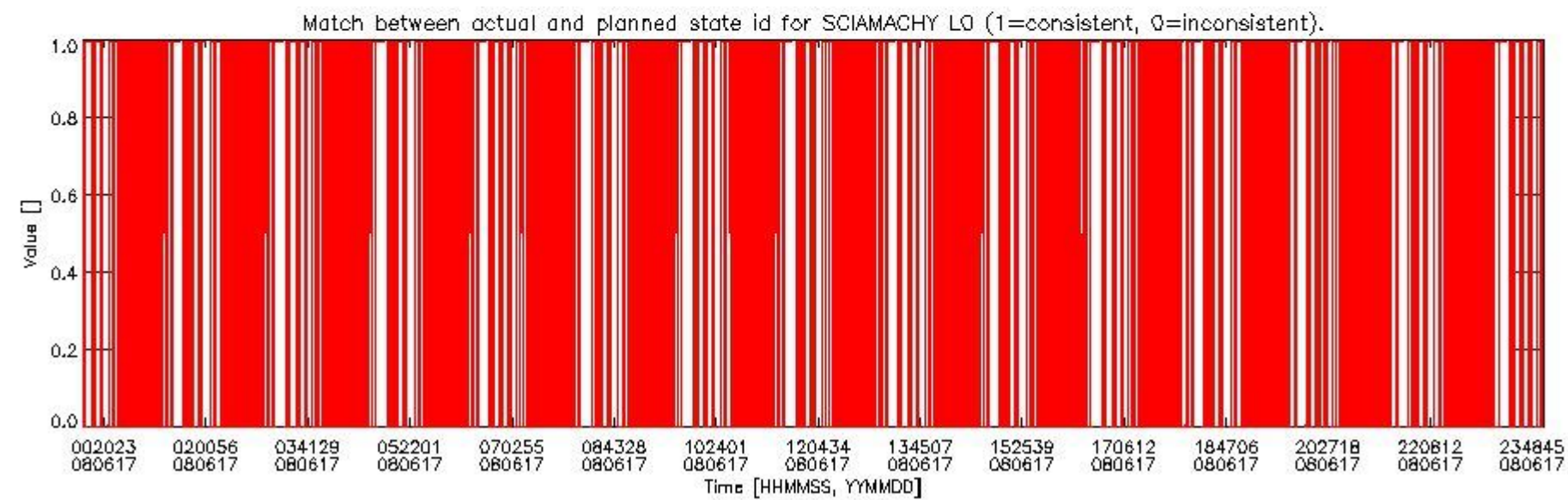
sciamachy_daily_report_level0_KSPT_L0_4303_N_20080617_5.PNG
