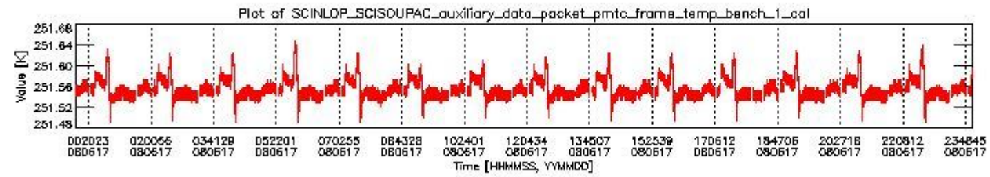
sciamachy_daily_report_level0_KSPT_L0_4303_N_20080617_0.PNG
