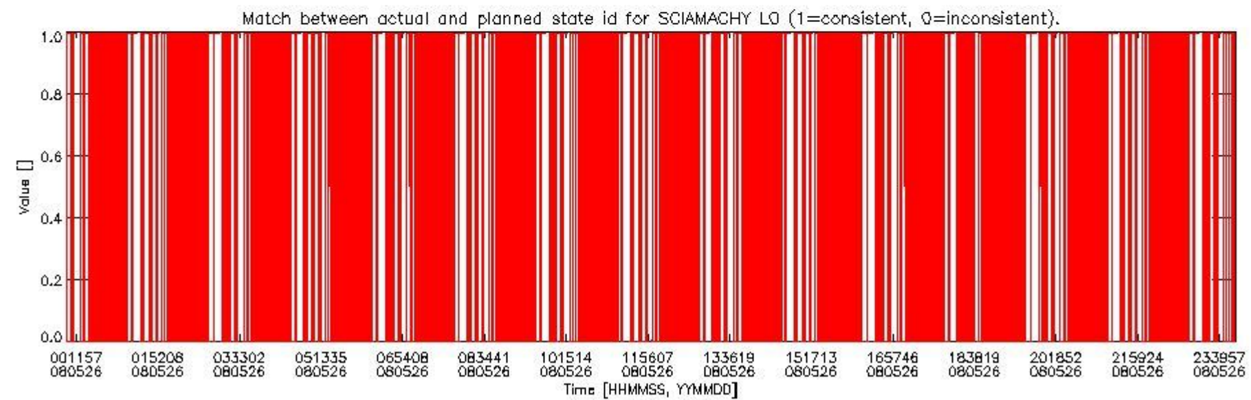
sciamachy_daily_report_level0_KSPT_L0_4303_N_20080526_5.PNG
