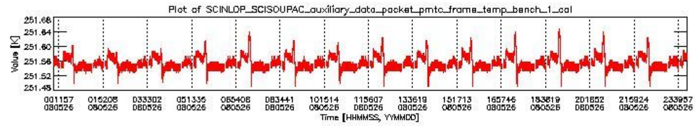
sciamachy_daily_report_level0_KSPT_L0_4303_N_20080526_0.PNG
