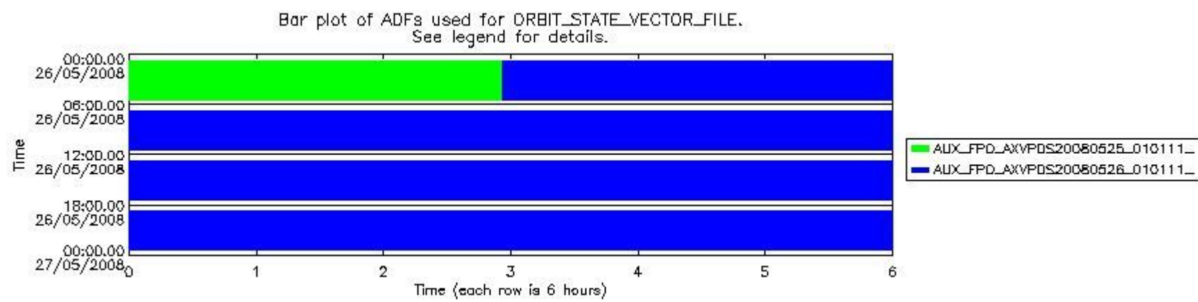
sciamachy_daily_report_level0_KSPT_L0_4303_N_20080526_8.PNG
