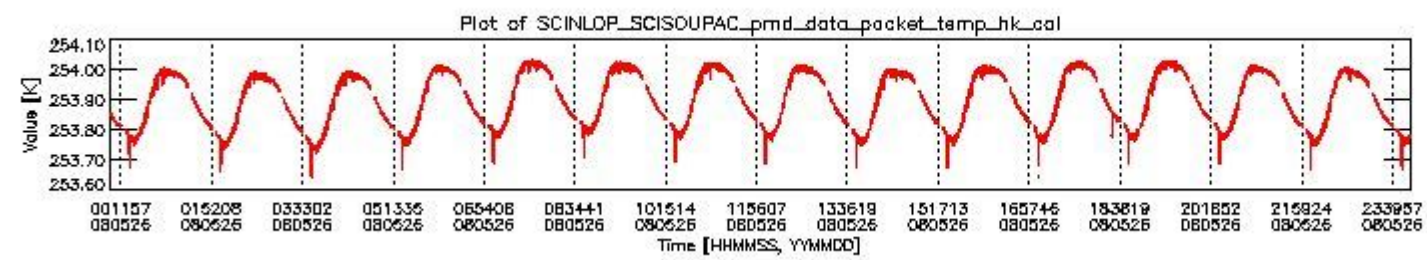
sciamachy_daily_report_level0_KSPT_L0_4303_N_20080526_3.PNG
