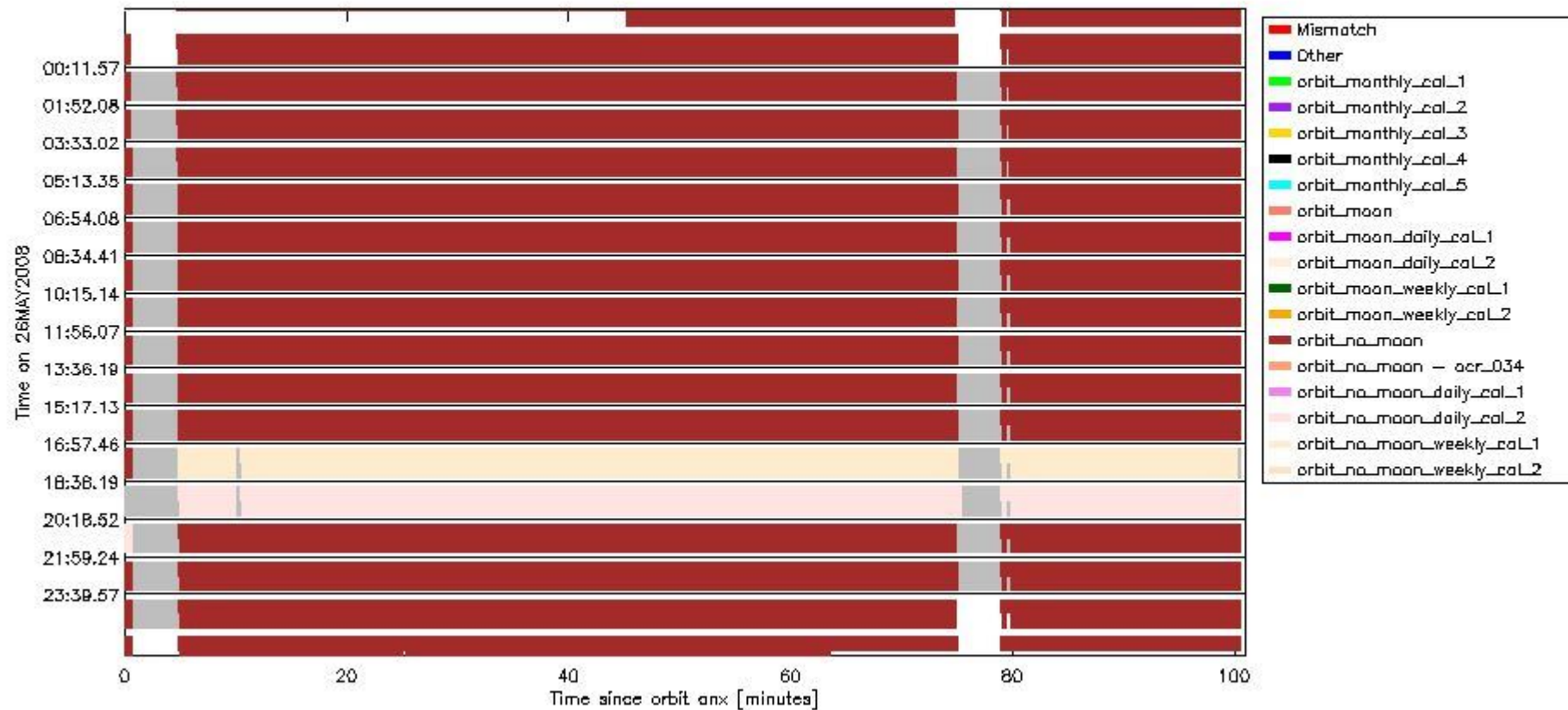
sciamachy_daily_report_level0_KSPT_L0_4303_N_20080526_6.PNG
