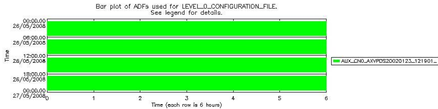
sciamachy_daily_report_level0_KSPT_L0_4303_N_20080526_7.PNG
