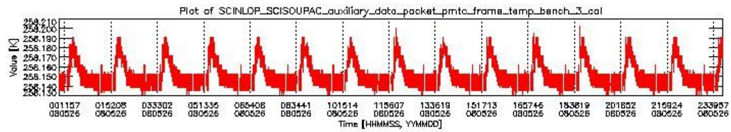
sciamachy_daily_report_level0_KSPT_L0_4303_N_20080526_2.PNG
