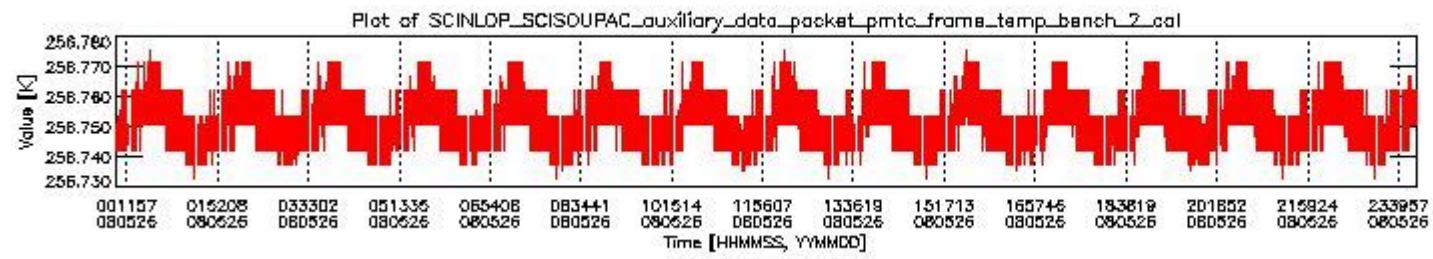
sciamachy_daily_report_level0_KSPT_L0_4303_N_20080526_1.PNG
