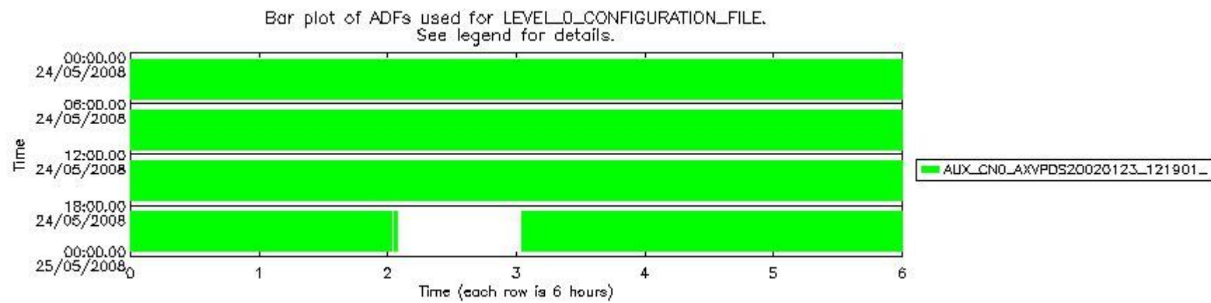
sciamachy_daily_report_level0_KSPT_L0_4303_N_20080524_7.PNG
