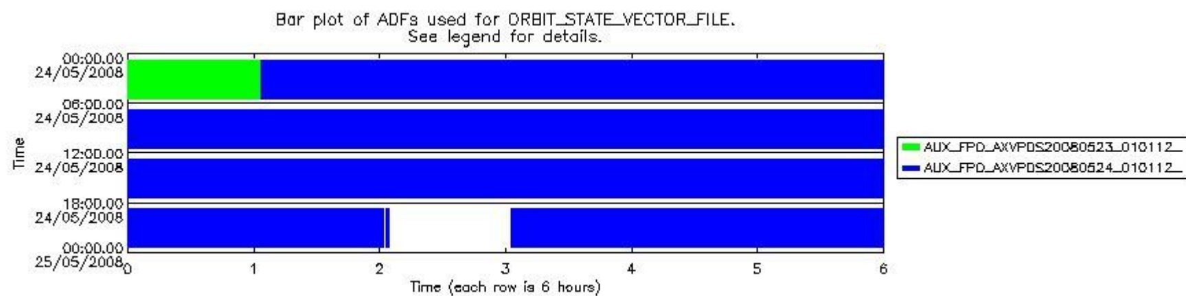
sciamachy_daily_report_level0_KSPT_L0_4303_N_20080524_8.PNG
