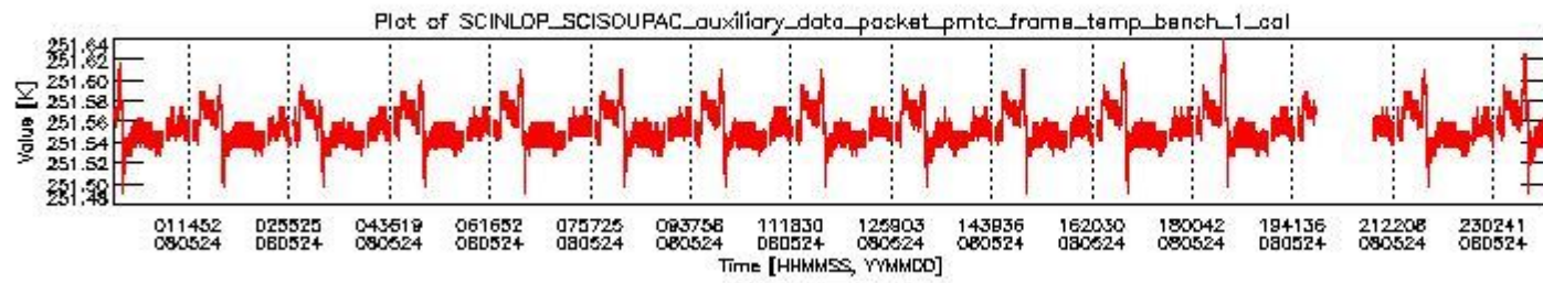
sciamachy_daily_report_level0_KSPT_L0_4303_N_20080524_0.PNG
