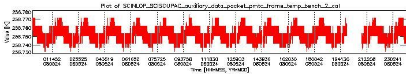
sciamachy_daily_report_level0_KSPT_L0_4303_N_20080524_1.PNG
