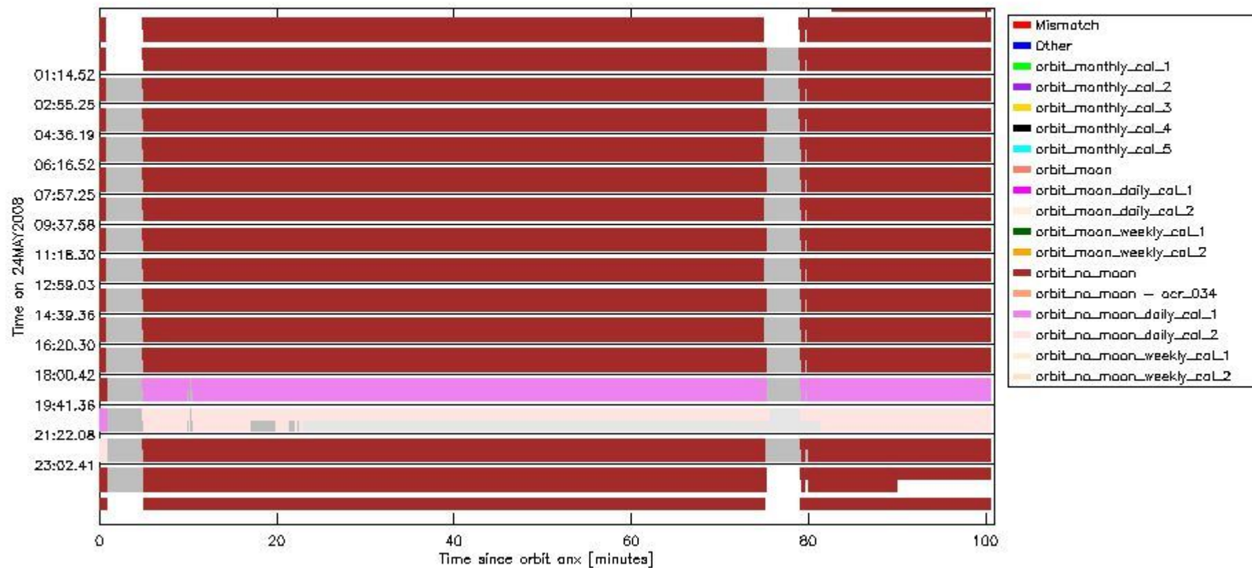
sciamachy_daily_report_level0_KSPT_L0_4303_N_20080524_6.PNG
