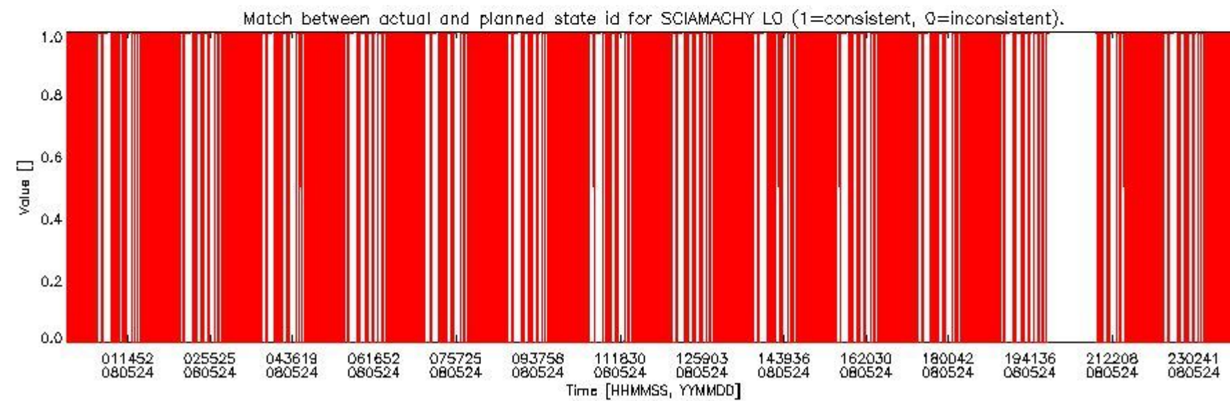
sciamachy_daily_report_level0_KSPT_L0_4303_N_20080524_5.PNG
