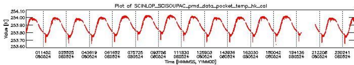
sciamachy_daily_report_level0_KSPT_L0_4303_N_20080524_3.PNG
