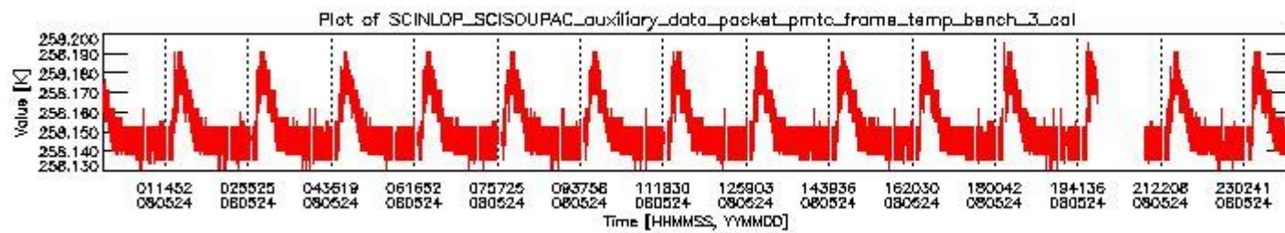
sciamachy_daily_report_level0_KSPT_L0_4303_N_20080524_2.PNG
