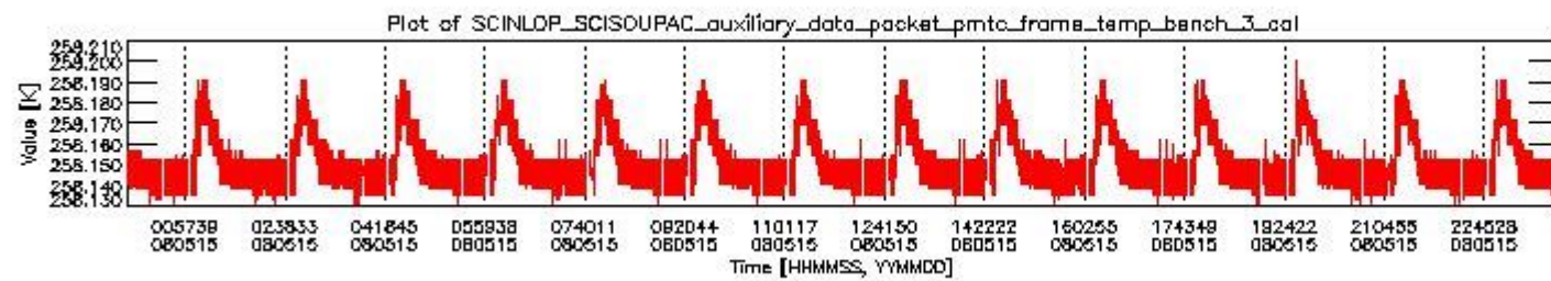
sciamachy_daily_report_level0_KSPT_L0_4303_N_20080515_2.PNG
