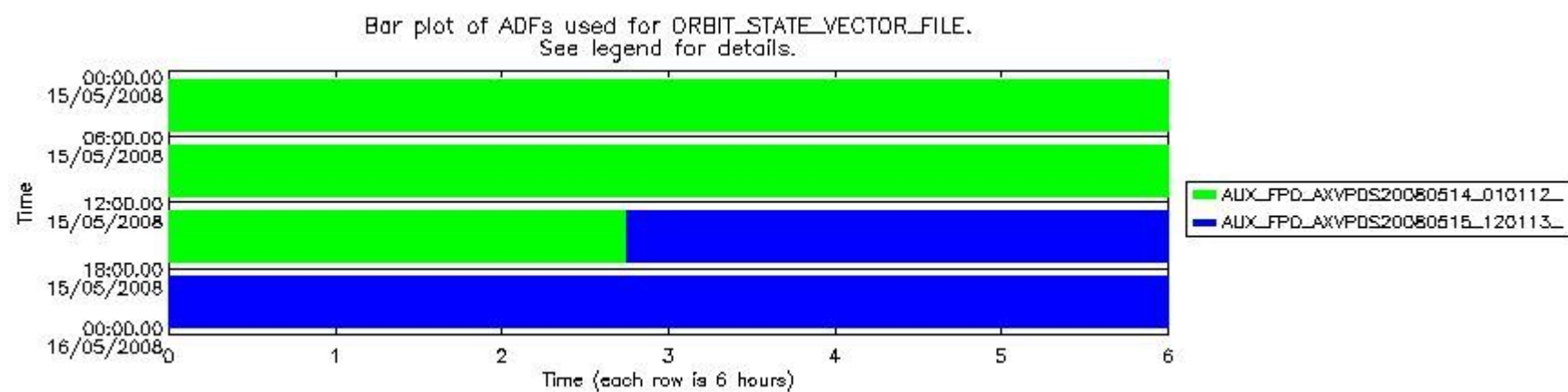
sciamachy_daily_report_level0_KSPT_L0_4303_N_20080515_8.PNG
