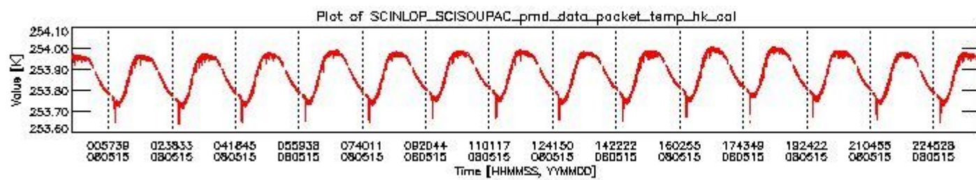
sciamachy_daily_report_level0_KSPT_L0_4303_N_20080515_3.PNG
