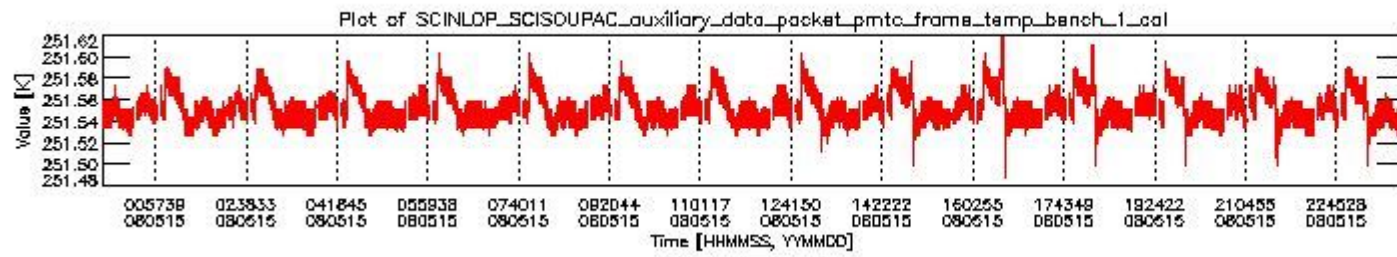
sciamachy_daily_report_level0_KSPT_L0_4303_N_20080515_0.PNG
