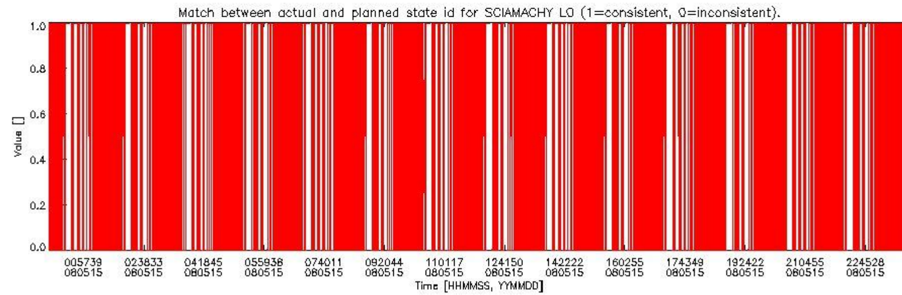
sciamachy_daily_report_level0_KSPT_L0_4303_N_20080515_5.PNG
