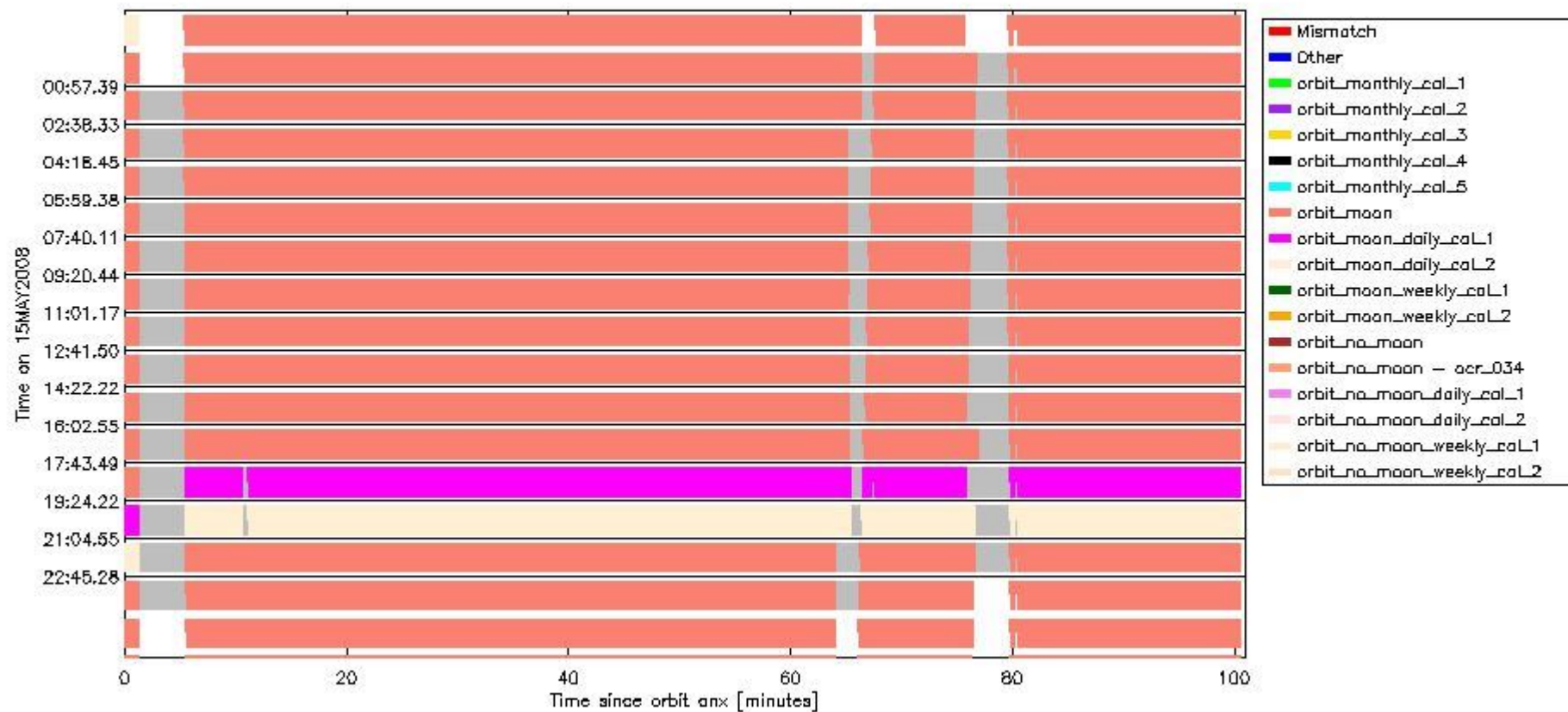
sciamachy_daily_report_level0_KSPT_L0_4303_N_20080515_6.PNG
