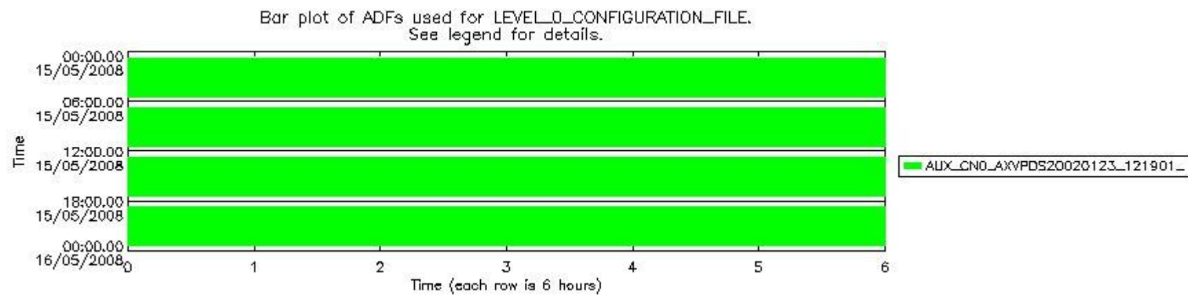
sciamachy_daily_report_level0_KSPT_L0_4303_N_20080515_7.PNG
