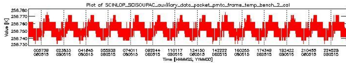
sciamachy_daily_report_level0_KSPT_L0_4303_N_20080515_1.PNG
