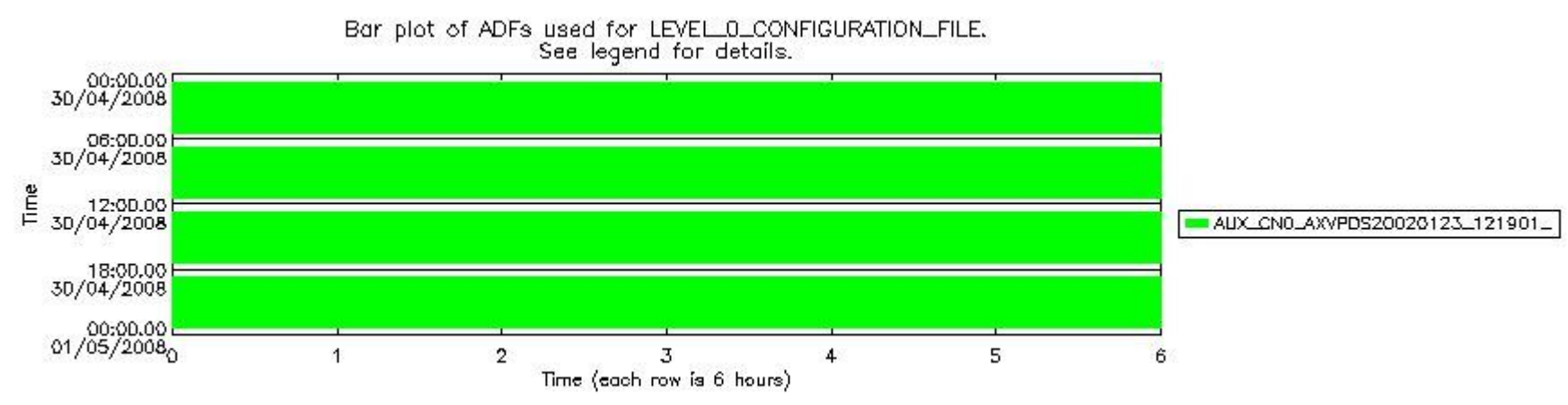
sciamachy_daily_report_level0_KSPT_L0_4303_N_20080430_7.PNG
