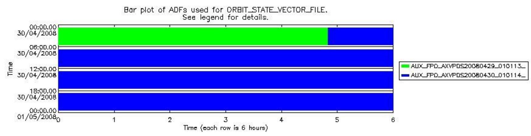
sciamachy_daily_report_level0_KSPT_L0_4303_N_20080430_8.PNG
