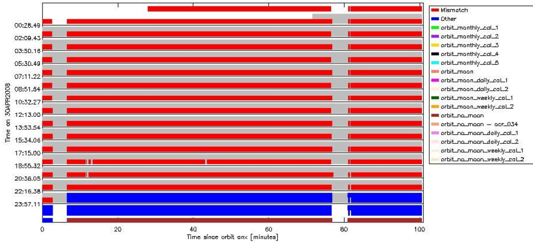
sciamachy_daily_report_level0_KSPT_L0_4303_N_20080430_6.PNG
