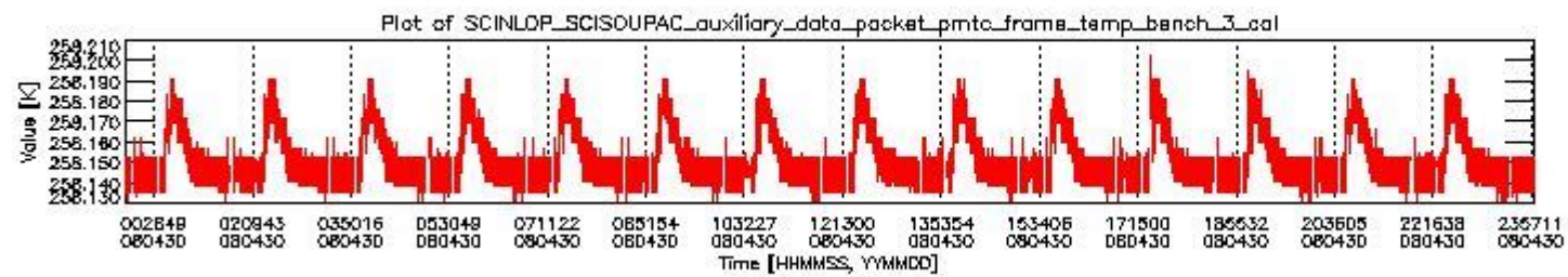
sciamachy_daily_report_level0_KSPT_L0_4303_N_20080430_2.PNG
