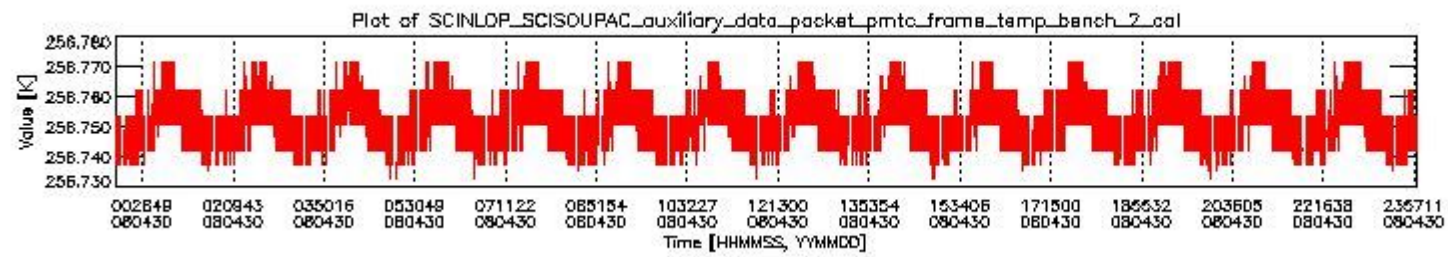
sciamachy_daily_report_level0_KSPT_L0_4303_N_20080430_1.PNG
