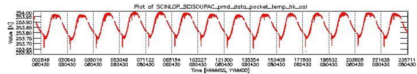
sciamachy_daily_report_level0_KSPT_L0_4303_N_20080430_3.PNG
