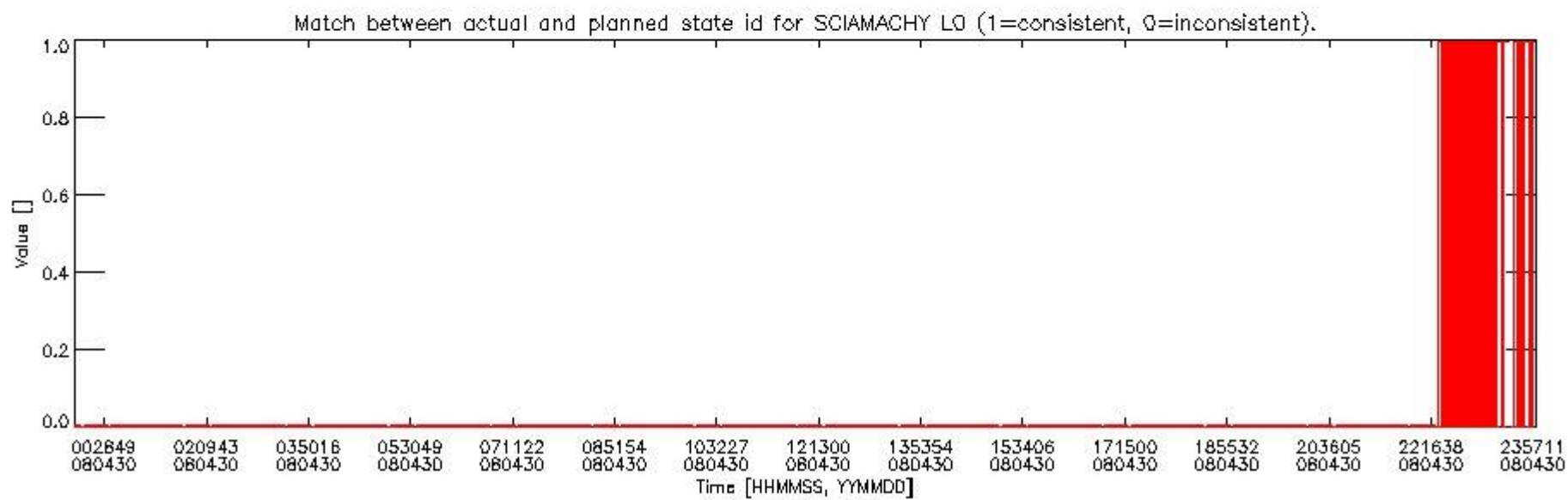
sciamachy_daily_report_level0_KSPT_L0_4303_N_20080430_5.PNG
