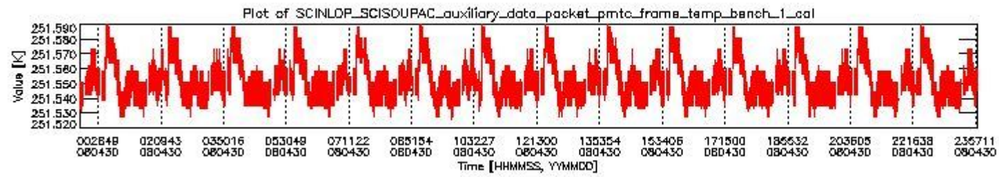
sciamachy_daily_report_level0_KSPT_L0_4303_N_20080430_0.PNG
