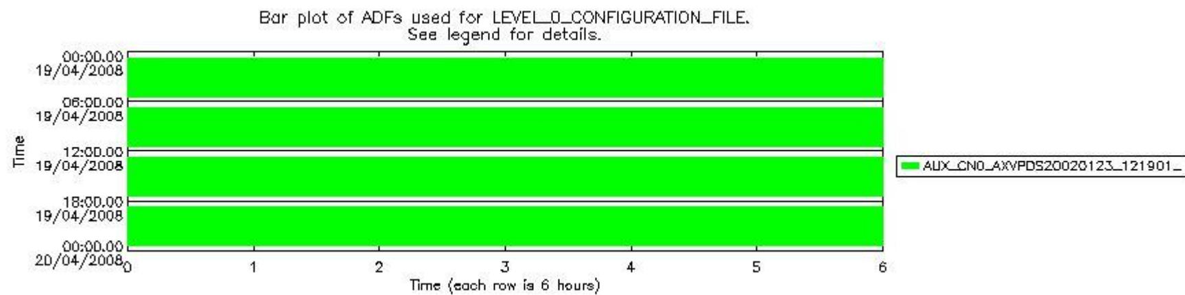
sciamachy_daily_report_level0_KSPT_L0_4303_N_20080419_7.PNG
