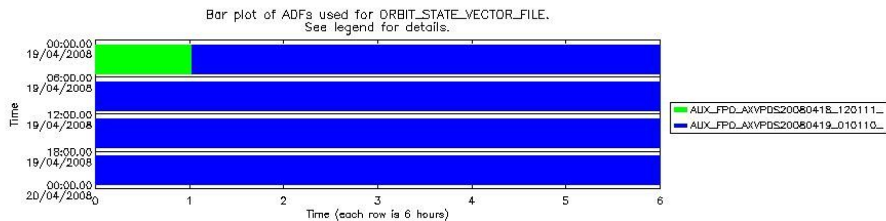
sciamachy_daily_report_level0_KSPT_L0_4303_N_20080419_8.PNG
