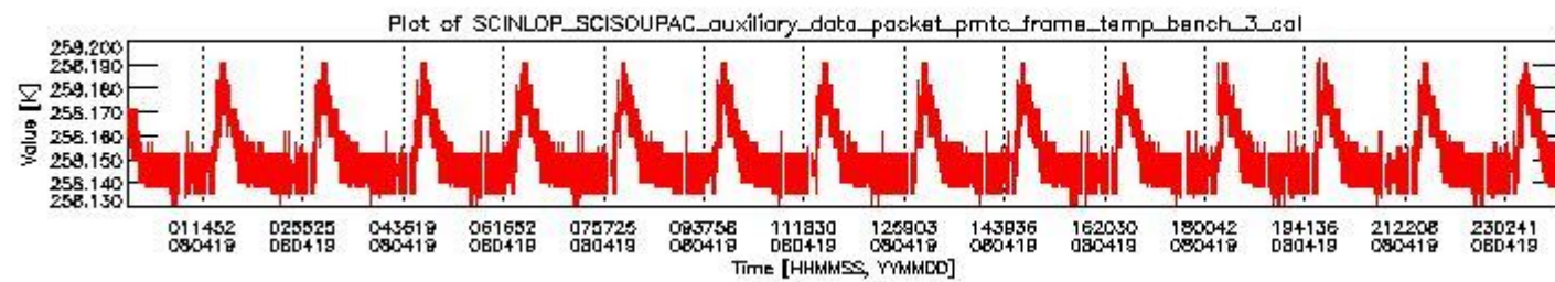
sciamachy_daily_report_level0_KSPT_L0_4303_N_20080419_2.PNG
