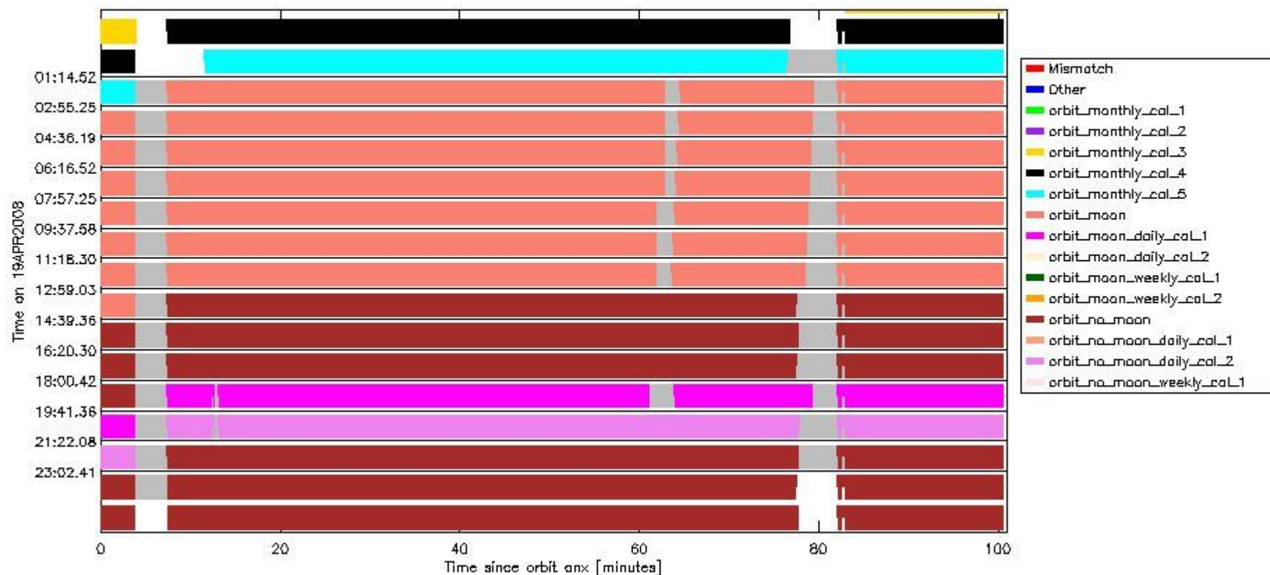
sciamachy_daily_report_level0_KSPT_L0_4303_N_20080419_6.PNG
