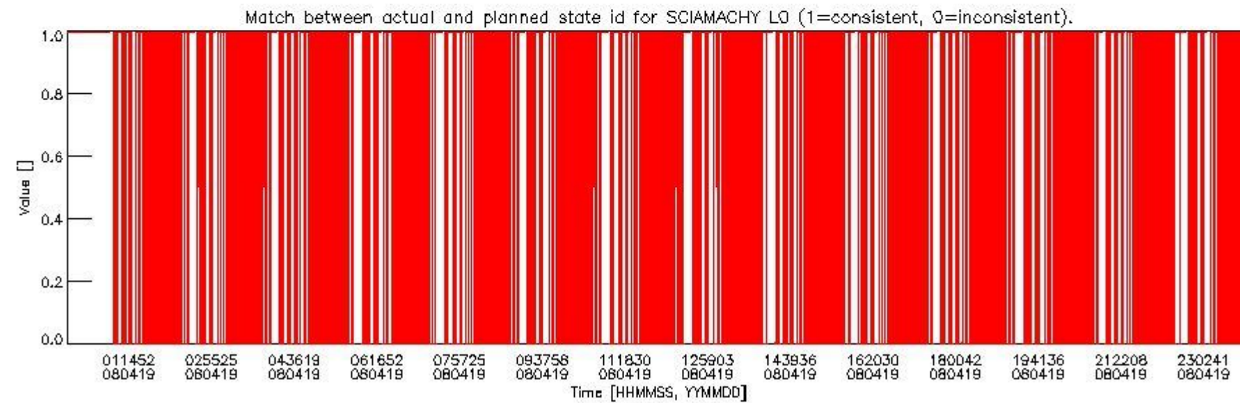
sciamachy_daily_report_level0_KSPT_L0_4303_N_20080419_5.PNG
