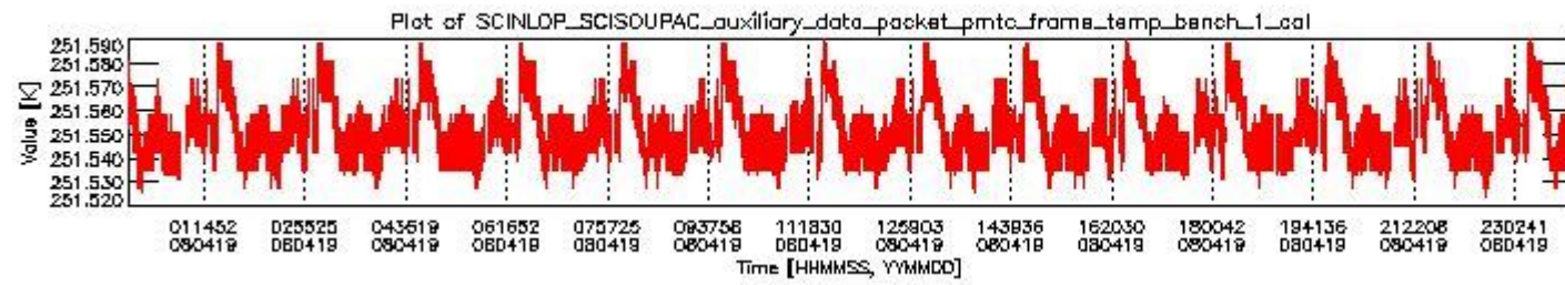
sciamachy_daily_report_level0_KSPT_L0_4303_N_20080419_0.PNG
