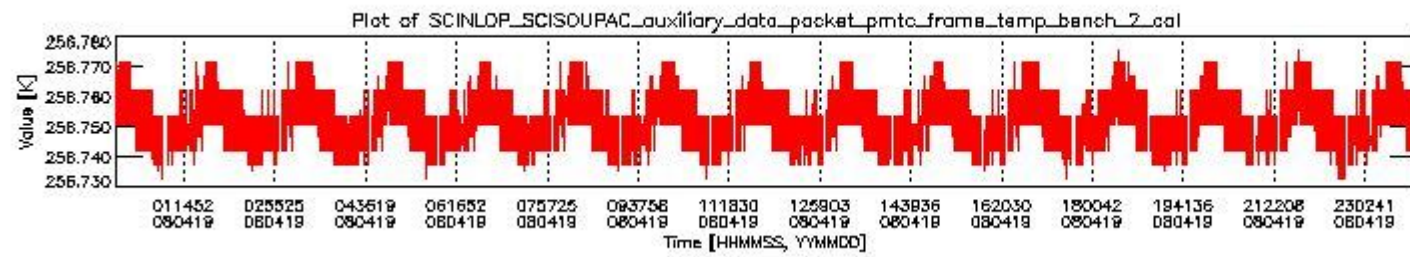
sciamachy_daily_report_level0_KSPT_L0_4303_N_20080419_1.PNG
