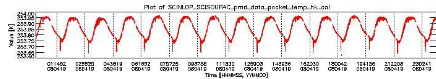
sciamachy_daily_report_level0_KSPT_L0_4303_N_20080419_3.PNG
