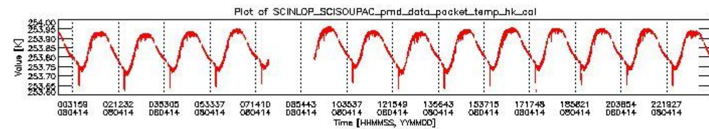
sciamachy_daily_report_level0_KSPT_L0_4303_N_20080414_3.PNG
