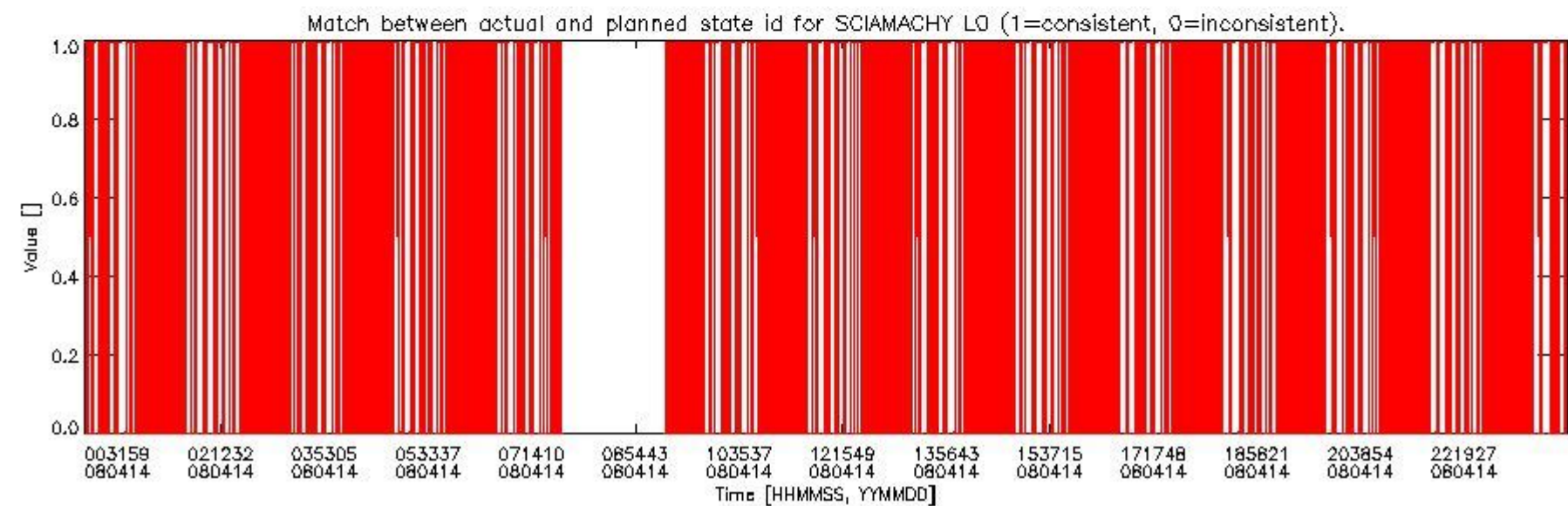
sciamachy_daily_report_level0_KSPT_L0_4303_N_20080414_5.PNG
