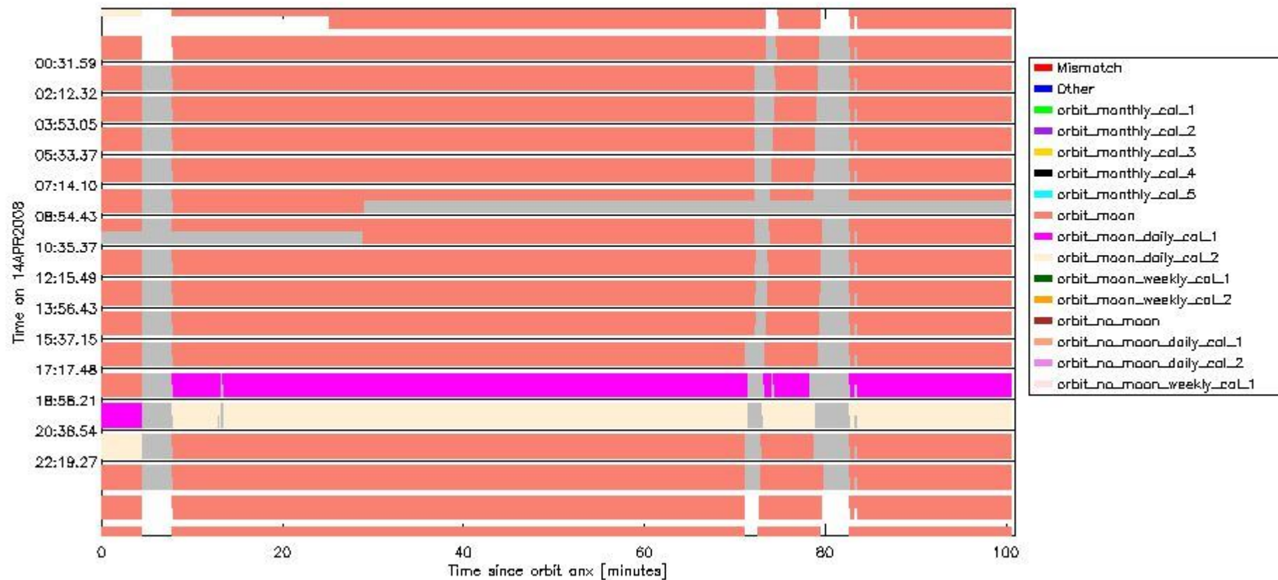
sciamachy_daily_report_level0_KSPT_L0_4303_N_20080414_6.PNG
