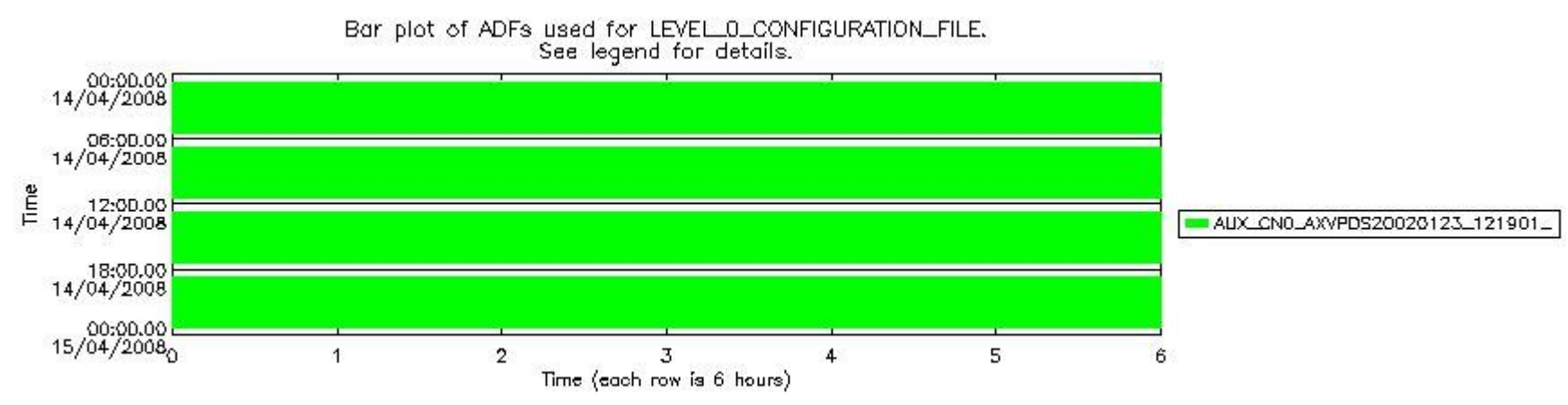
sciamachy_daily_report_level0_KSPT_L0_4303_N_20080414_7.PNG
