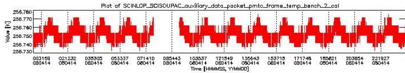
sciamachy_daily_report_level0_KSPT_L0_4303_N_20080414_1.PNG
