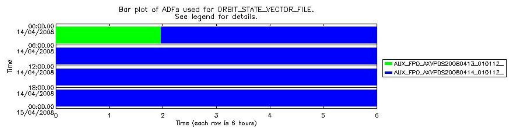
sciamachy_daily_report_level0_KSPT_L0_4303_N_20080414_8.PNG
