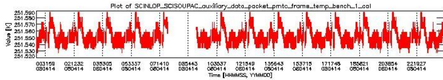
sciamachy_daily_report_level0_KSPT_L0_4303_N_20080414_0.PNG
