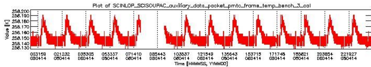
sciamachy_daily_report_level0_KSPT_L0_4303_N_20080414_2.PNG
