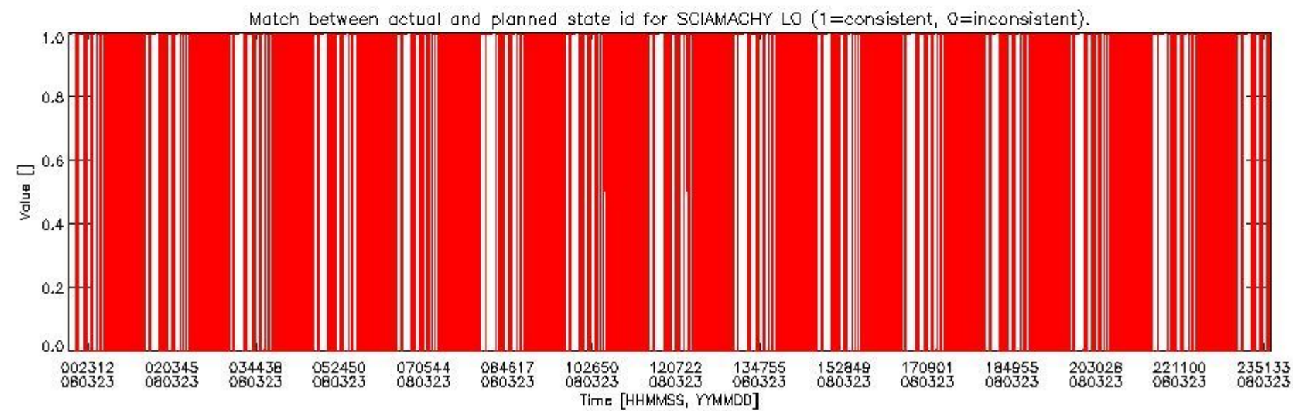
sciamachy_daily_report_level0_KSPT_L0_4303_N_20080323_5.PNG
