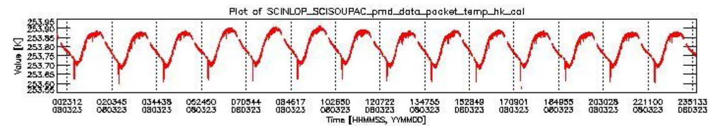
sciamachy_daily_report_level0_KSPT_L0_4303_N_20080323_3.PNG
