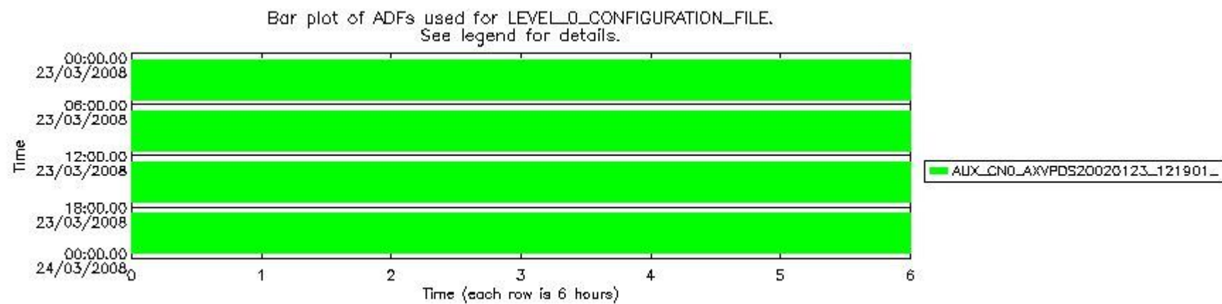
sciamachy_daily_report_level0_KSPT_L0_4303_N_20080323_7.PNG
