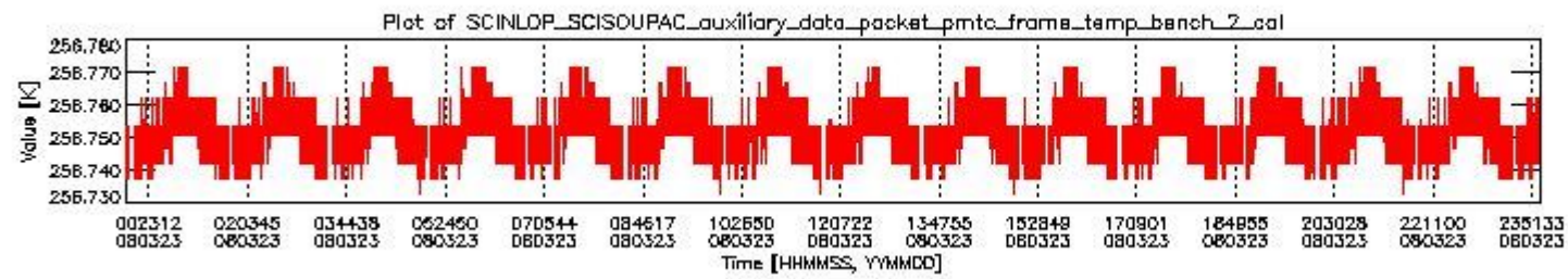
sciamachy_daily_report_level0_KSPT_L0_4303_N_20080323_1.PNG
