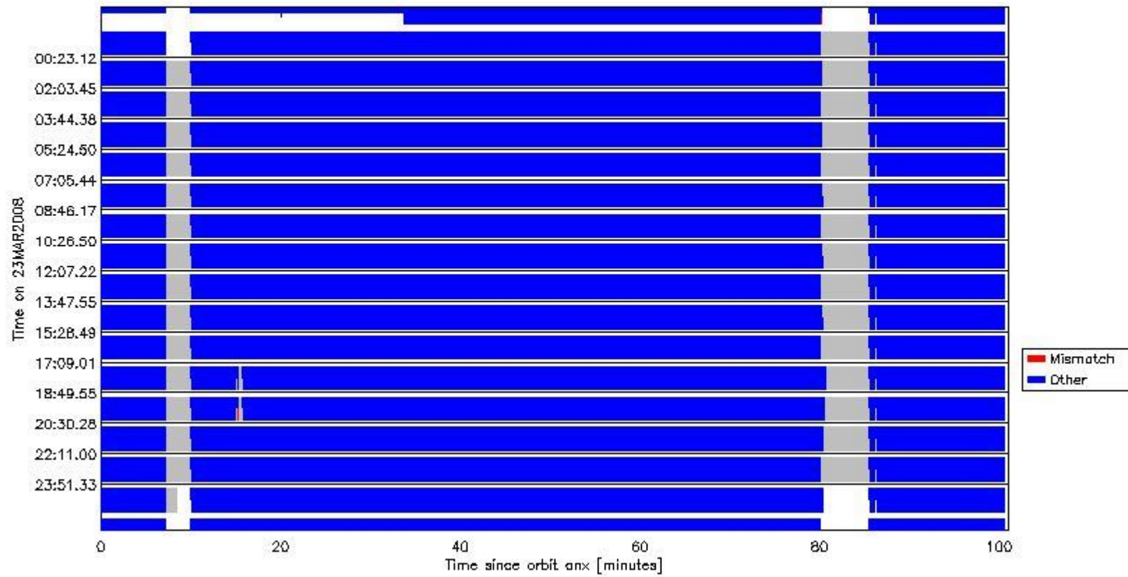
sciamachy_daily_report_level0_KSPT_L0_4303_N_20080323_6.PNG
