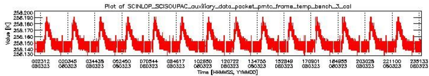
sciamachy_daily_report_level0_KSPT_L0_4303_N_20080323_2.PNG
