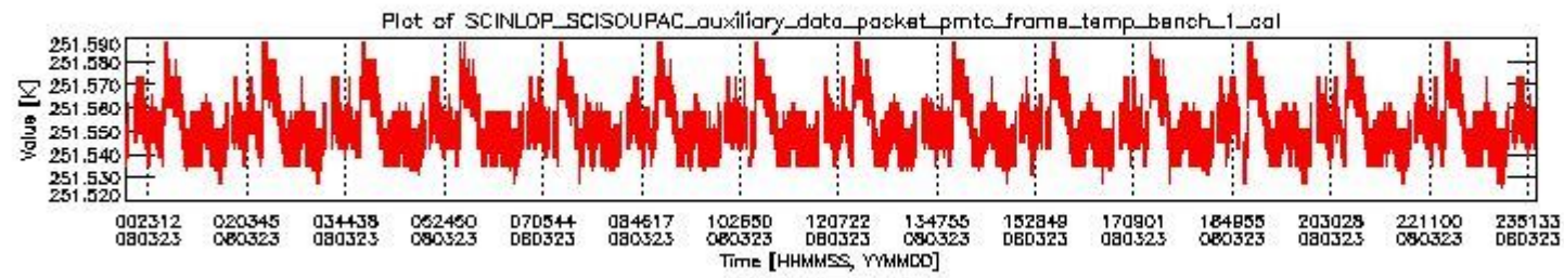
sciamachy_daily_report_level0_KSPT_L0_4303_N_20080323_0.PNG
