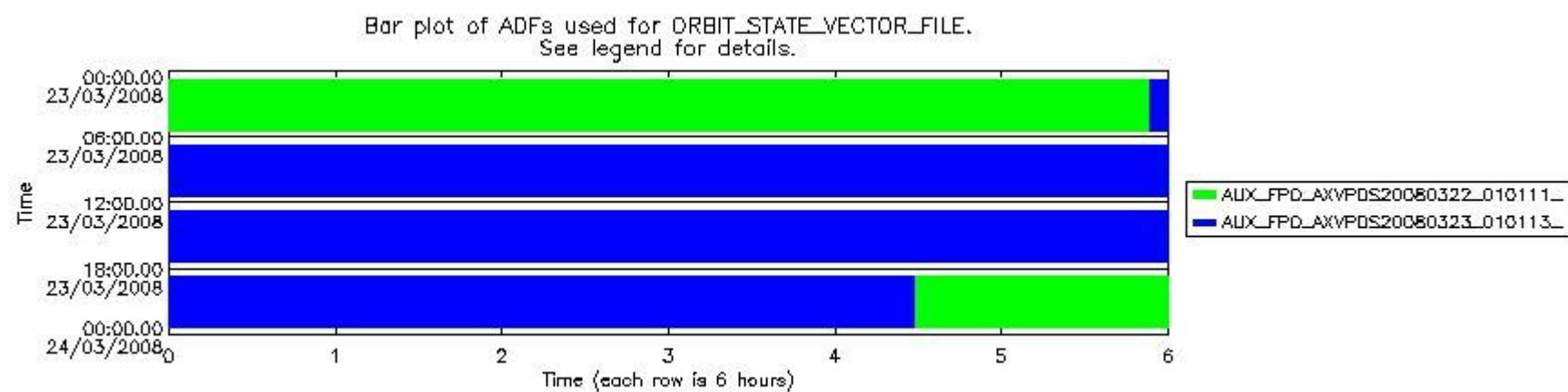
sciamachy_daily_report_level0_KSPT_L0_4303_N_20080323_8.PNG
