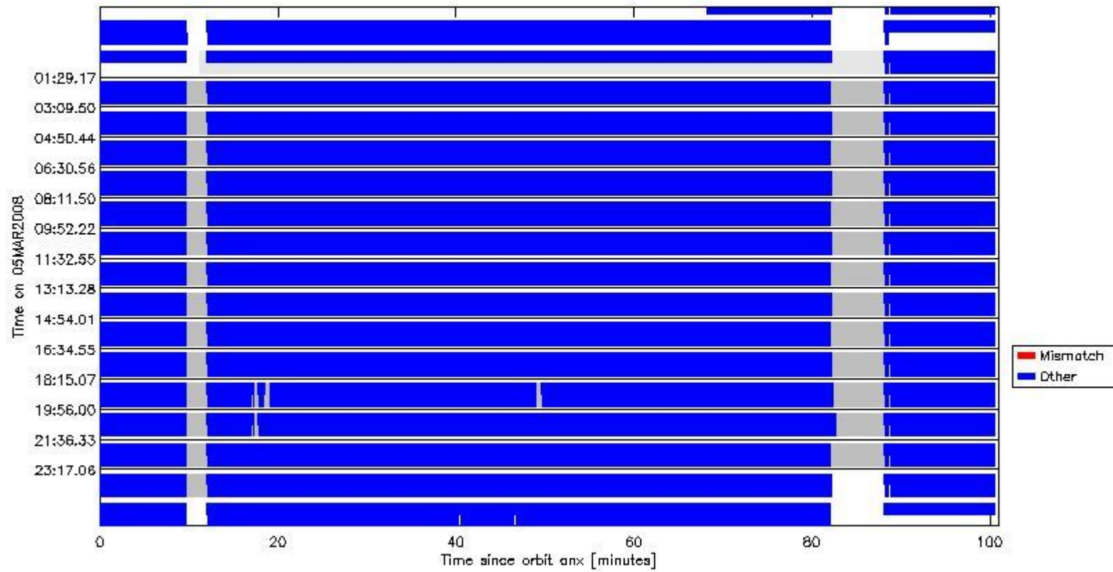
sciamachy_daily_report_level0_KSPT_L0_4303_N_20080305_6.PNG
