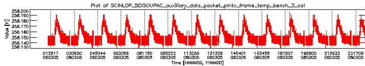
sciamachy_daily_report_level0_KSPT_L0_4303_N_20080305_2.PNG
