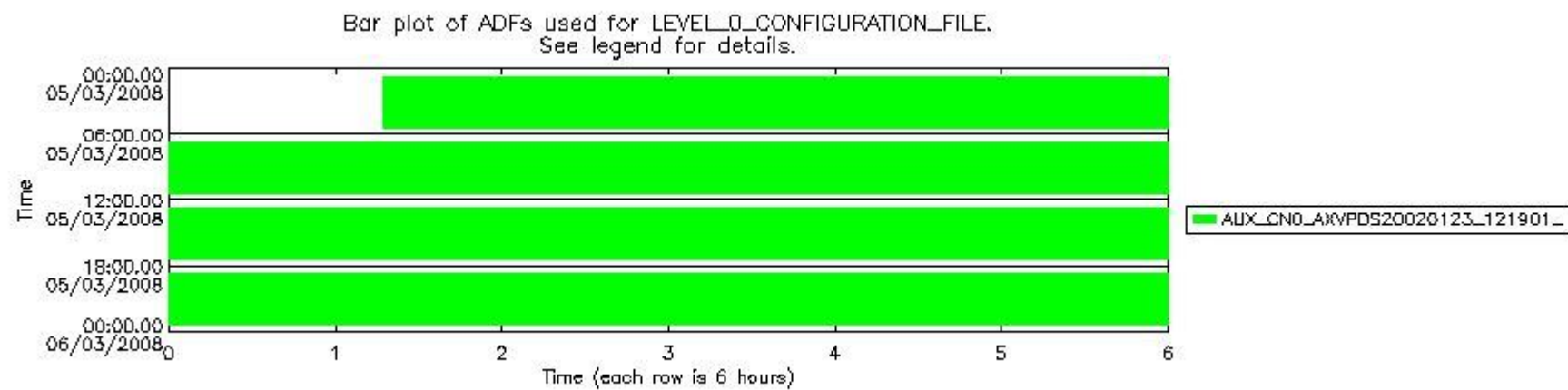
sciamachy_daily_report_level0_KSPT_L0_4303_N_20080305_7.PNG
