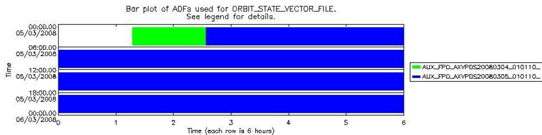
sciamachy_daily_report_level0_KSPT_L0_4303_N_20080305_8.PNG
