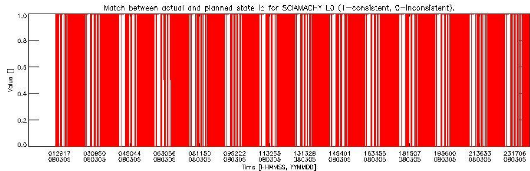
sciamachy_daily_report_level0_KSPT_L0_4303_N_20080305_5.PNG
