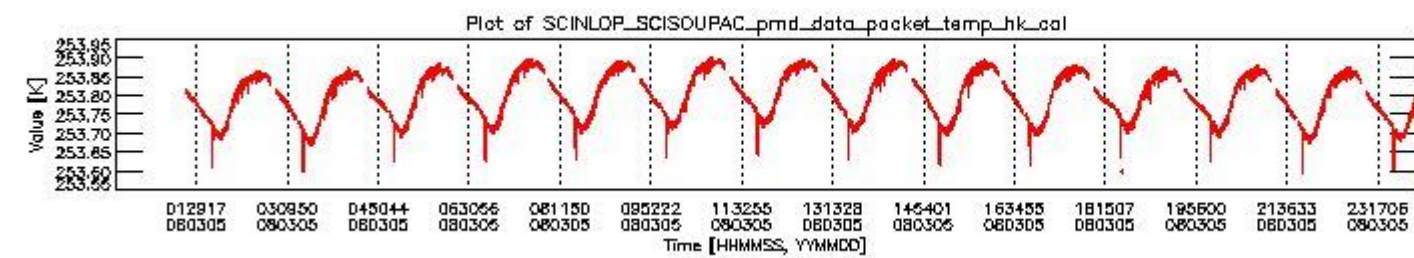
sciamachy_daily_report_level0_KSPT_L0_4303_N_20080305_3.PNG
