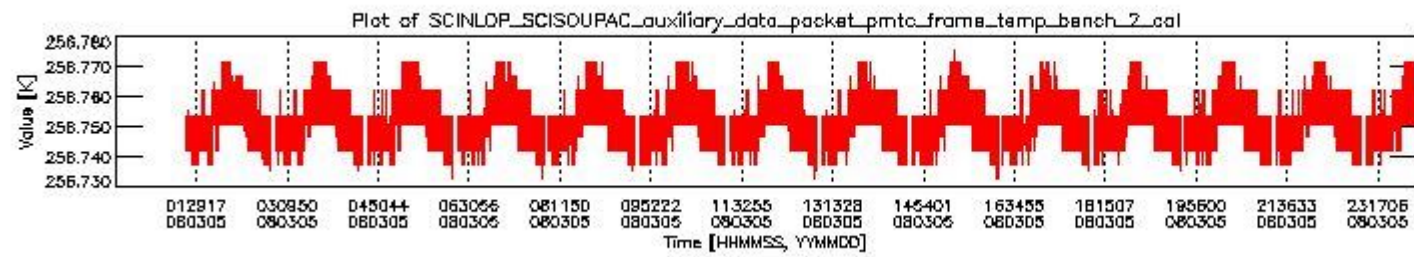
sciamachy_daily_report_level0_KSPT_L0_4303_N_20080305_1.PNG
