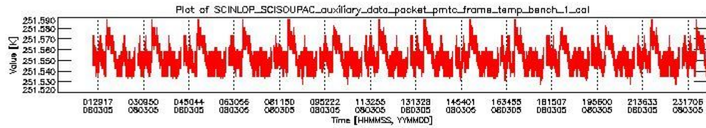
sciamachy_daily_report_level0_KSPT_L0_4303_N_20080305_0.PNG
